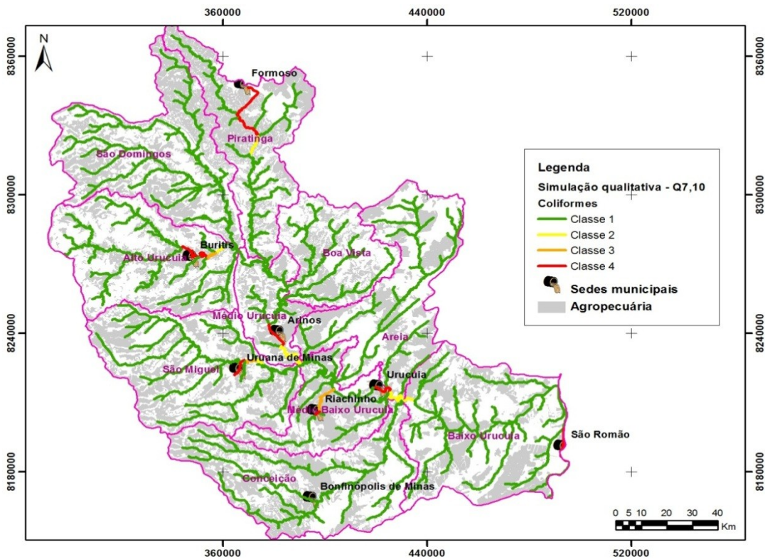
Figura 7.29 - Simulação qualitativa SF8 - Q 7,10 / Coliformes.
