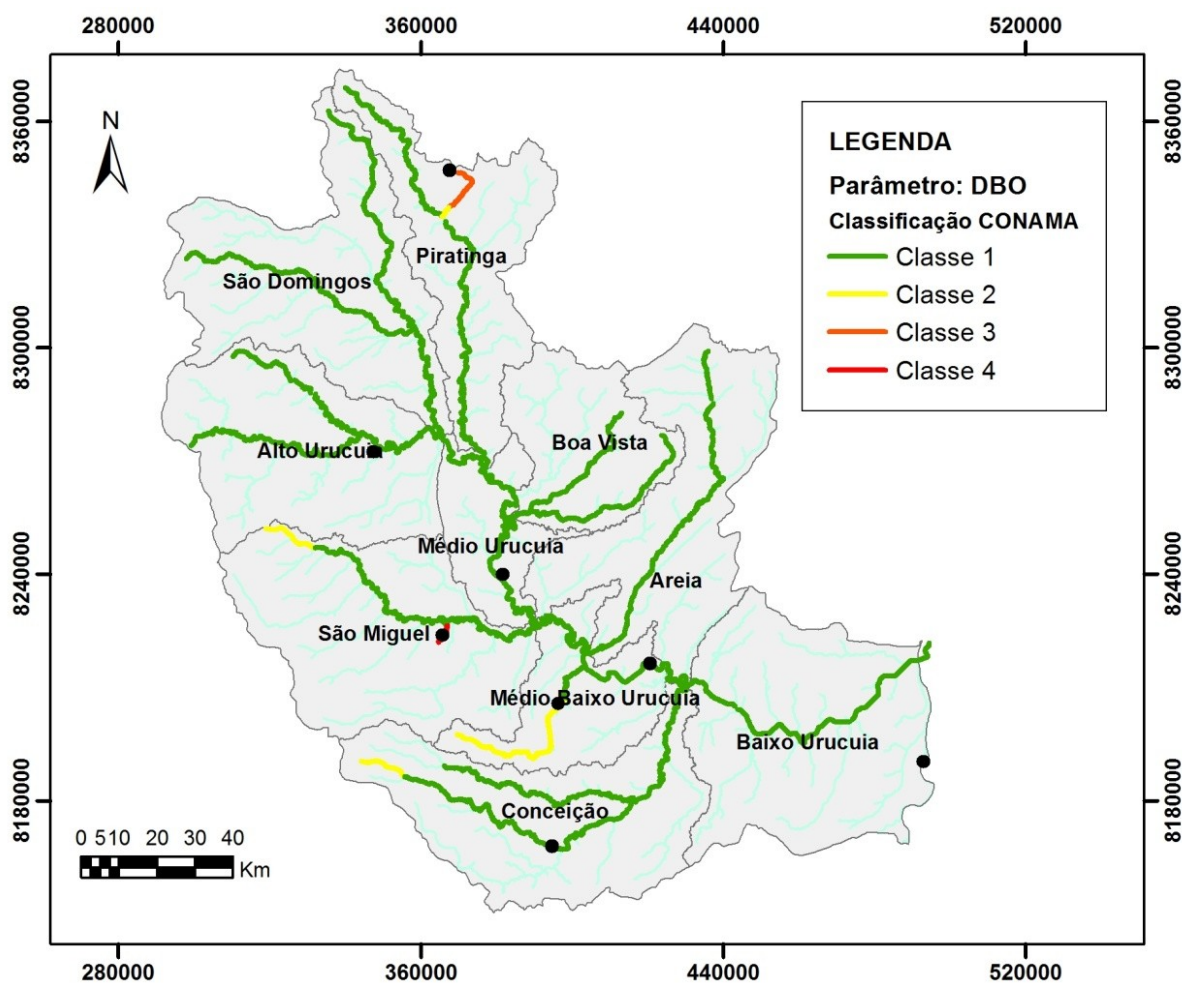
Figura 7.43 - Simulação da concentração de DBO na bacia SF8, considerando um cenário de vazão correspondente à Q_{mld} .
