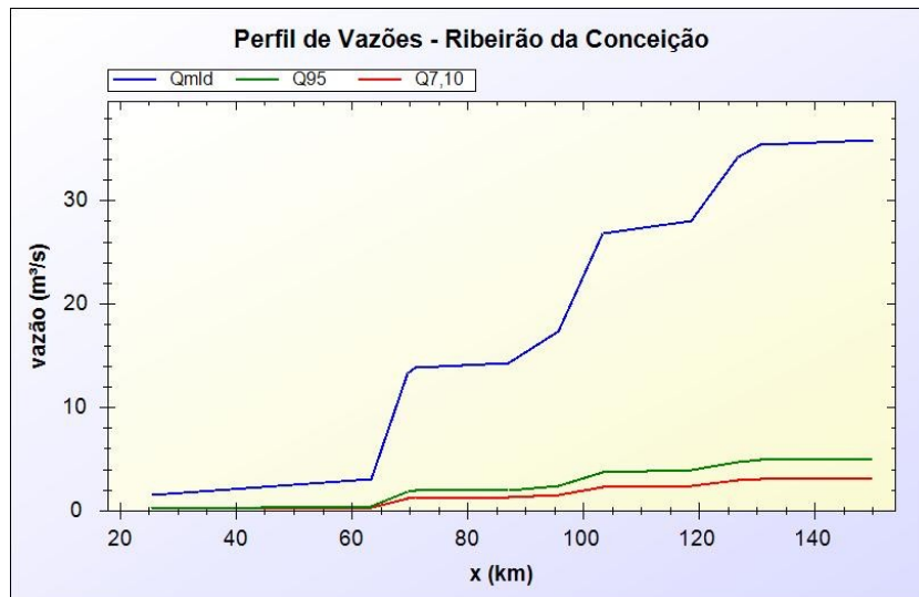
Figura A.10 - Perfil de Vazões - Ribeirão da Conceição (Bacia SF8).
