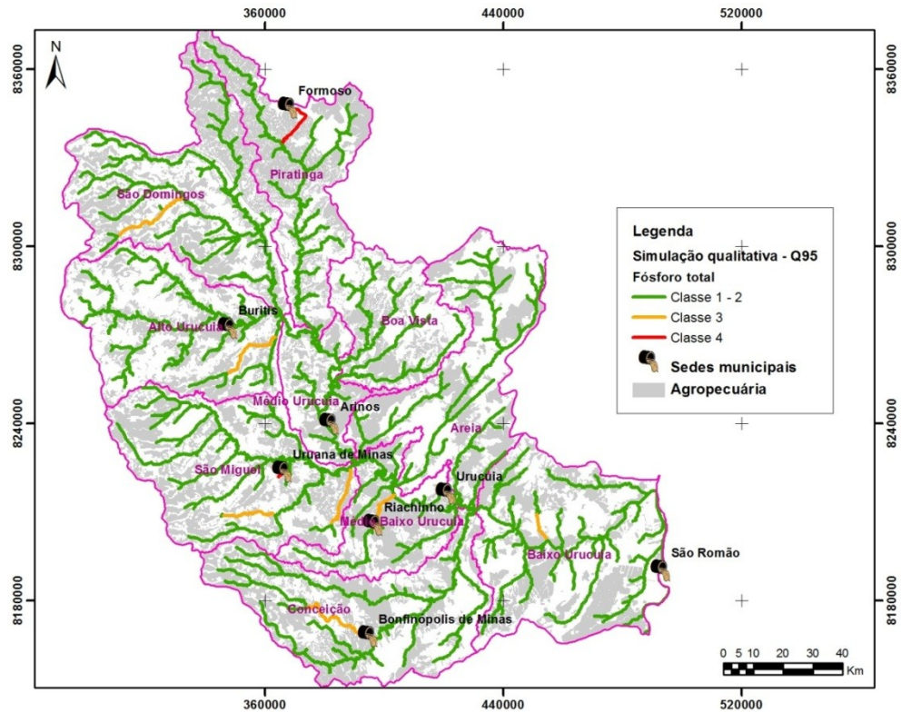
Figura 7.26 - Simulação qualitativa SF8 - Q 95 / P total.
