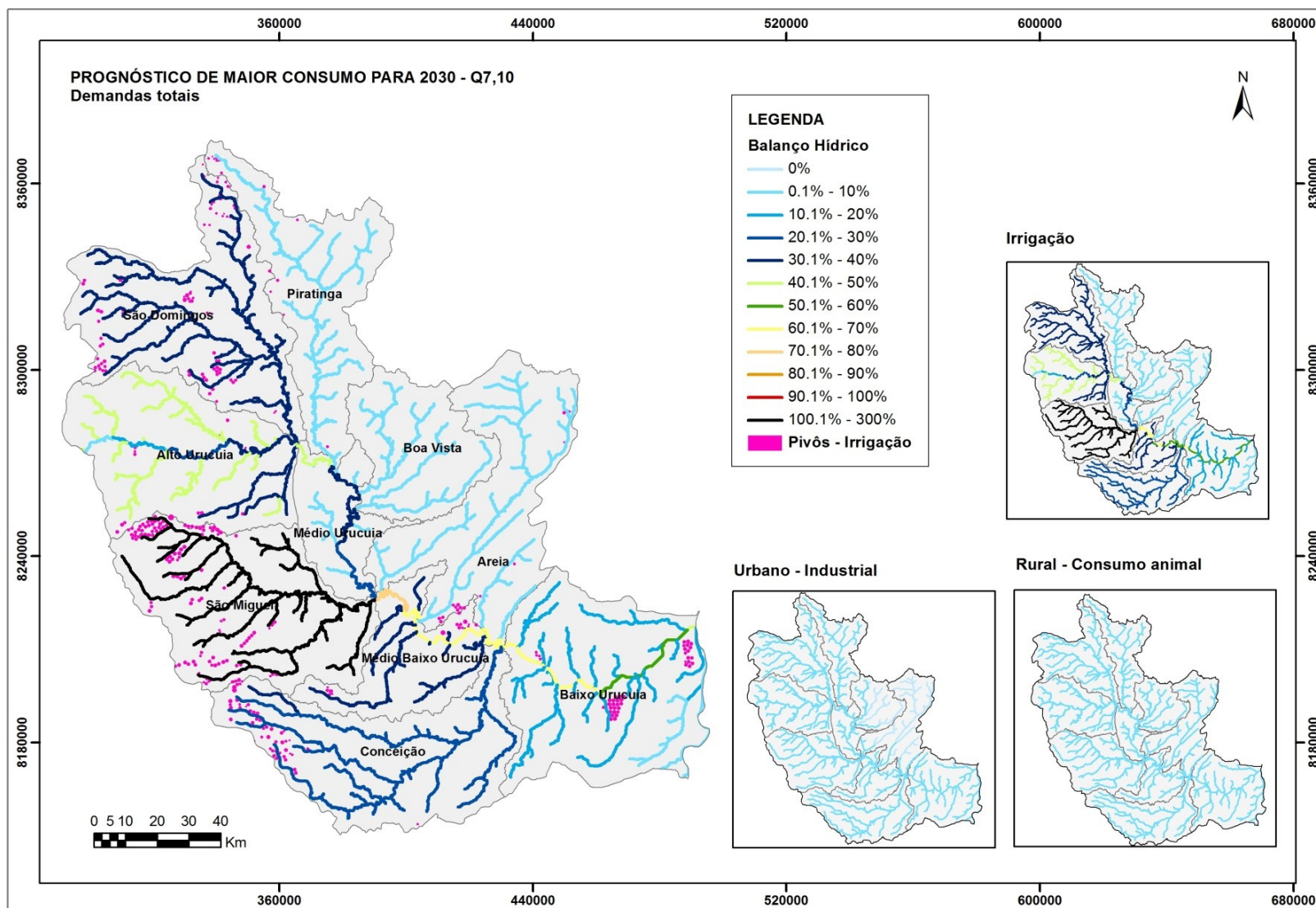
Figura 7.35 - Balanço hídrico - Cenário de maior consumo - Q7,10..
