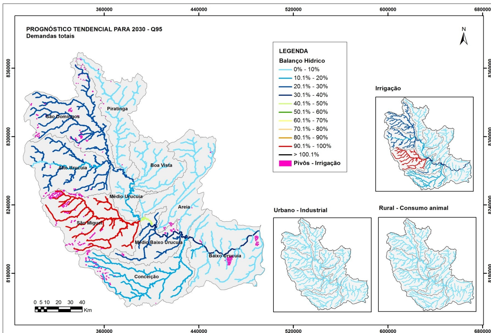
Figura 7.32 - Balanço hídrico - Cenário tendencial - Q95.
