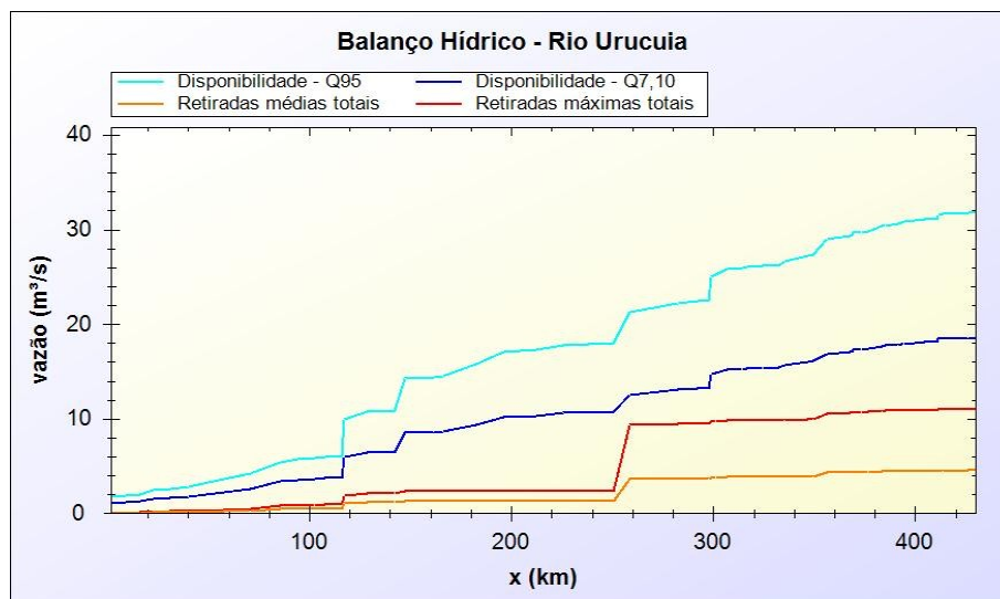
Figura 7.13 - Perfil de balanço hídrico - Rio Urucuia.
