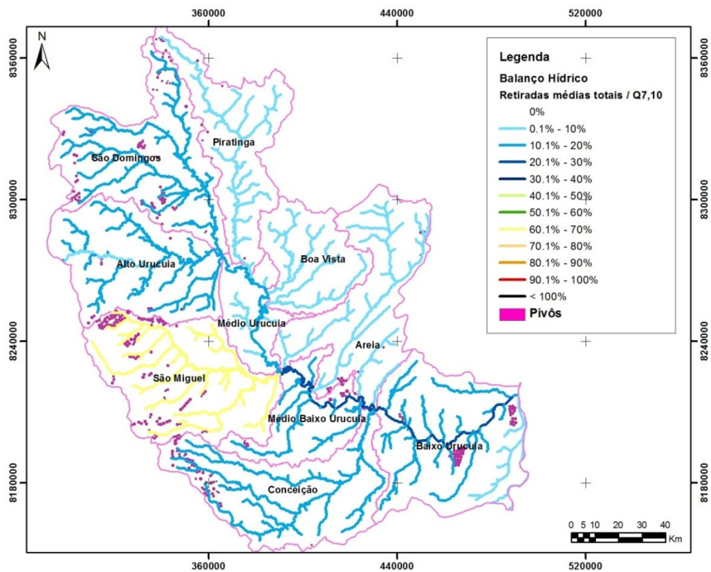
Figura 7.6 - Balanço hídrico SF8 (Retiradas médias totais / Q 7,10 ).
