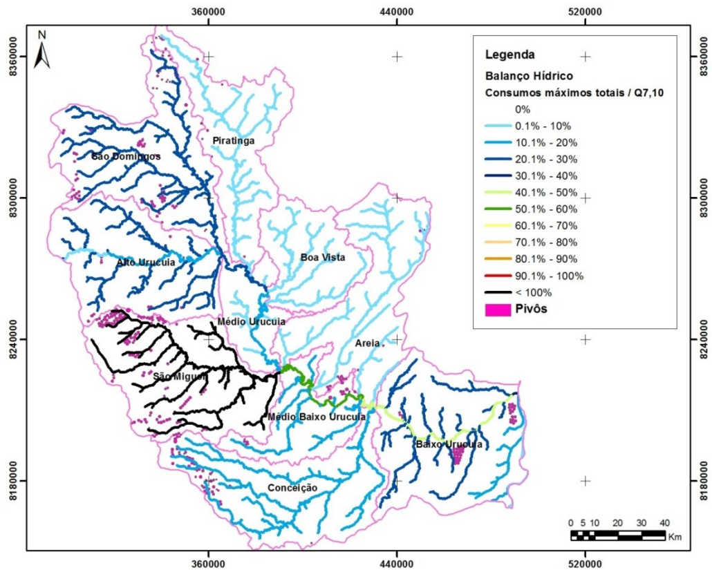
Figura 7.12 - Balanço hídrico SF8 (Consumos máximos totais / Q_{7,10} ).
