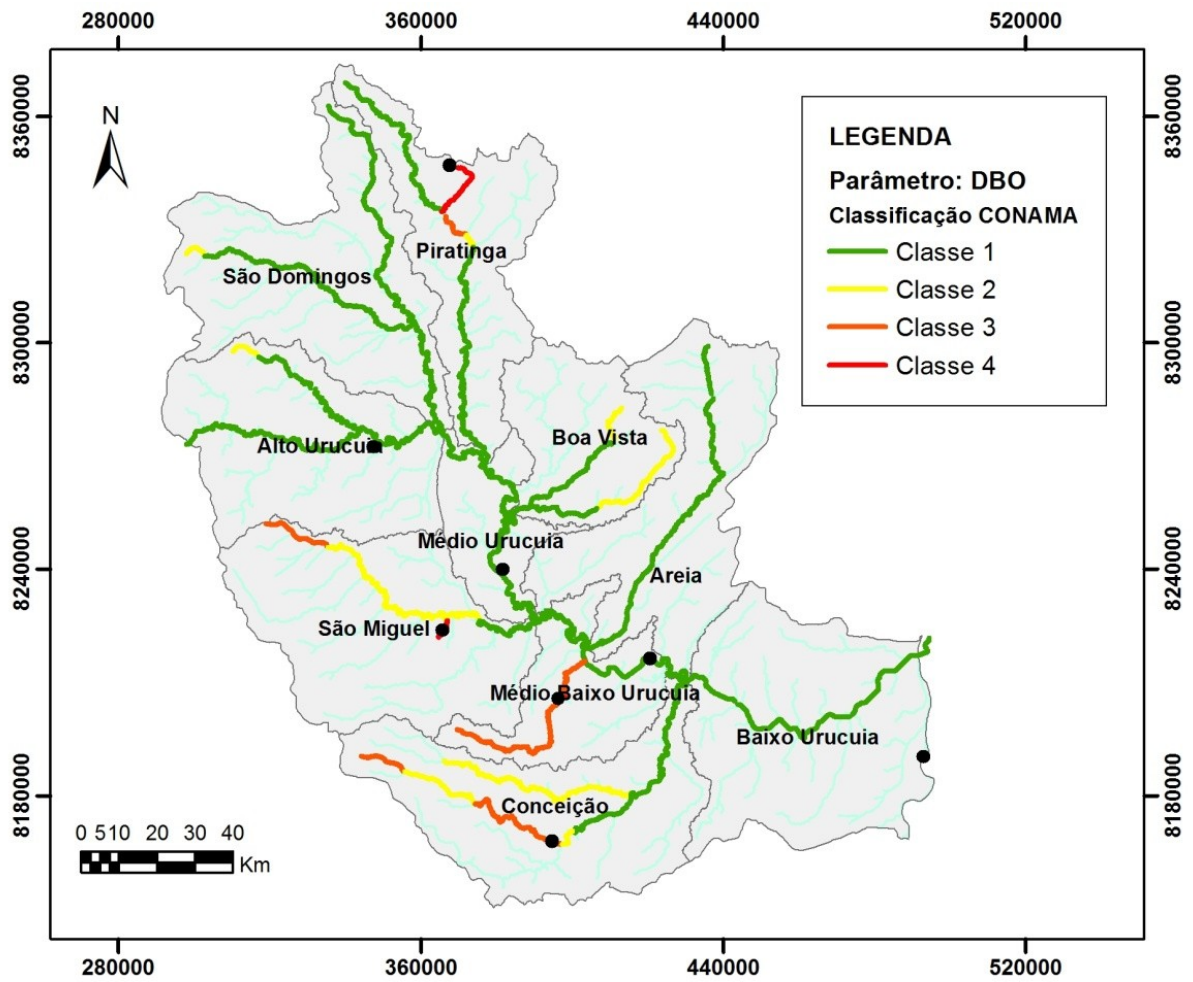
Figura 7.42 - Simulação da concentração de DBO na bacia SF8, considerando um cenário de vazão correspondente à Q_{95} .
