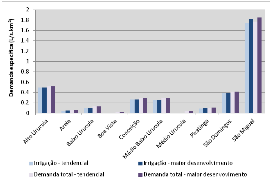
Figura 7.31 - Projeções das demandas da irrigação e total na bacia SF8 (L/s.km 2 ). Fonte: Consórcio EcoPLAN-Lume-Skill, 2011.
