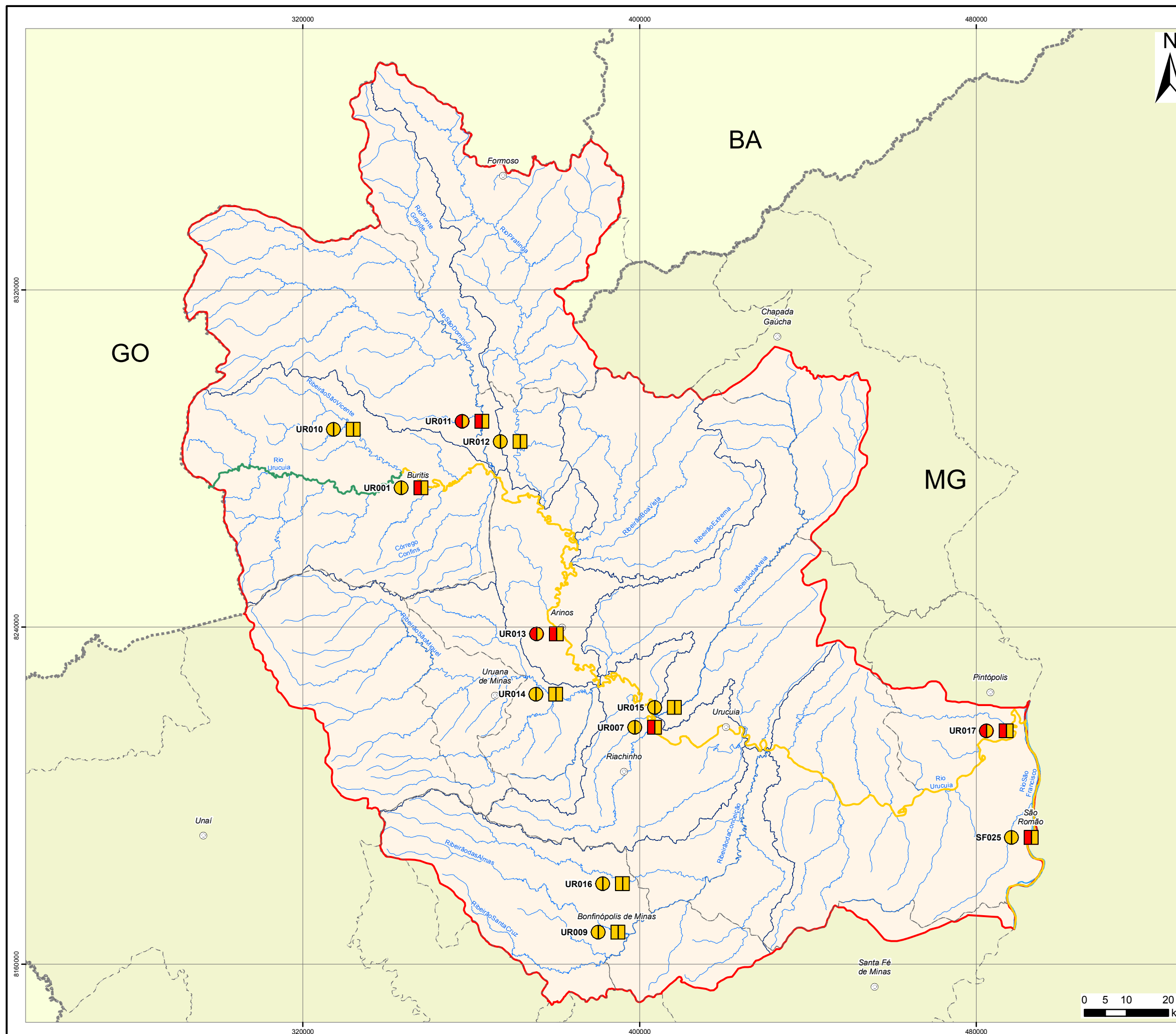
Figura 6.6 - Condição Média Frente à Classe de Qualidade (2008-2010) - Chumbo Total e Manganês Total
