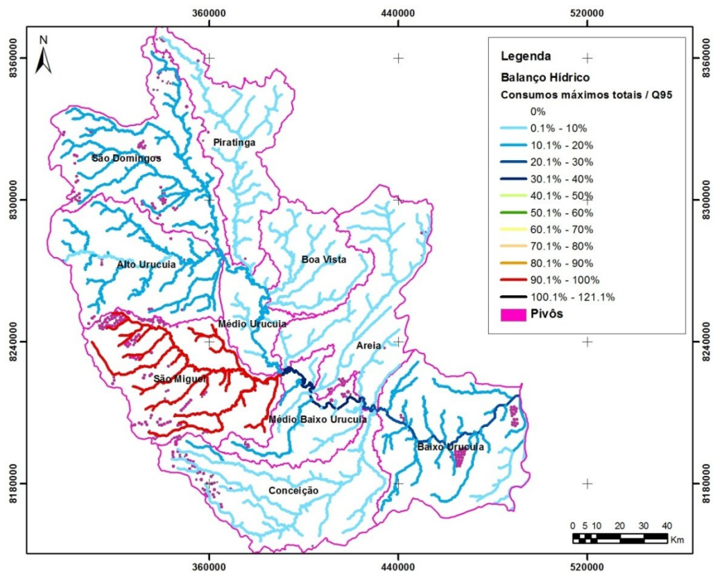
Figura 7.11 - Balanço hídrico SF8 (Consumos máximos totais / Q 95 ).
