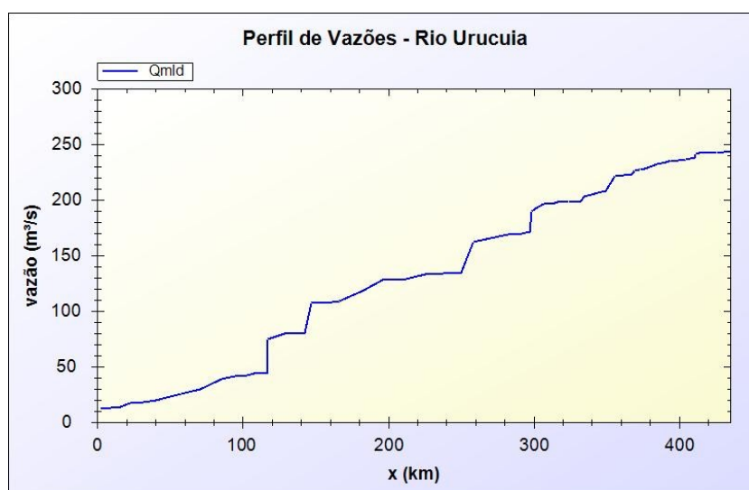
Figura A.11 - Perfil de Vazões - Rio Urucuia (Bacia SF8).
