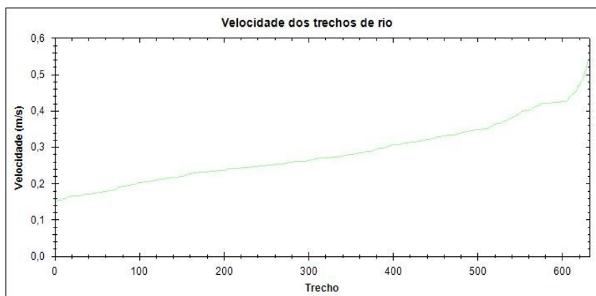
Figura 7.18 - Estimativa da velocidade em todos os segmentos da rede de drenagem.
