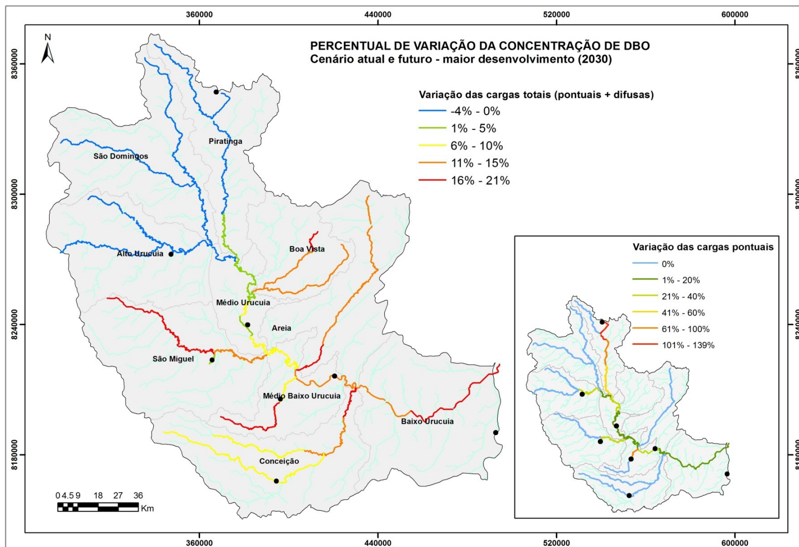
Figura 7.48 - Percentual de variação da concentração da DBO – Comparativo entre cenário atual e futuro – Q95.
