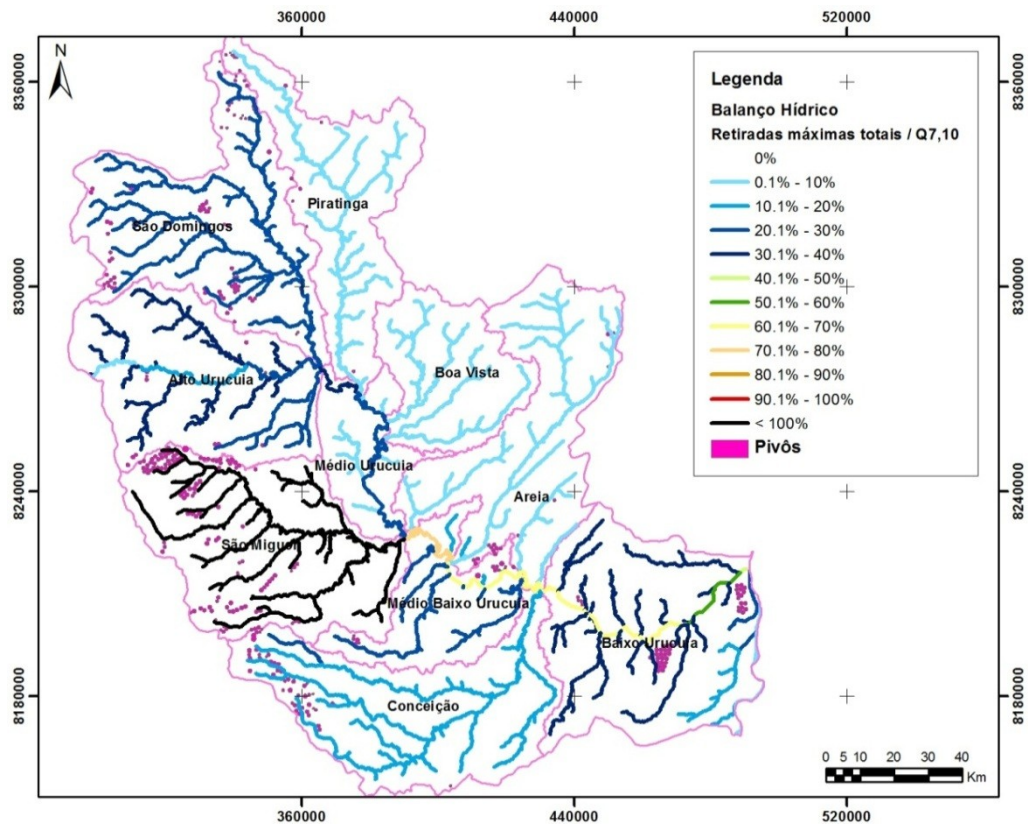
Figura 7.10 - Balanço hídrico SF8 (Retiradas máximas totais / Q 7,10 ).
