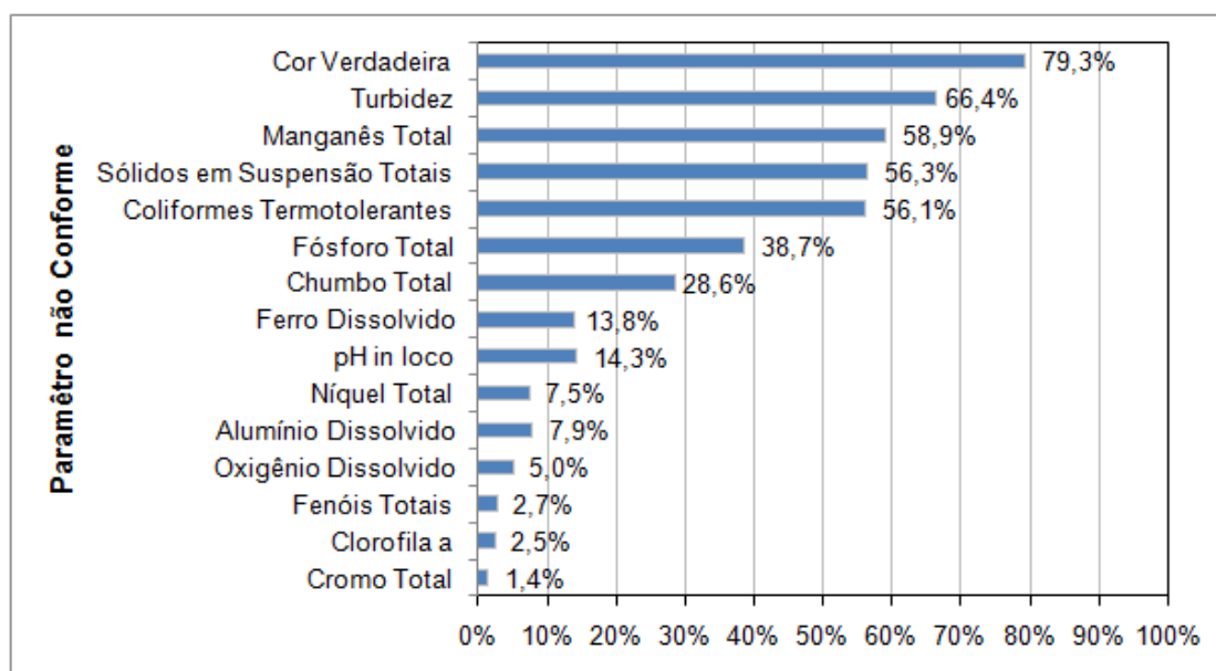
Figura 6.3 - Percentuais de Resultados Não Conformes em Relação aos Padrões de Qualidade da Classe 2, 2003 a 2010, Período de Chuva.
