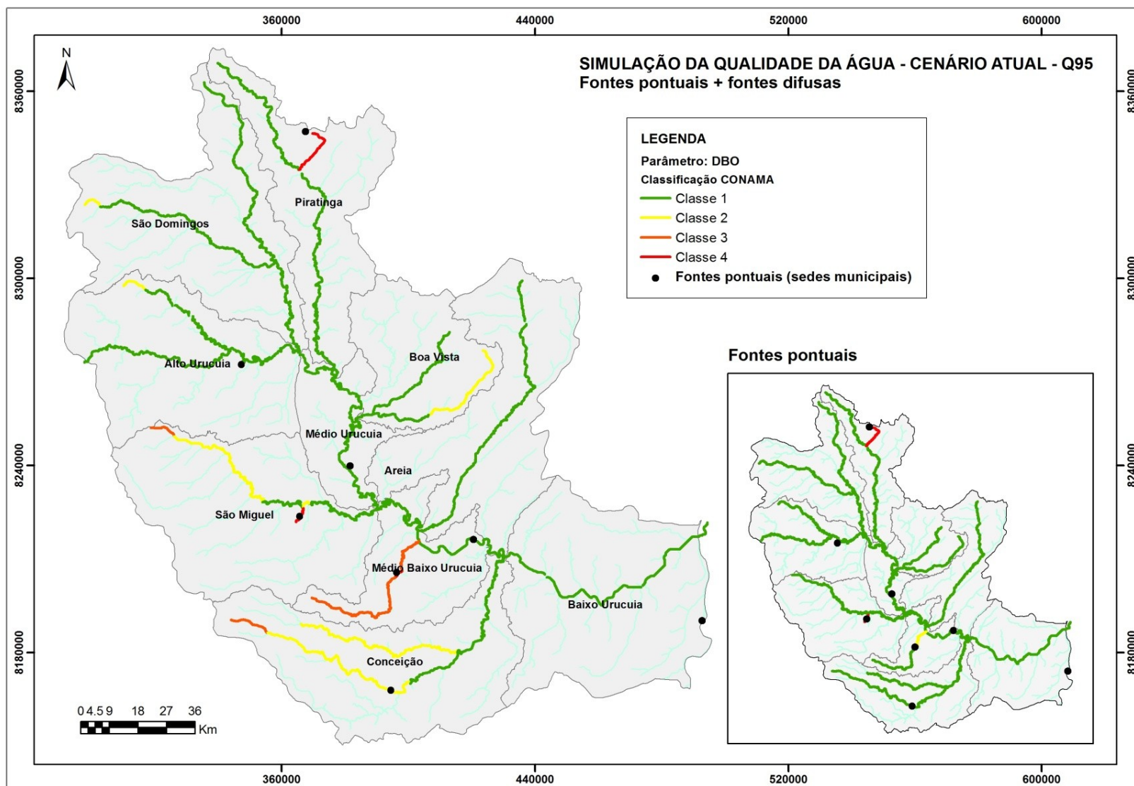
Figura 7.44 - Simulação qualitativa – Parâmetro: DBO – Cenário atual – Q95.
