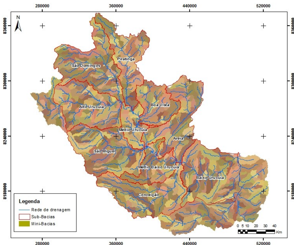
Figura A.3 - Resultado da discretização do MNT - Bacia SF8.
