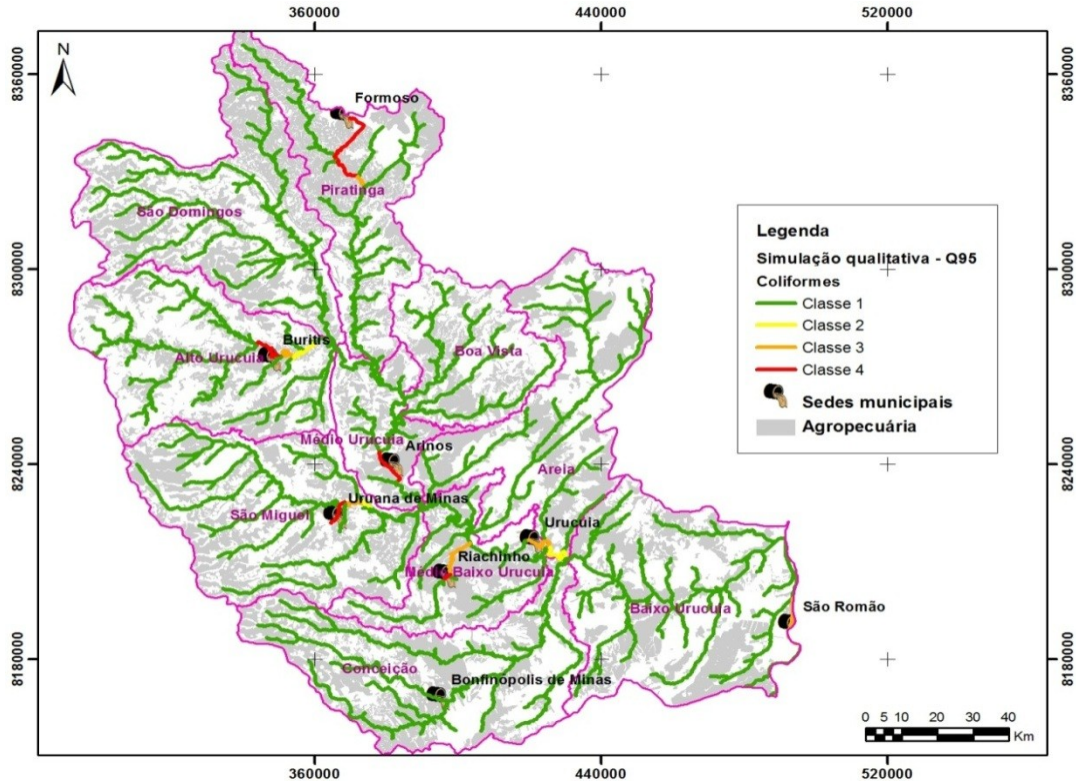
Figura 7.28 - Simulação qualitativa SF8 - Q95 / Coliformes.
