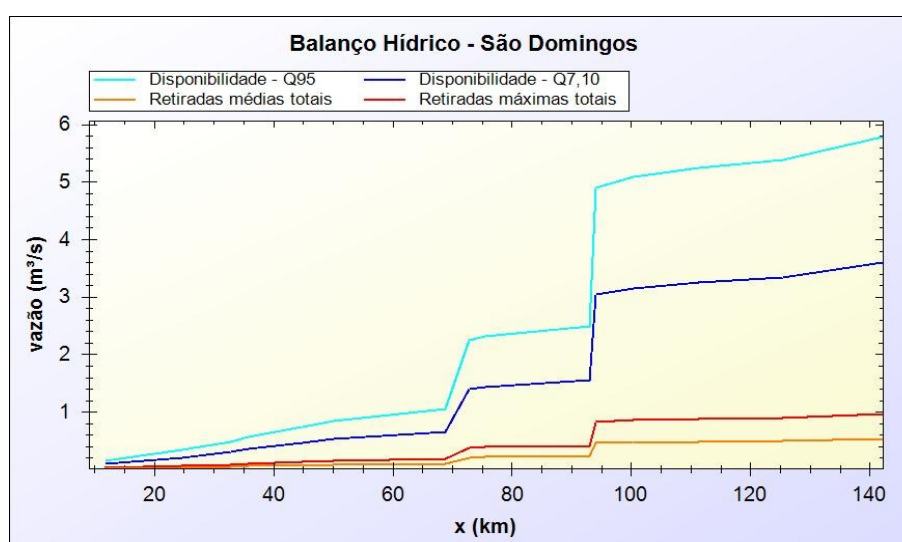
Figura 7.15 - Perfil de balanço hídrico - Ribeirão São Domingos.
