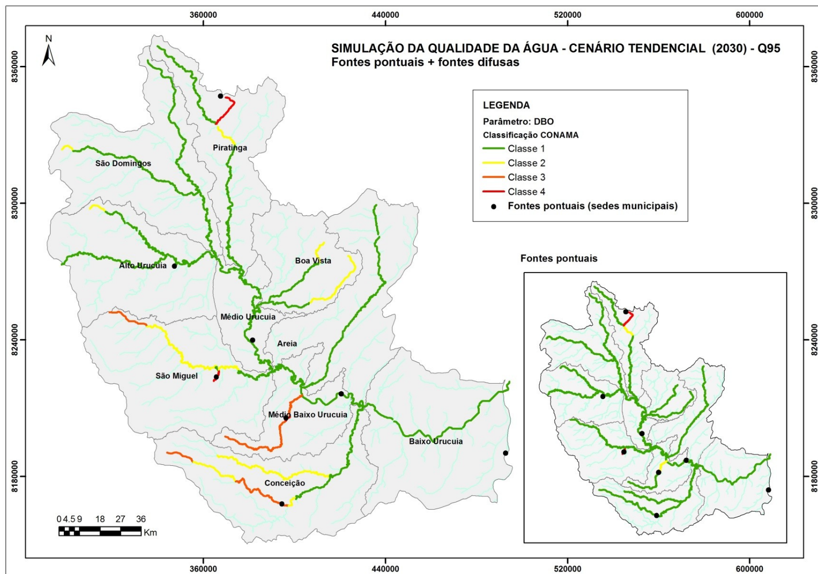
Figura 7.45 - Simulação qualitativa – Parâmetro: DBO – Cenário tendencial – Q95.
