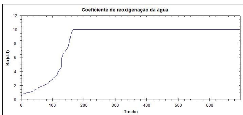
Figura 7.20 - Estimativa da reoxigenação da água em todos os segmentos da rede de drenagem.
