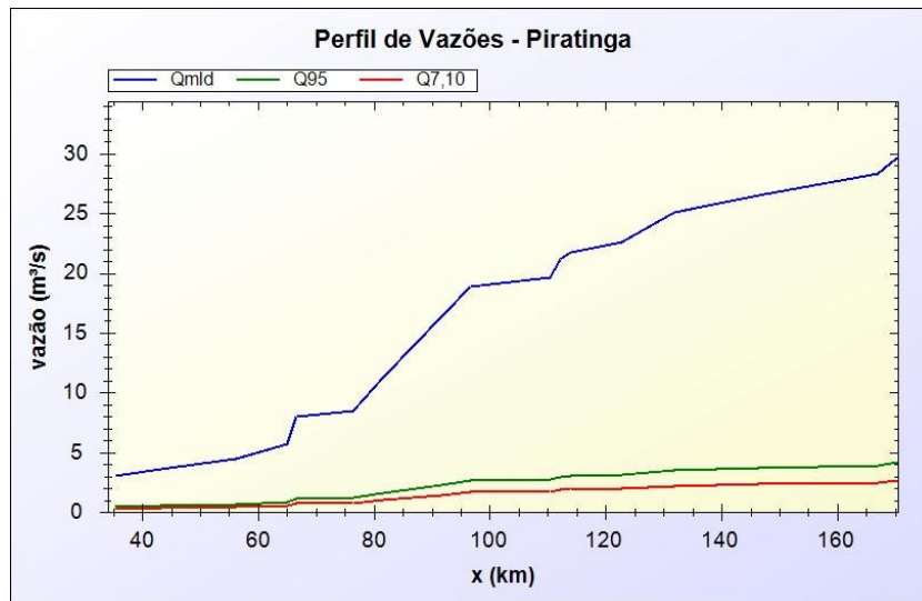
Figura A.9 - Perfil de Vazões - Rio Piratinga (Bacia SF8).
