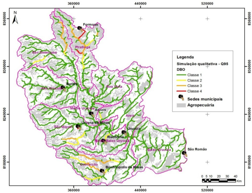
Figura 7.22 - Simulação qualitativa SF8 – Q 95 / DBO.
