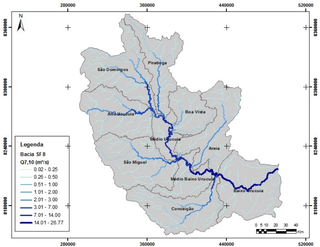
Figura A.7 - Disponibilidade por trecho de rio – Q7,10 (Bacia SF8).
