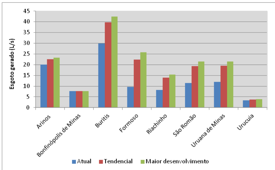
Figura 7.36 - Estimativa da geração de esgotos nas sedes urbanas da bacia SF8.
