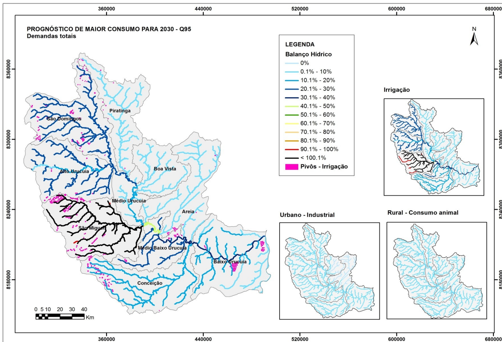
Figura 7.34 - Balanço hídrico - Cenário de maior consumo - Q95.
