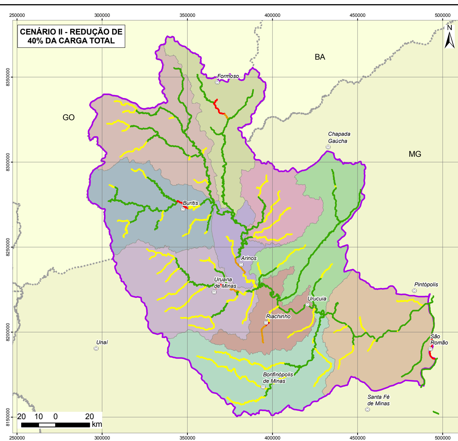
Figura 7.53 - Cenários de Intervenção Qualitativa - Parâmetro Coliformes Termotolerantes
