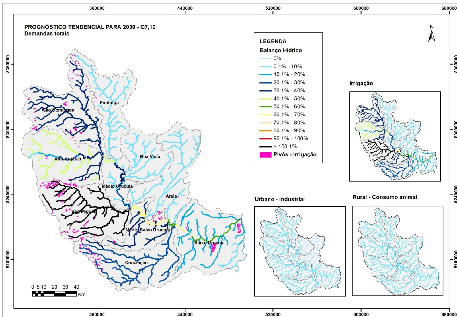
Figura 7.33 - Balanço hídrico - Cenário tendencial - Q7,10.
