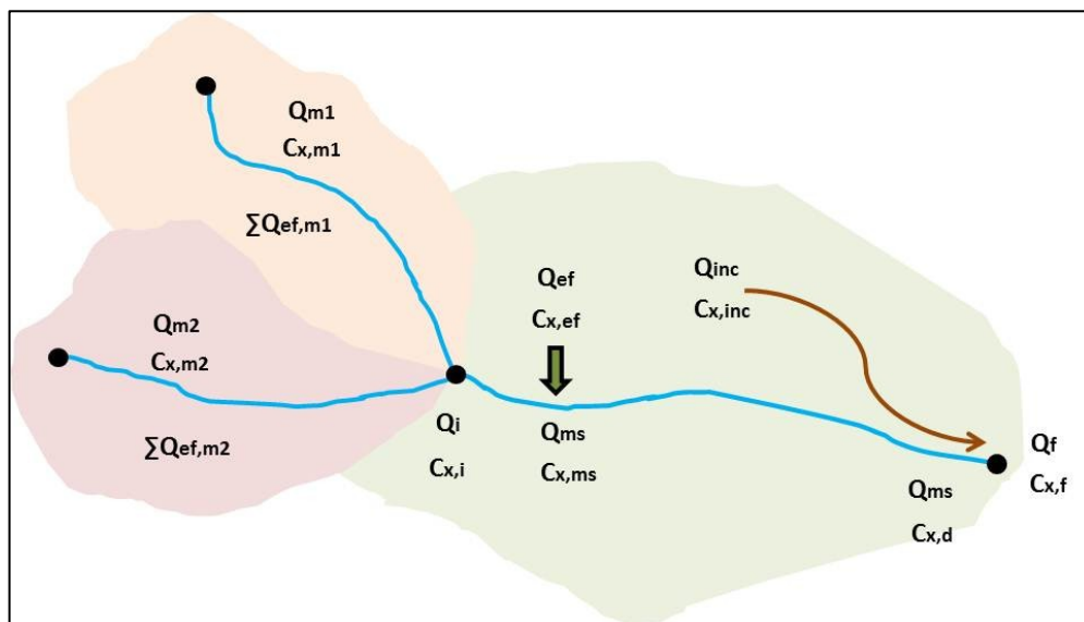
Figura 7.16 - Esquema ilustrando as variáveis envolvidas no modelo qualitativo do sistema.
