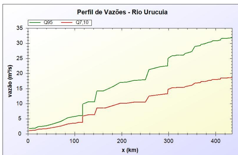
Figura A.12 - Perfil de Vazões - Rio Urucuia (Bacia SF8).
