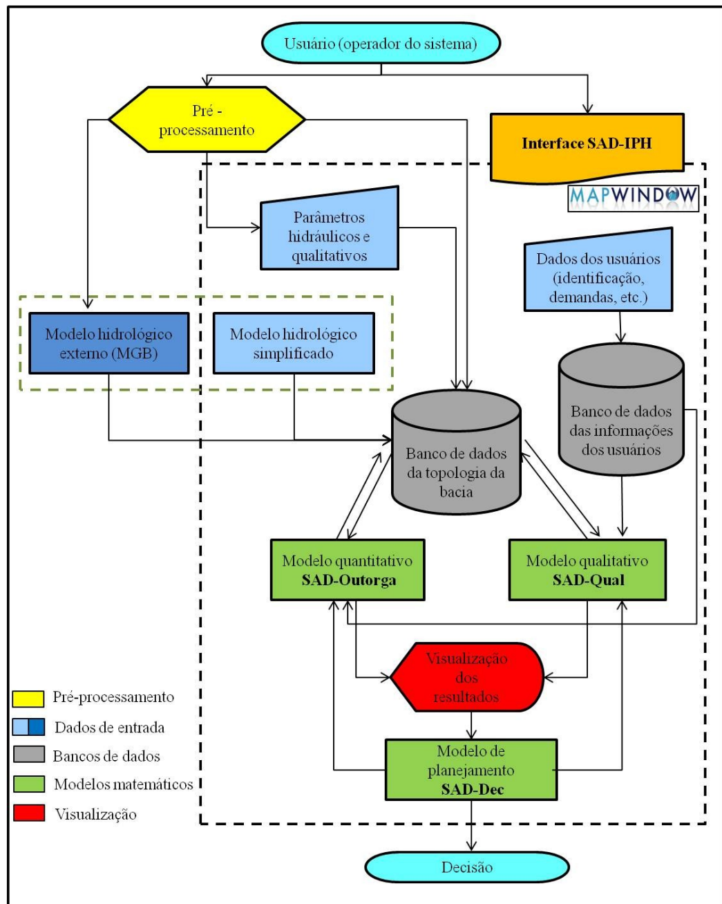
Figura 7.2 - Algoritmo geral de funcionamento do SAD-IPH.
