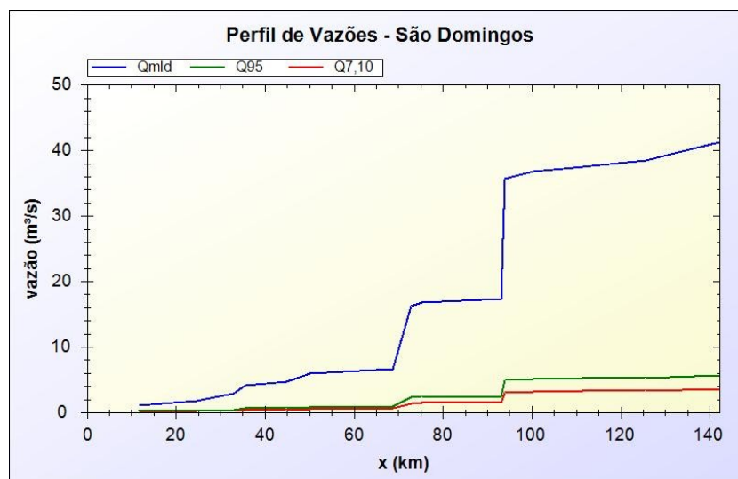
Figura A.8 - Perfil de Vazões - Rio São Domingos (Bacia SF8).
