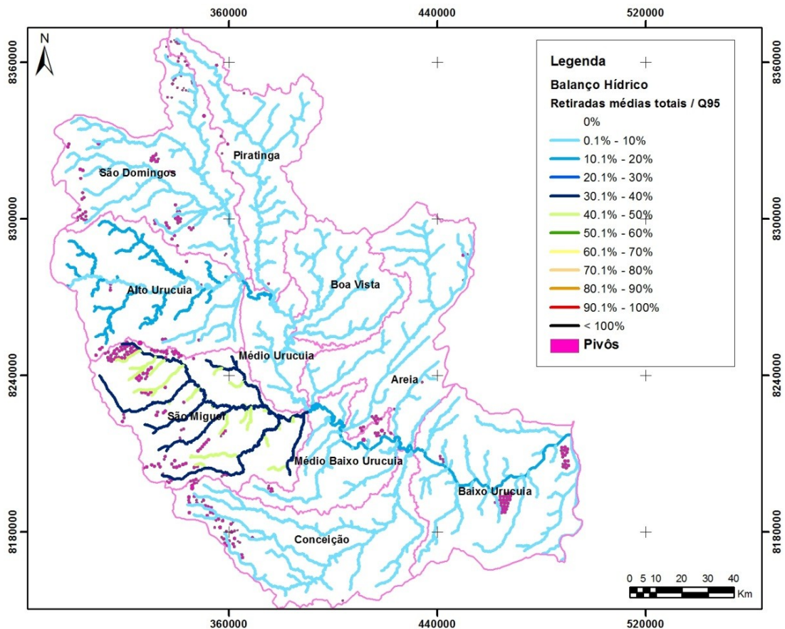
Figura 7.5 - Balanço hídrico SF8 (Retiradas médias totais / Q_{95} ).
