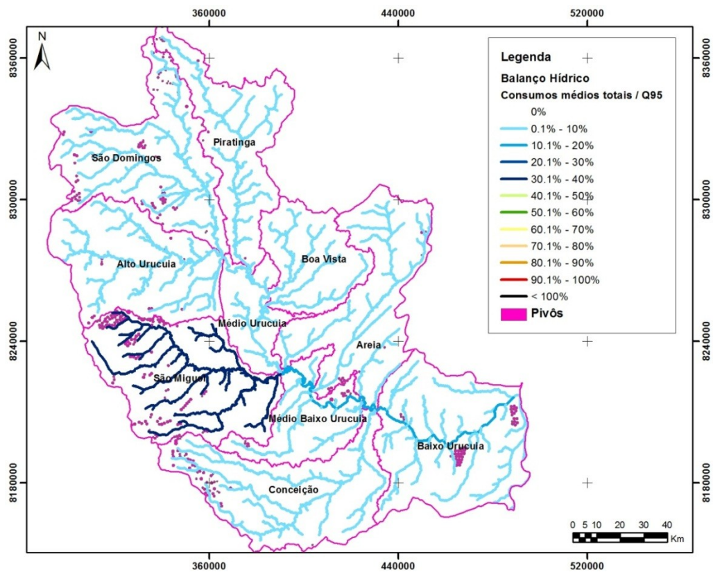
Figura 7.7 - Balanço hídrico SF8 (Consumos médios totais / Q 95 ).
