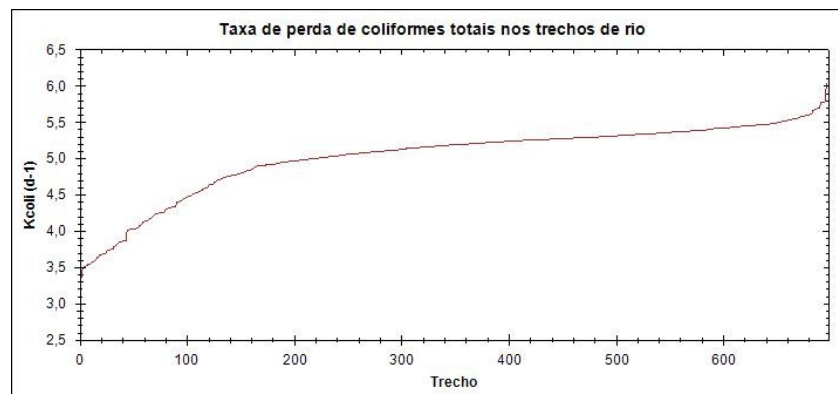
Figura 7.21 - Estimativa taxa de perda de coliformes em todos os segmentos da rede de drenagem.
