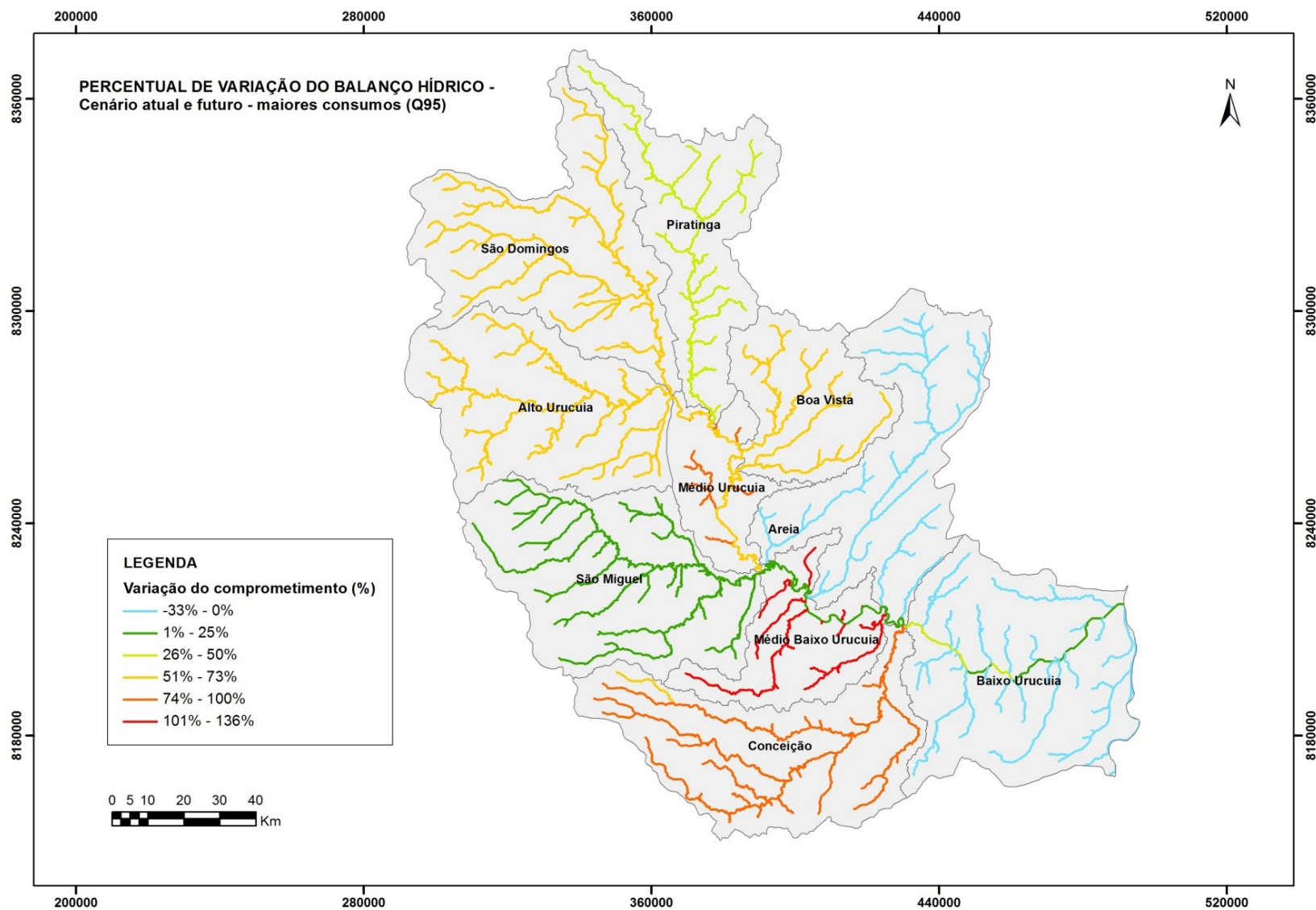
Figura 7.47 - Percentual de variação do balanço hídrico – comparativo entre cenários atual e futuro – Q95.
