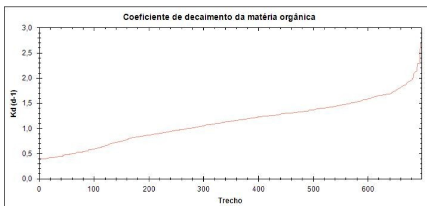
Figura 7.19 - Estimativa do decaimento da matéria orgânica em todos os segmentos da rede de drenagem.
