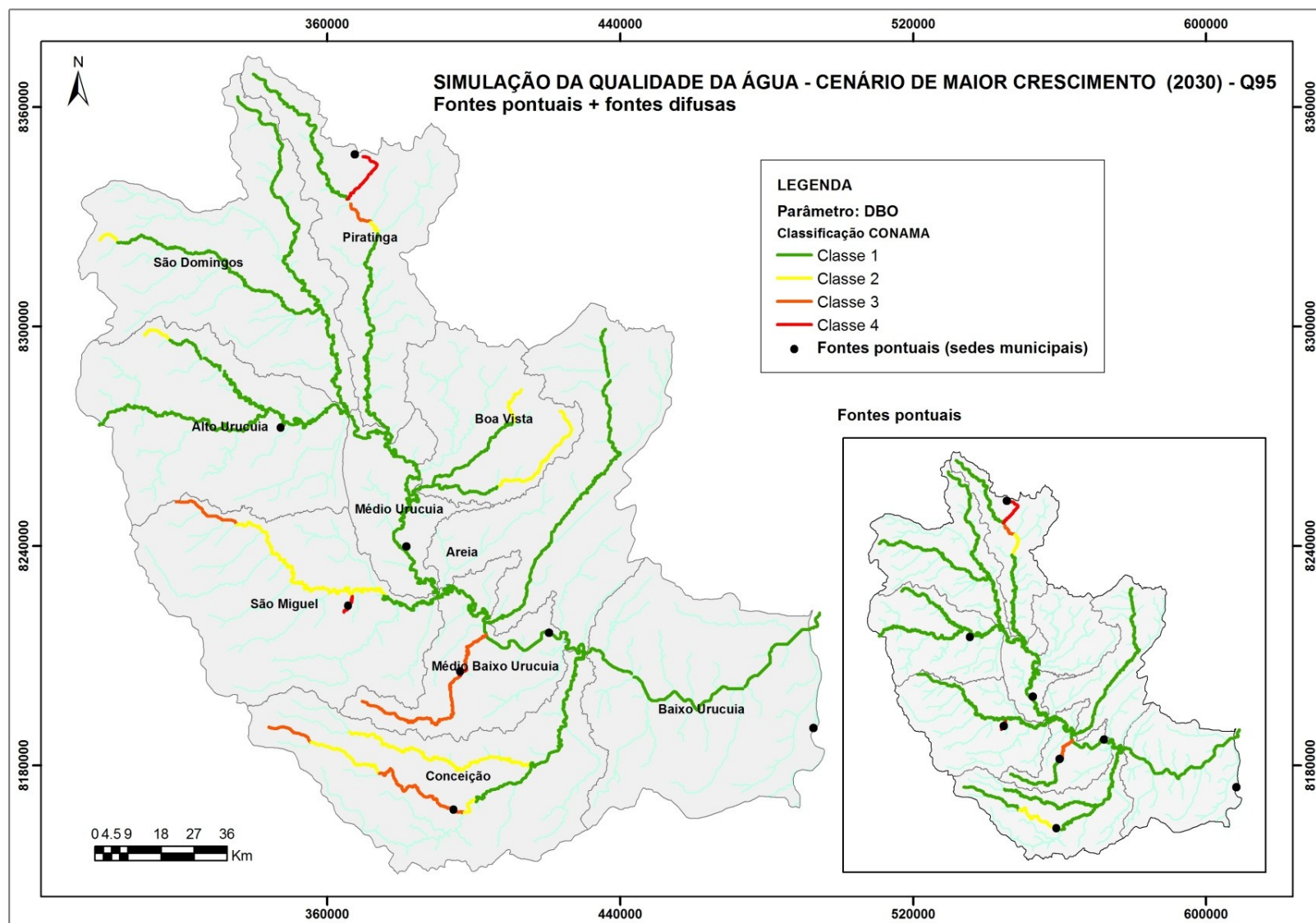
Figura 7.46 - Simulação qualitativa – Parâmetro: DBO – Cenário de maior desenvolvimento – Q95.
