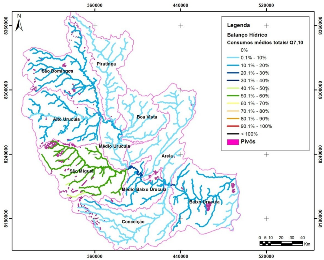
Figura 7.8 - Balanço hídrico SF8 (Consumos médios totais / Q_{7,10} ).
