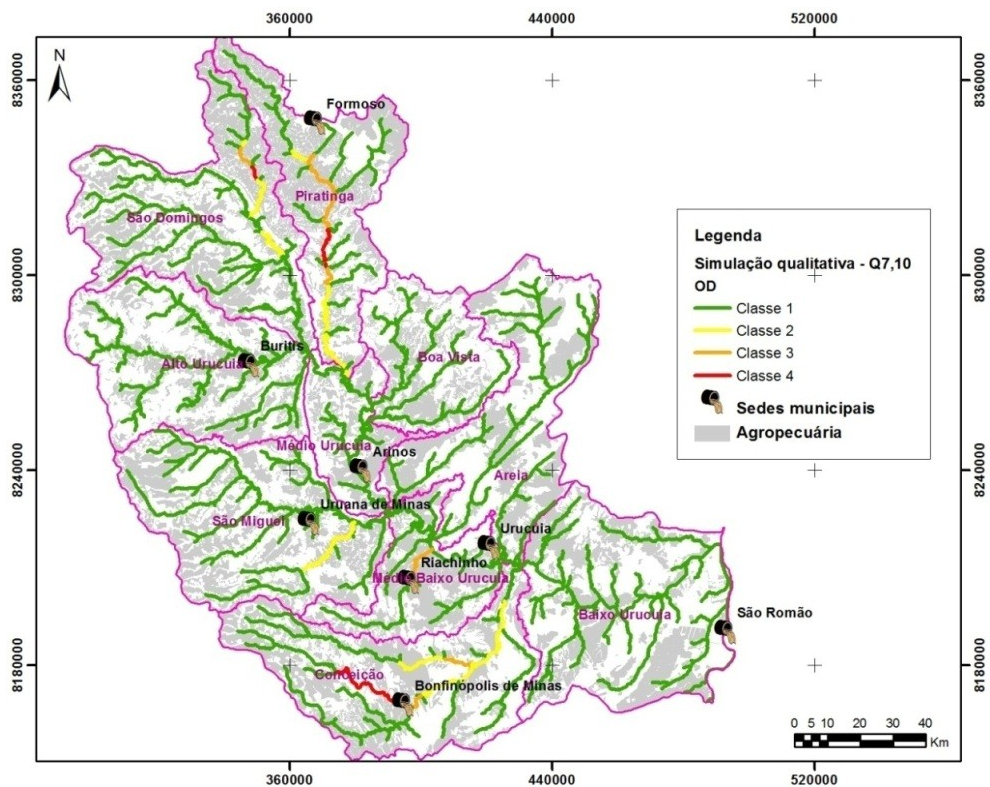
Figura 7.25 - Simulação qualitativa SF8 - Q 7,10 / OD.
