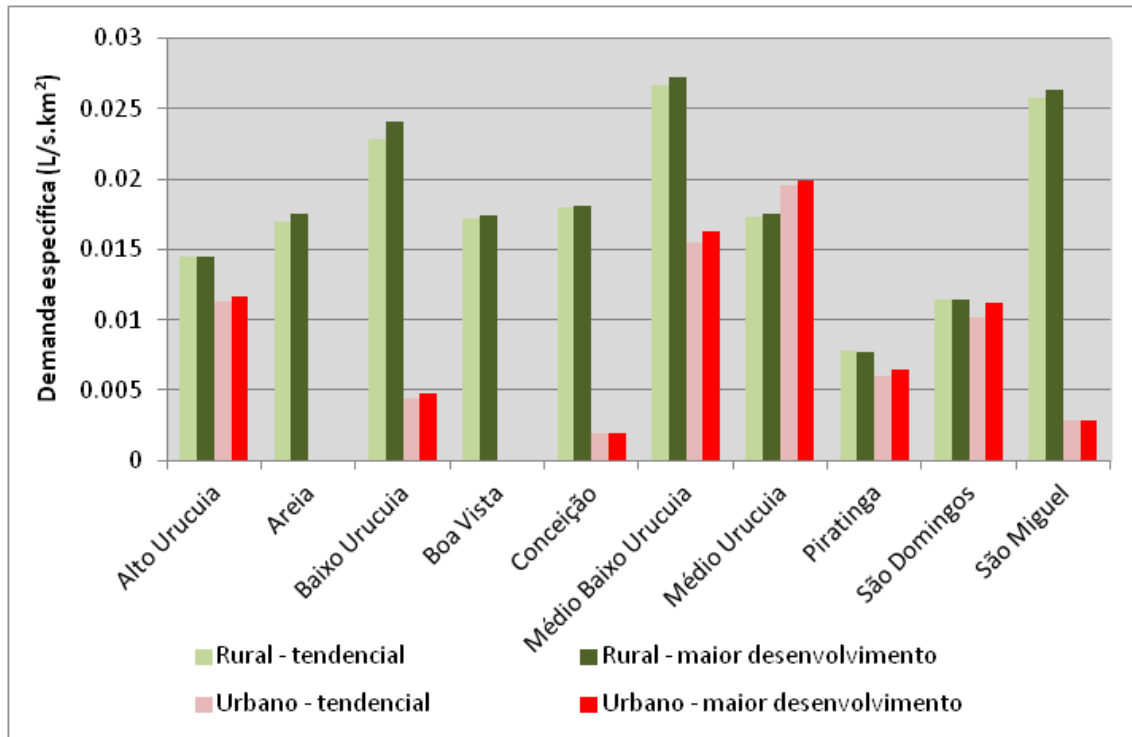
Figura 7.30 - Projeções das demandas rural e urbana na bacia SF8 (L/s.km 2 ). Fonte: Consórcio EcoPLAN-Lume-Skill, 2011.
