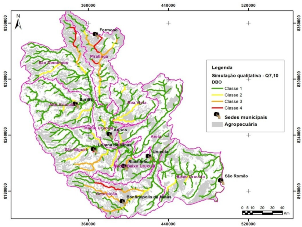
Figura 7.23 - Simulação qualitativa SF8 - Q 7,10 / DBO.
