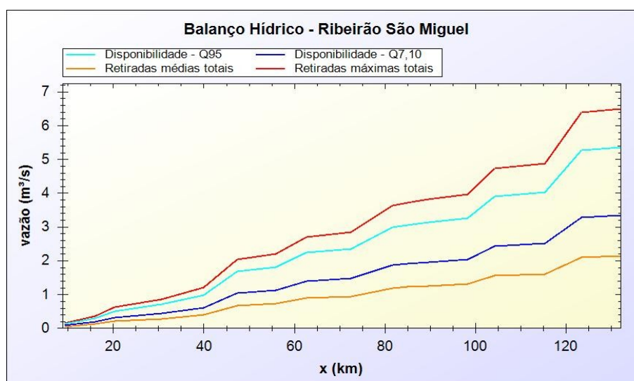
Figura 7.14 - Perfil de balanço hídrico - Ribeirão São Miguel.
