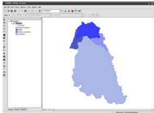
Figura 138 – Shape Aquíferos
