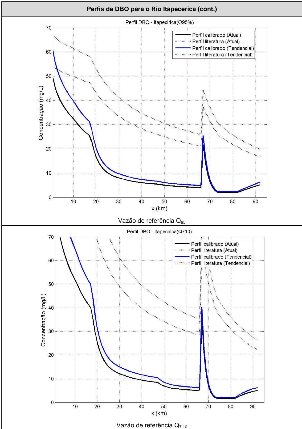
Figura 24 – Perfis de DBO para o Rio Itapecirica
