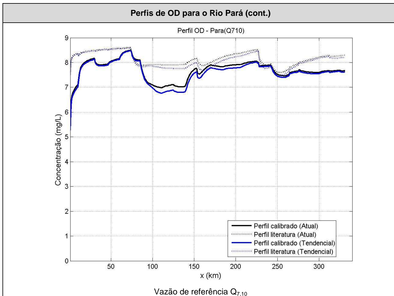
Figura 37 – Perfis de OD para o Rio Pará
