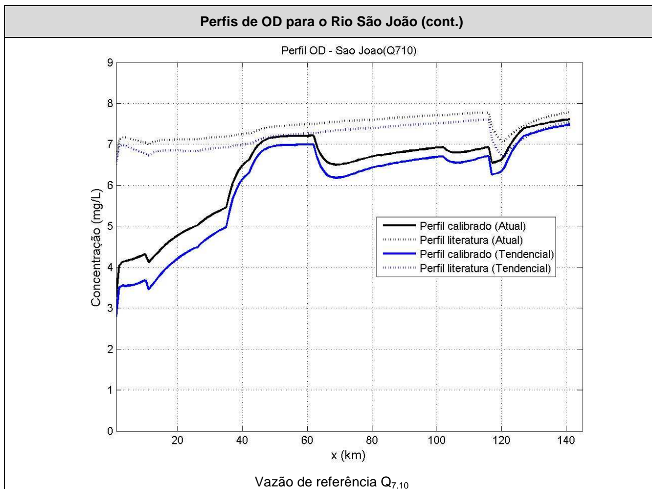
Figura 29 – Perfis de OD para o Rio São João
