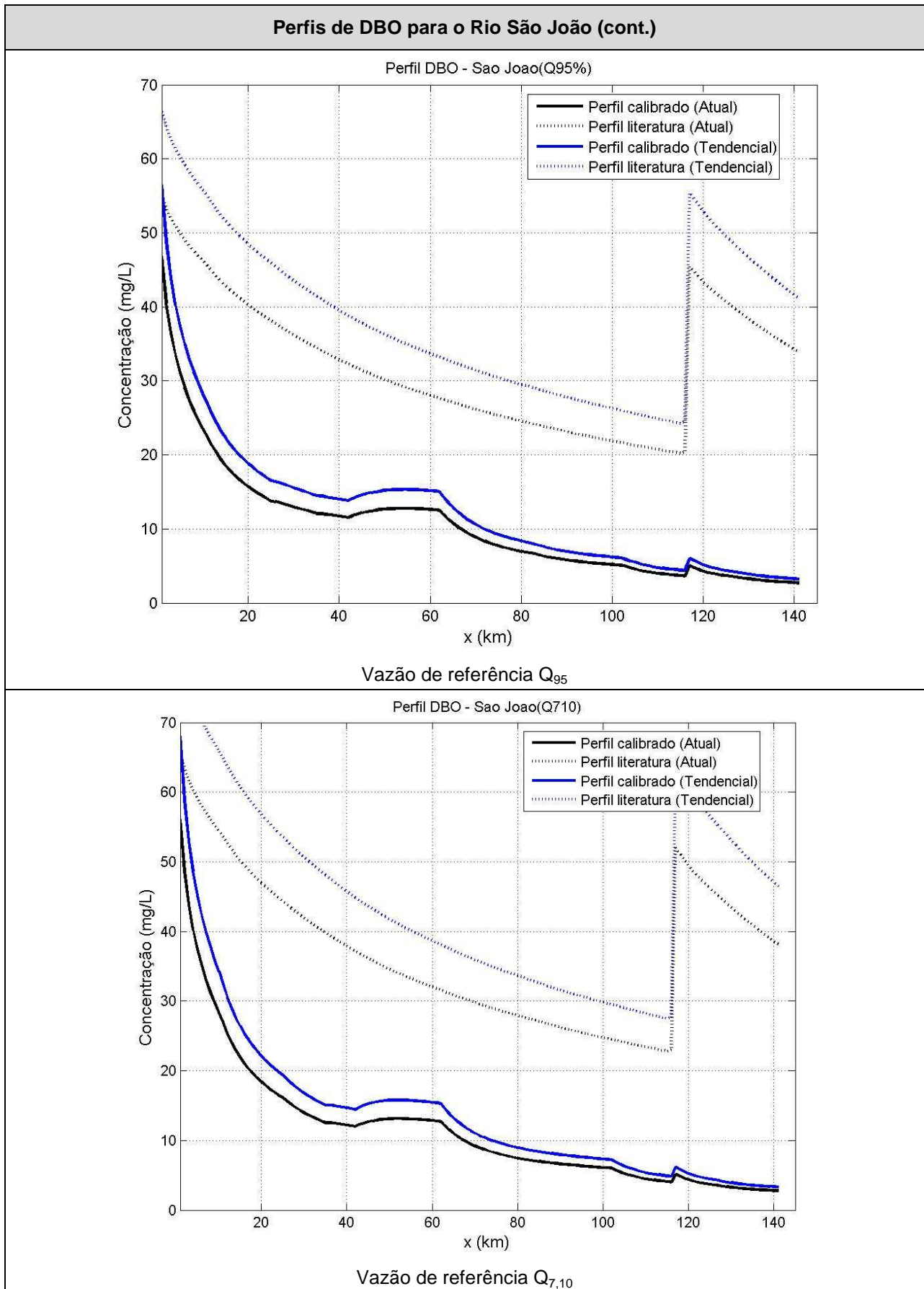
Figura 28 – Perfis de DBO para o Rio São João Fonte: Processamento TESE Tecnologia em Sistemas Espaciais Ltda.
