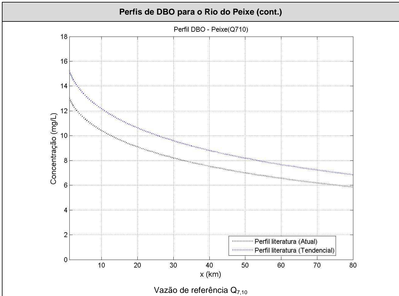
Figura 32 – Perfis de DBO para o Rio do Peixe
