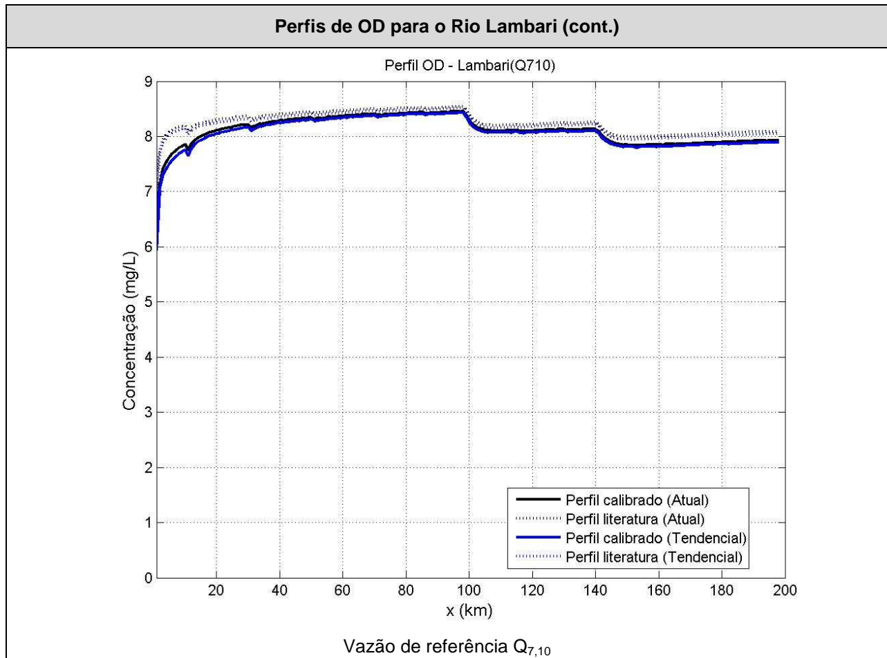
Figura 31 – Perfis de OD para o Rio Lambari
