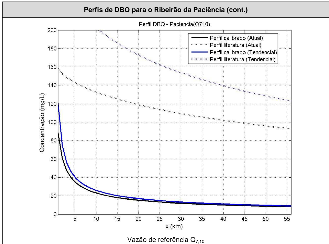
Figura 26 – Perfis de DBO para o Ribeirão da Paciência
