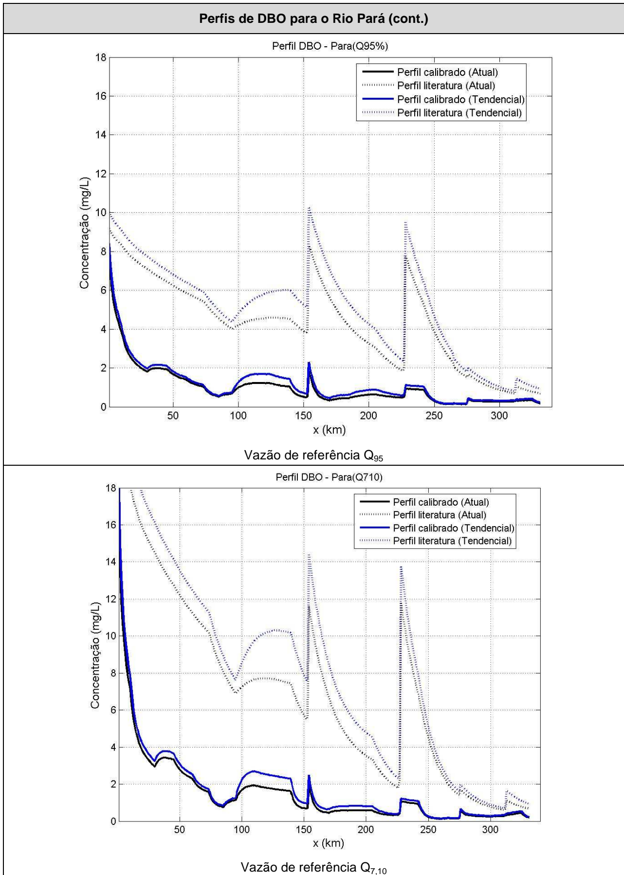
Figura 36 – Perfis de DBO para o Rio Pará
