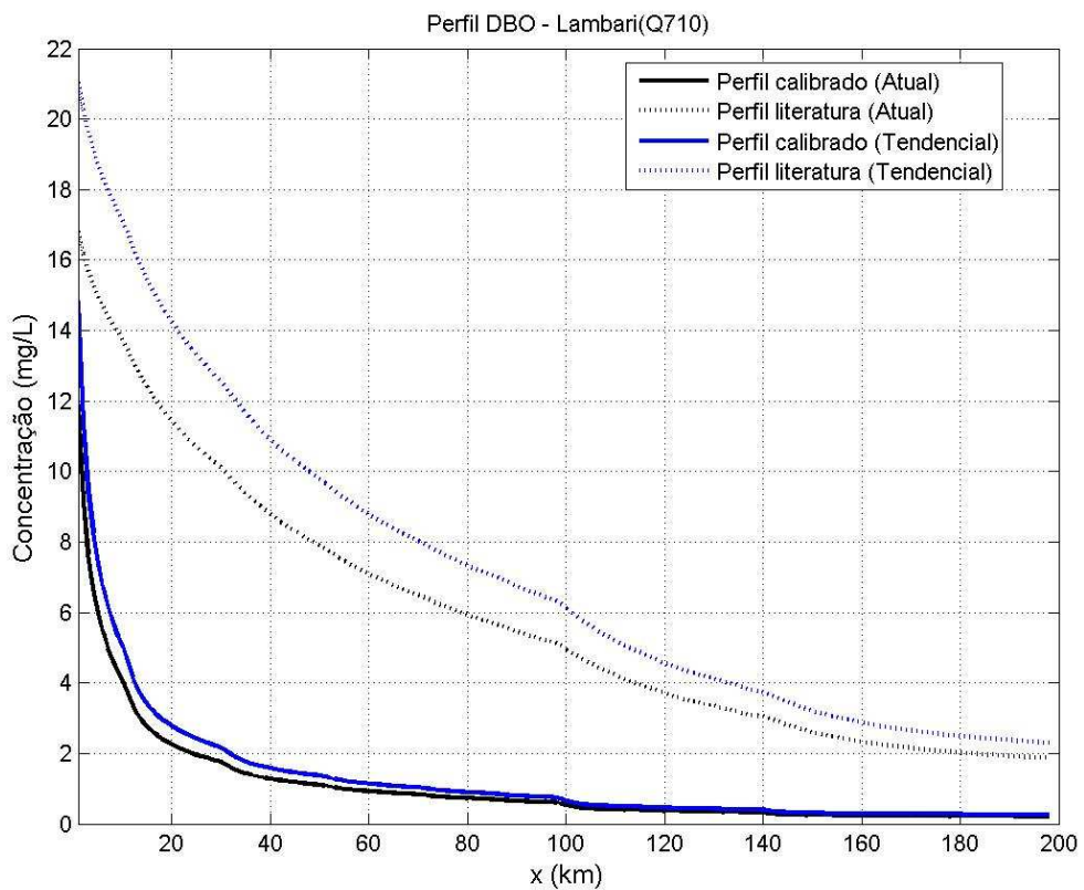
Figura 30 – Perfis de DBO para o Rio Lambari
