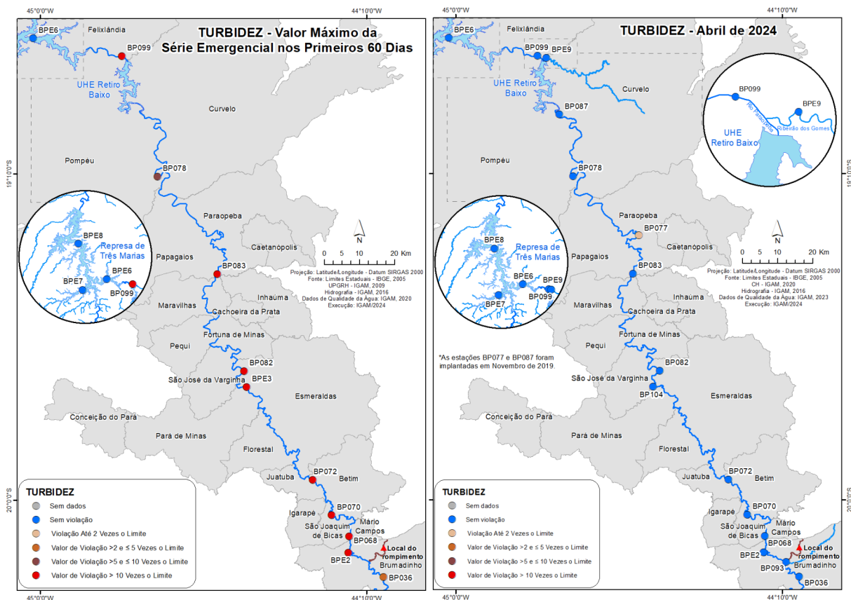
Figura 8 - Resultados dos valores máximos de turbidez para cada estação de monitoramento nos primeiros 60 dias após o rompimento da B-I e os resultados do mês de abril de 2024
