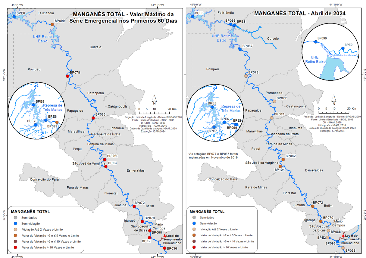
Figura 10 - Resultados de manganês total para cada estação de monitoramento nos primeiros 60 dias após o rompimento da B-I e os resultados do mês de abril de 2024
