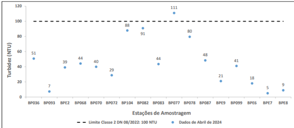
Figura 7 - Resultados de turbidez para abril de 2024
