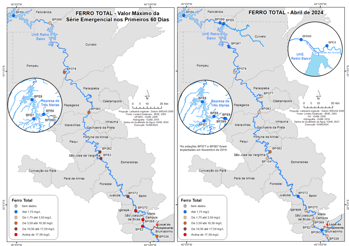
Figura 12 - Resultados dos valores máximos de ferro total para cada estação de monitoramento nos primeiros 60 dias após o rompimento da B-I e os resultados do mês de abril de 2024
