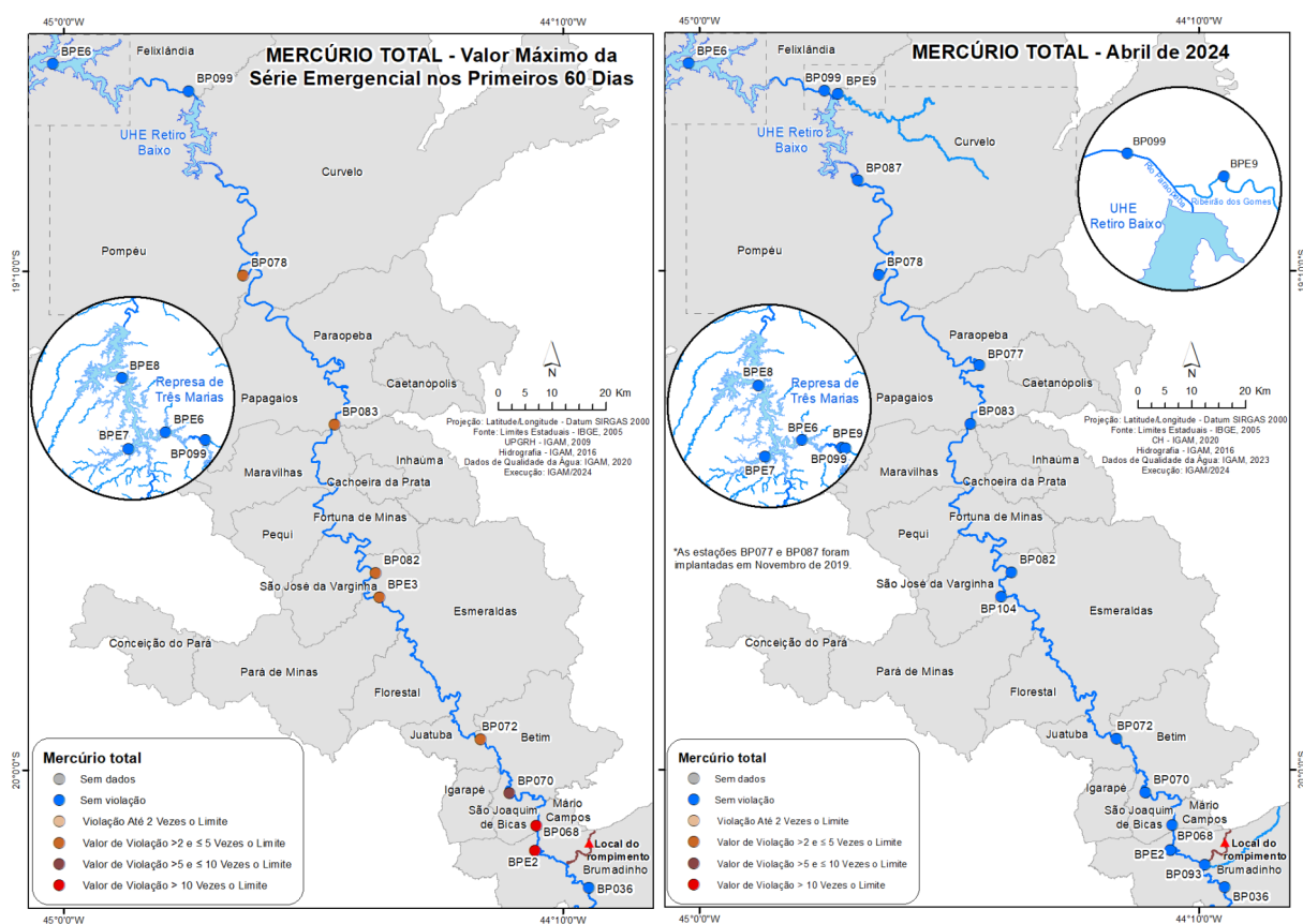
Figura 6 - Resultados dos valores máximos de mercúrio total para cada estação de monitoramento nos primeiros 60 dias após o rompimento da B-I e os resultados do mês de abril de 2024
