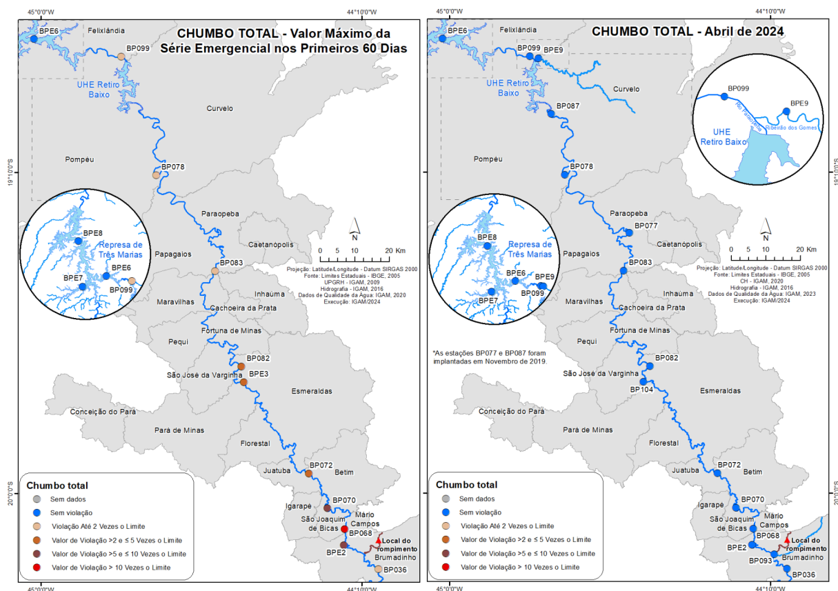
Figura 5 - Resultados dos valores máximos de chumbo total para cada estação de monitoramento nos primeiros 60 dias após o rompimento da B-I e os resultados do mês de abril de 2024
