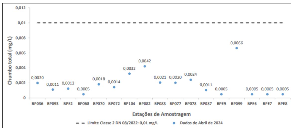
Figura 4 - Resultados de chumbo total para abril de 2024
