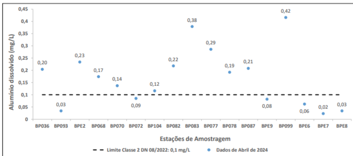
Figura 2 - Resultados de alumínio dissolvido para abril de 2024
