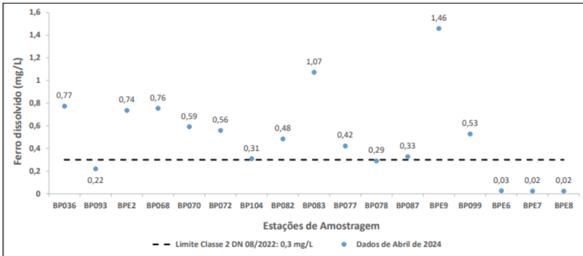
Figura 13 - Resultados de ferro dissolvido para abril de 2024
