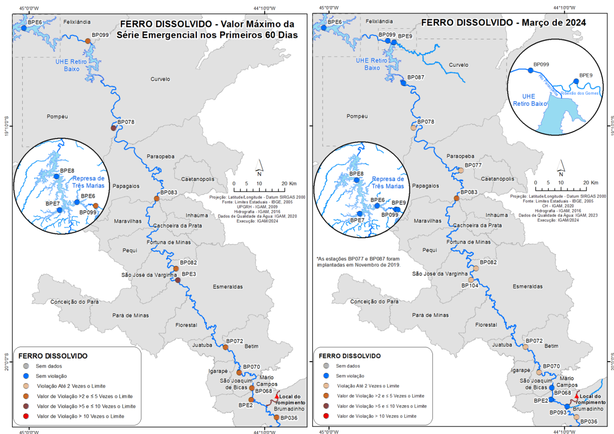
Figura 14 - Resultados dos valores máximos de ferro dissolvido para cada estação de monitoramento nos primeiros 60 dias após o rompimento da B-I e os resultados do mês de abril de 2024
