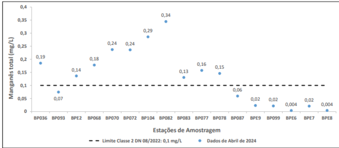
Figura 9 - Resultados de manganês total para abril de 2024
