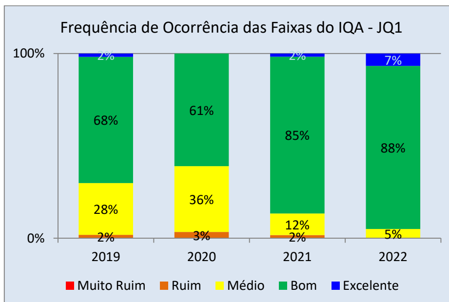
Figura 1: Distribuição percentual das faixas do IQA na CH JQ1 para os anos de 2019 a 2022
