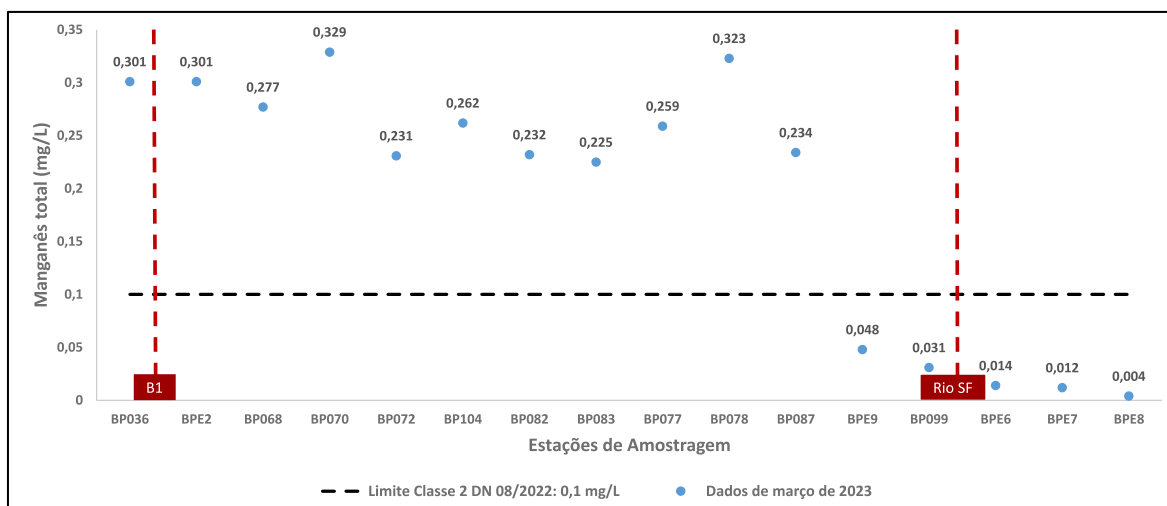
Figura 6 - Resultados de Manganês total para março de 2023
