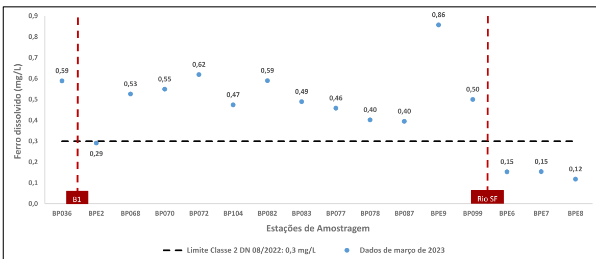
Figura 8 - Resultados de Ferro dissolvido para março de 2023
