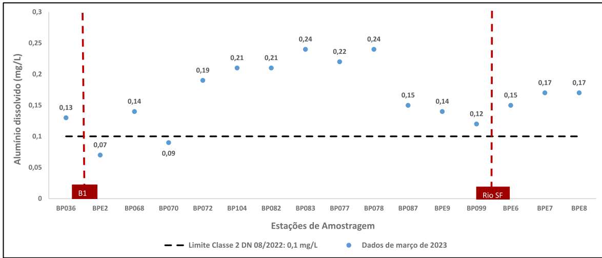
Figura 3 - Resultados de Alumínio dissolvido para março de 2023
