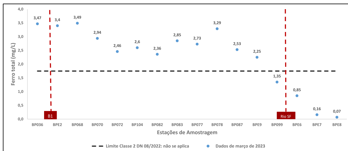
Figura 7 - Resultados de Ferro total para março de 2023
