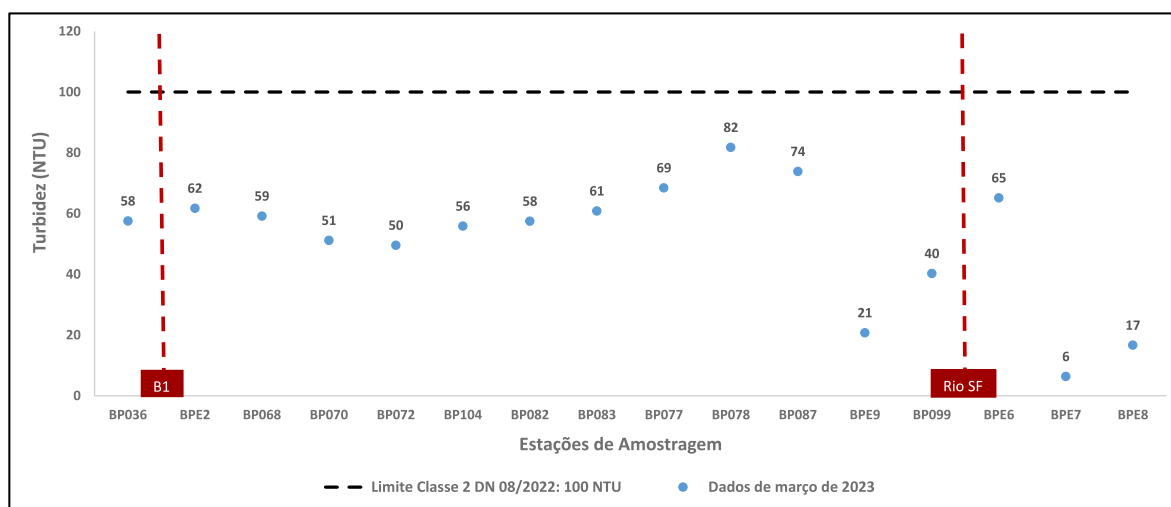
Figura 5 - Resultados de Turbidez para março de 2023
