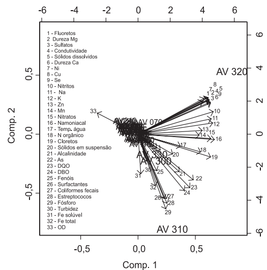
Figura 6. Gráfico “biplot” de escores e pesos (“loadings”) para as duas primeiras componentes principais para todas as estações da rede de monitoramento do alto curso do Rio das Velhas. Escala de escores no intervalo de -1 a +1 e escala de pesos no intervalo de -6 a +6
