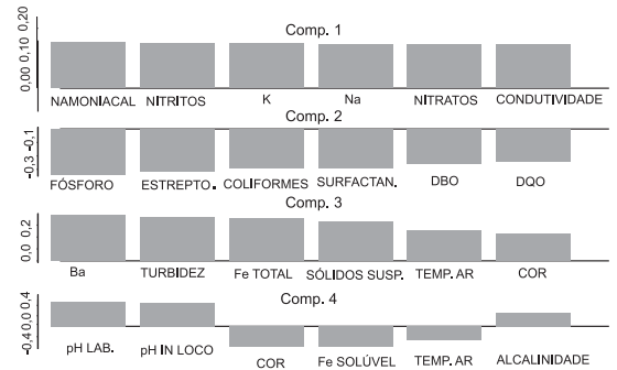
Figura 5. As contribuições dos 6 parâmetros mais importantes nas 4 primeiras componentes principais
