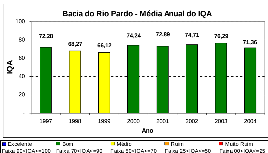
Figura 8.1: Evolução Temporal da Média Anual do IQA na Bacia do Rio Pardo.
