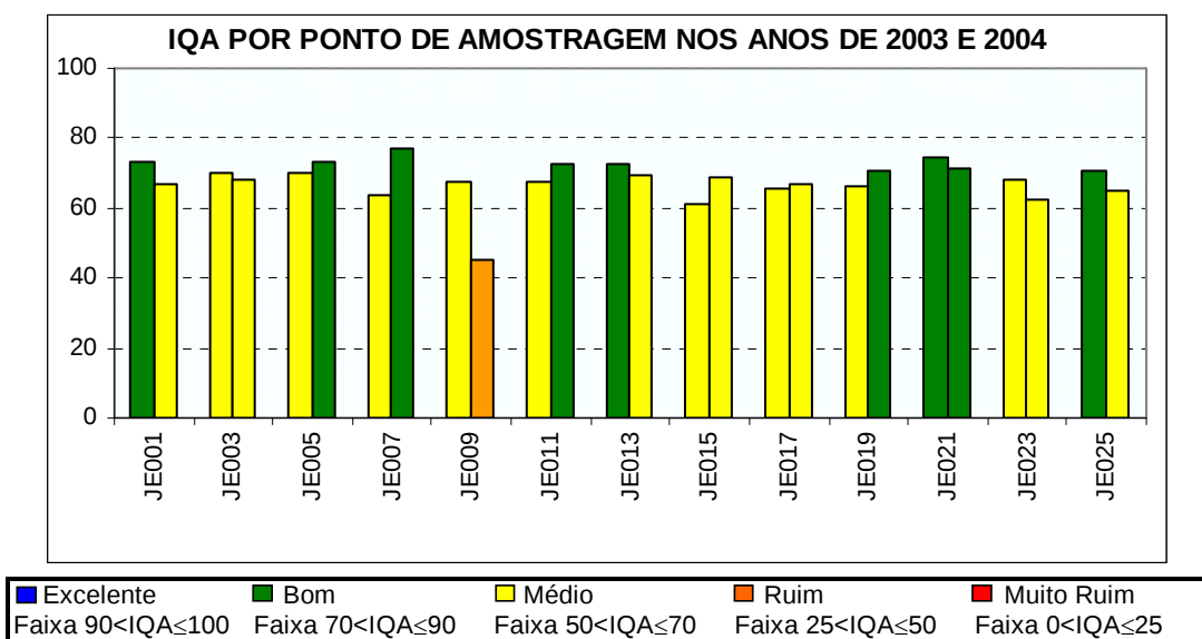
Figura 7.11: IQA médio dos anos 2003 e 2004, respectivamente, por estação de amostragem – UGRHs JQ1, JQ2 e JQ3
