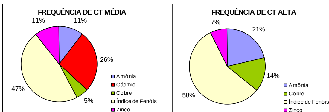
Figura 7.19: Frequência da ocorrência de parâmetros, responsáveis pela Contaminação por Tóxicos Alta e Média – UPRHs SF6, SF7, SF8, SF9 e SF10
