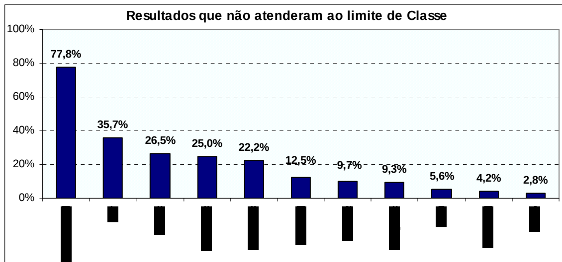
Figura 7.35: Frequência da ocorrência de parâmetros fora dos limites estabelecidos na legislação – UGRHs PN1, PN2 e PN3
