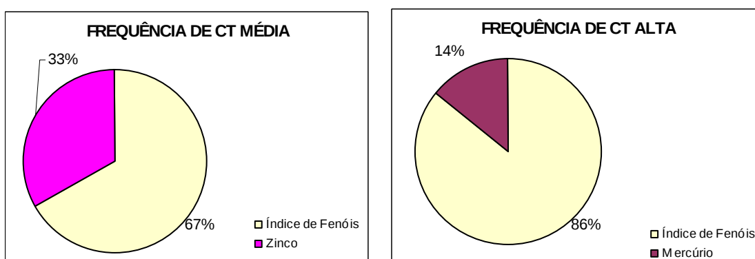
Figura 7.18: Frequência da ocorrência de parâmetros, responsáveis pela Contaminação por Tóxicos Alta e Média – UPRHs SF1 e SF4
