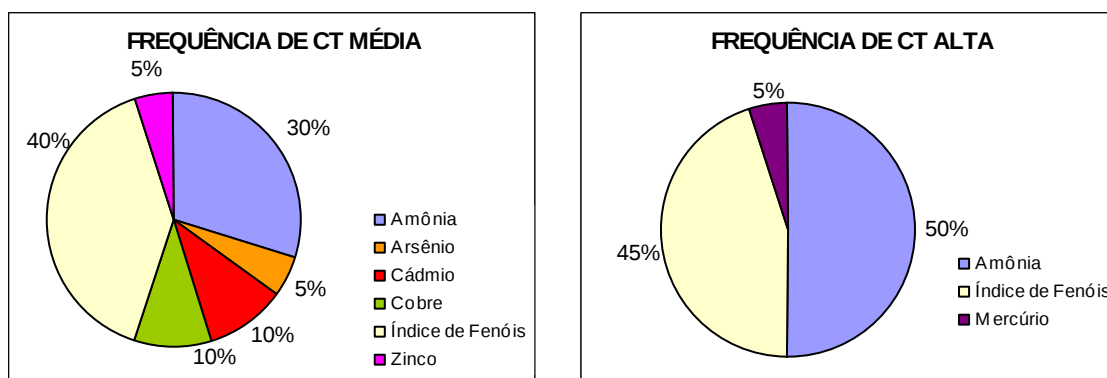
Figura 7.15: Frequência da ocorrência de parâmetros, responsáveis pela Contaminação por Tóxicos Alta e Média – UPGRH SF5
