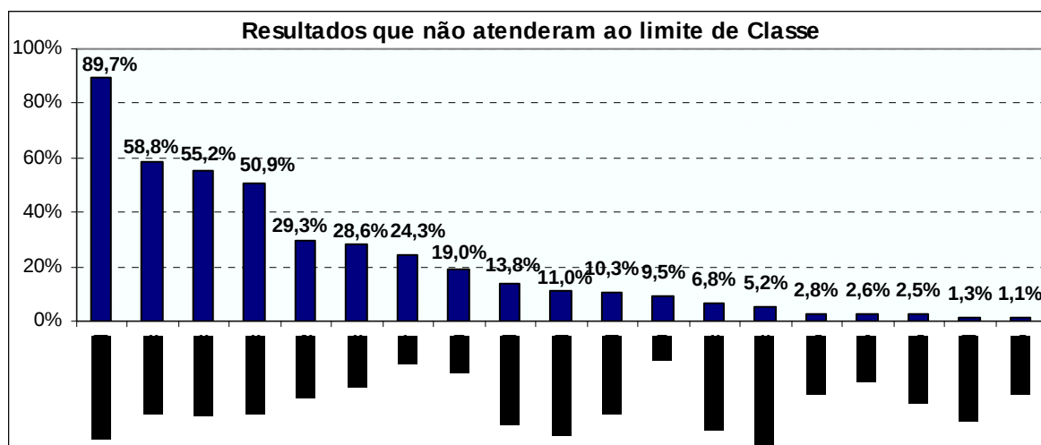
Figura 7.27: Frequência da ocorrência de parâmetros fora dos limites estabelecidos na legislação – UPGRH SF5
