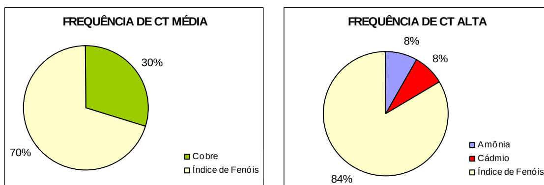
Figura 7.16: Frequência da ocorrência de parâmetros, responsáveis pela Contaminação por Tóxicos Alta e Média – UPGRH SF3
