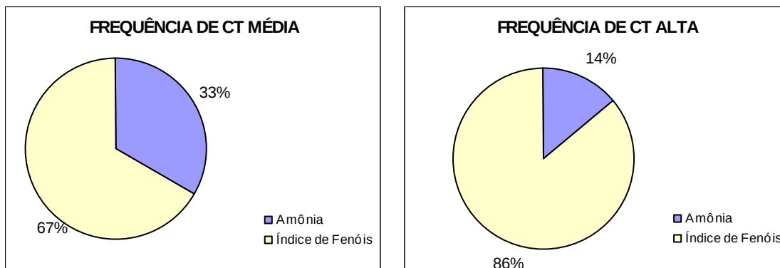
Figura 7.17: Frequência da ocorrência de parâmetros, responsáveis pela Contaminação por Tóxicos Alta e Média – UPRH SF2
