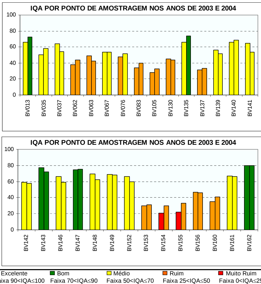
Figura 7.2: IQA médio dos anos 2003 e 2004, respectivamente, por estação de amostragem – UPGRH SF5
