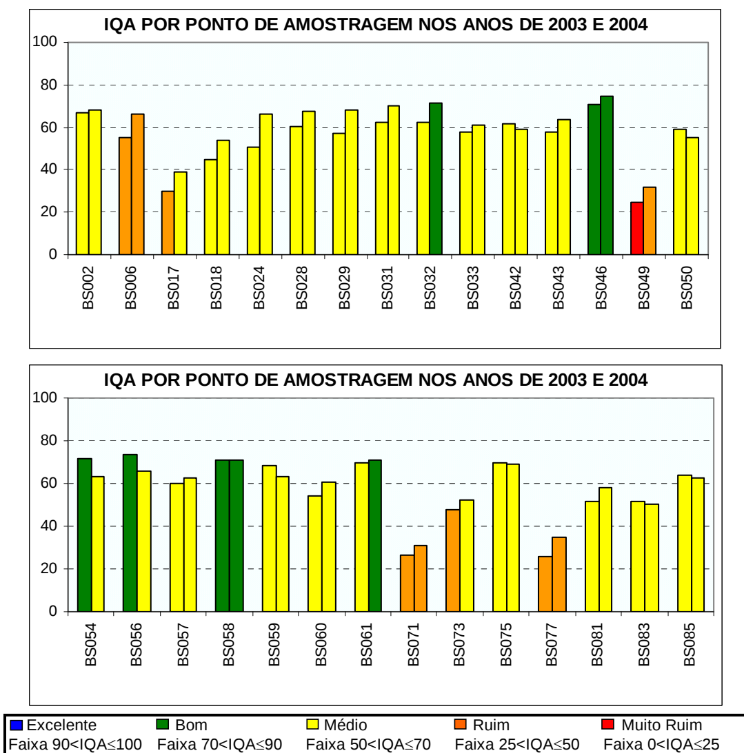
Figura 7.9: IQA médio dos anos 2003 e 2004, respectivamente, por estação de amostragem – UPGRHs PS1 e PS2
