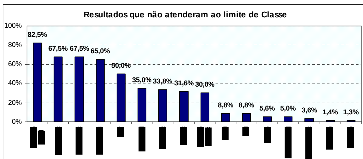
Figura 7.28: Frequência da ocorrência de parâmetros fora dos limites estabelecidos na legislação – UPGRH SF3
