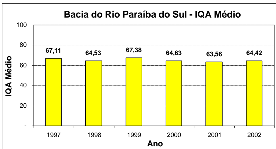
Figura 9.1: Evolução Temporal do IQA Médio na Bacia do Rio Paraíba do Sul.
