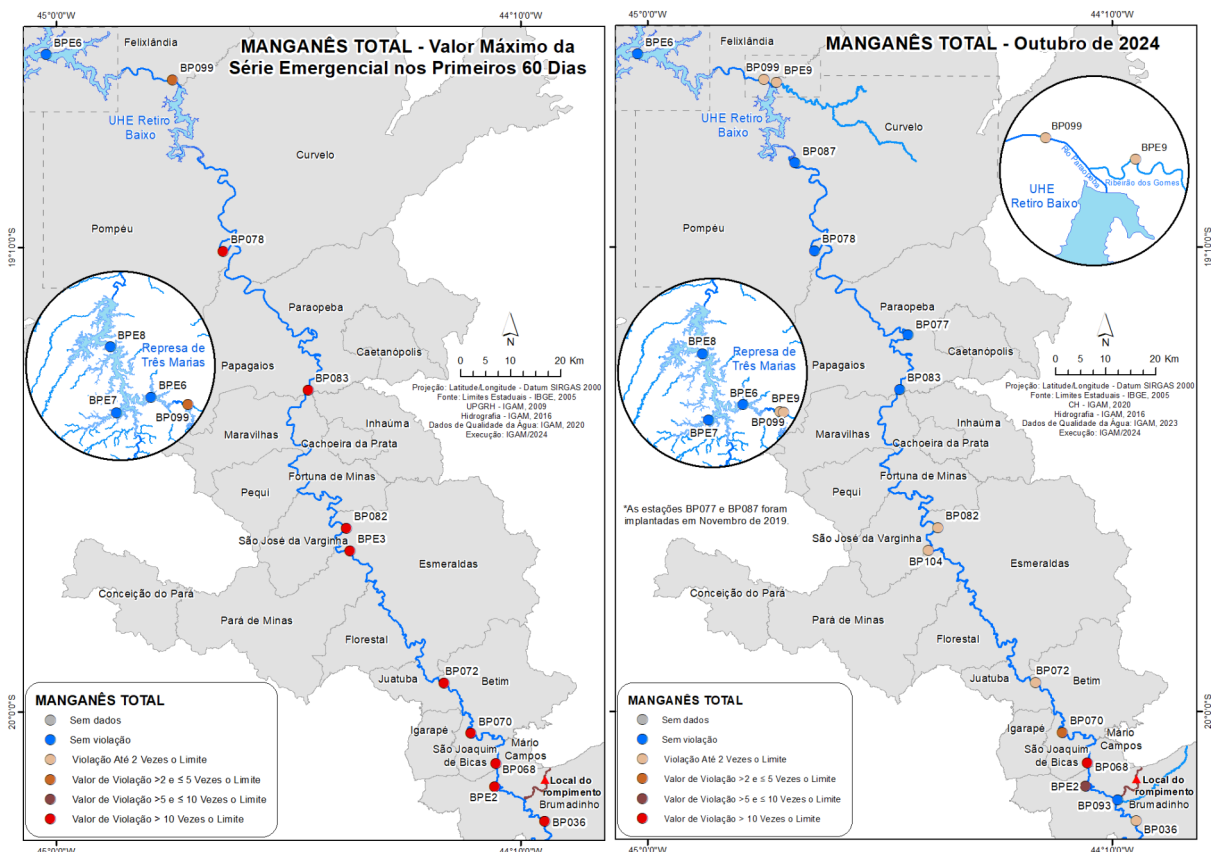
Figura 10 - Resultados de manganês total para cada estação de monitoramento nos primeiros 60 dias após o rompimento da B-I e os resultados do mês de setembro de 2024
