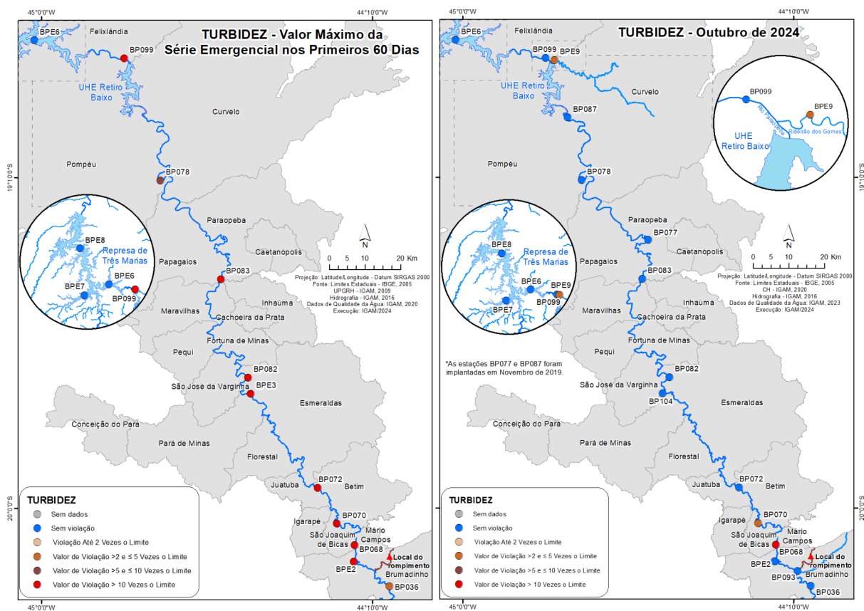
Figura 8 - Resultados dos valores máximos de turbidez para cada estação de monitoramento nos primeiros 60 dias após o rompimento da B-I e os resultados do mês de outubro de 2024
