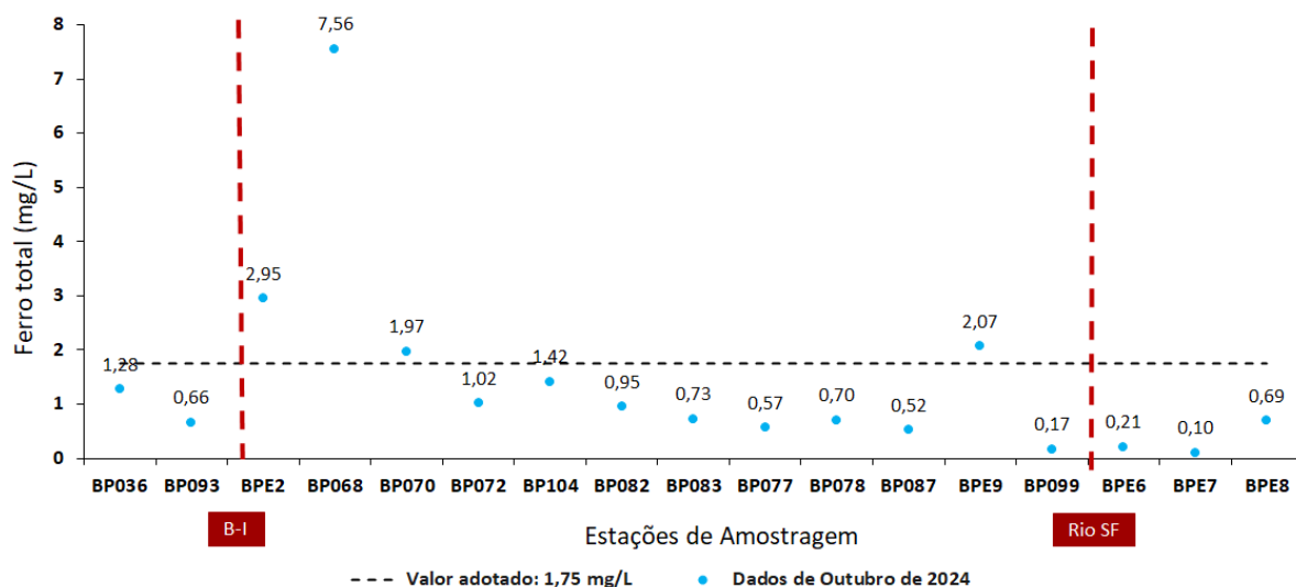
Figura 11 - Resultados de ferro total para outubro de 2024
