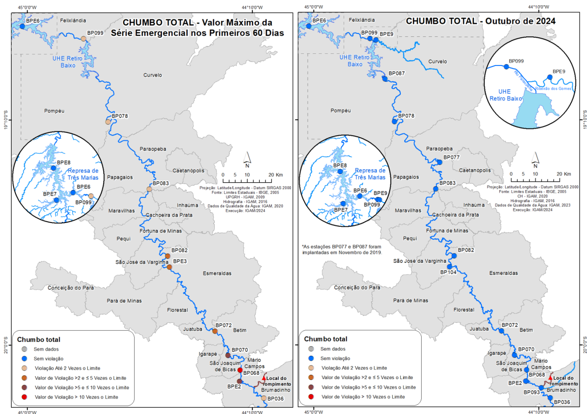
Figura 5 - Resultados dos valores máximos de chumbo total para cada estação de monitoramento nos primeiros 60 dias após o rompimento da B-I e os resultados do mês de outubro de 2024
