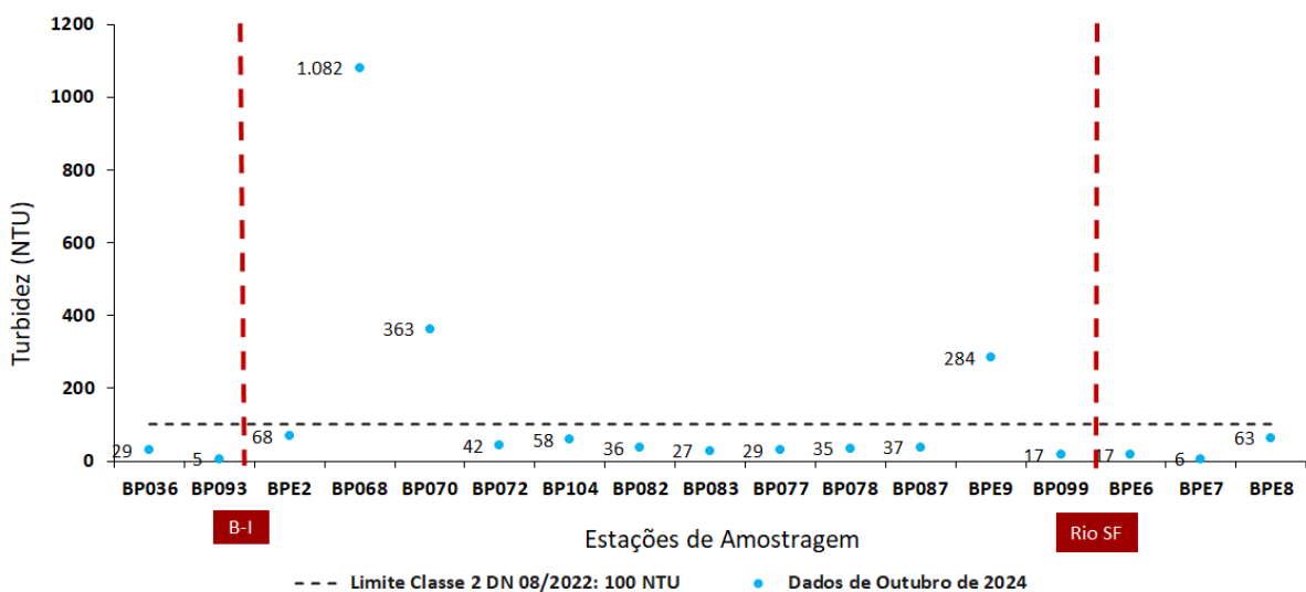
Figura 7 - Resultados de turbidez para outubro de 2024
