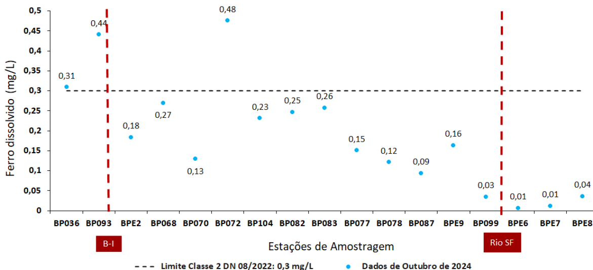
Figura 13 - Resultados de ferro dissolvido para outubro de 2024
