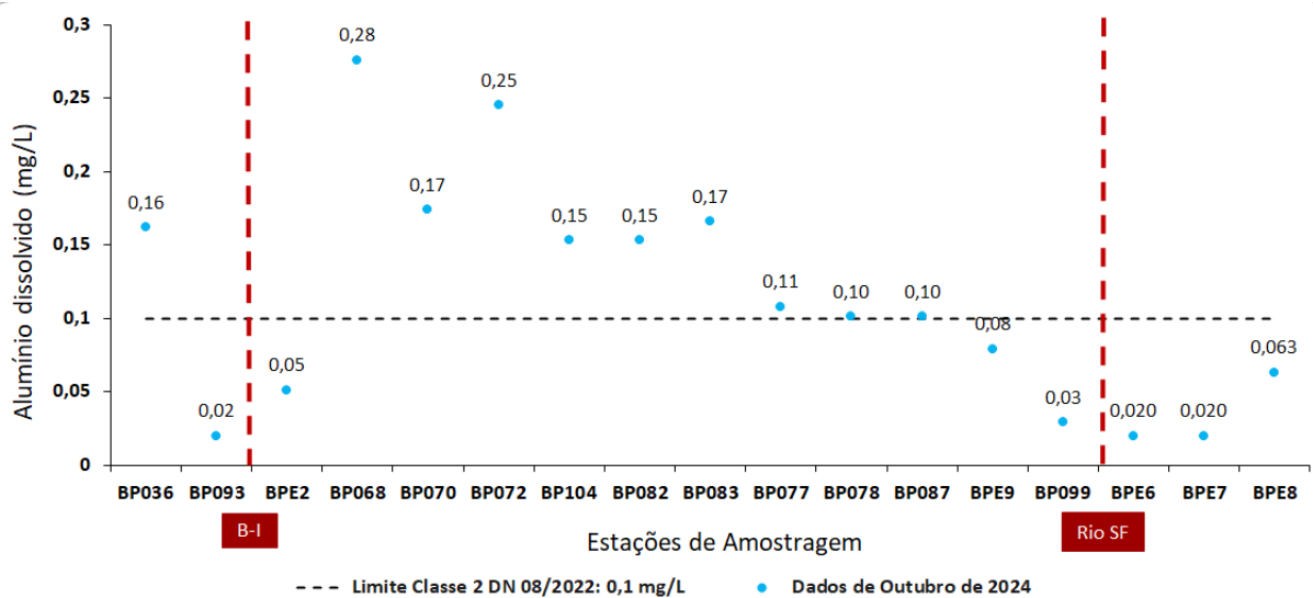
Figura 2 - Resultados de alumínio dissolvido para outubro de 2024
