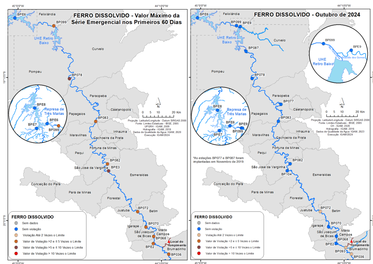
Figura 14 - Resultados dos valores máximos de ferro dissolvido para cada estação de monitoramento nos primeiros 60 dias após o rompimento da B-I e os resultados do mês de outubro de 2024
