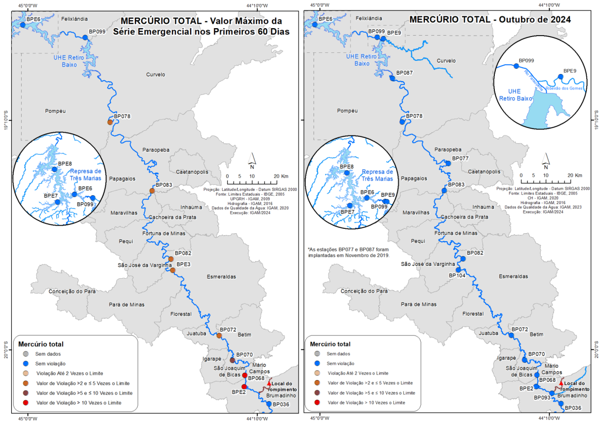
Figura 6 - Resultados dos valores máximos de mercúrio total para cada estação de monitoramento nos primeiros 60 dias após o rompimento da B-I e os resultados do mês de outubro de 2024
