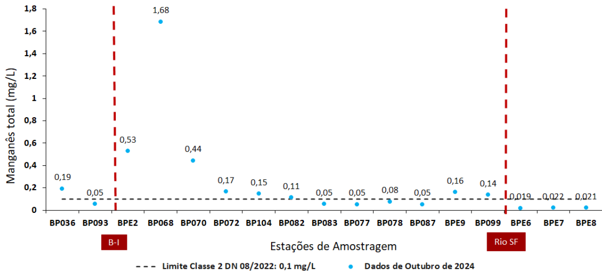
Figura 9 - Resultados de manganês total para outubro de 2024
