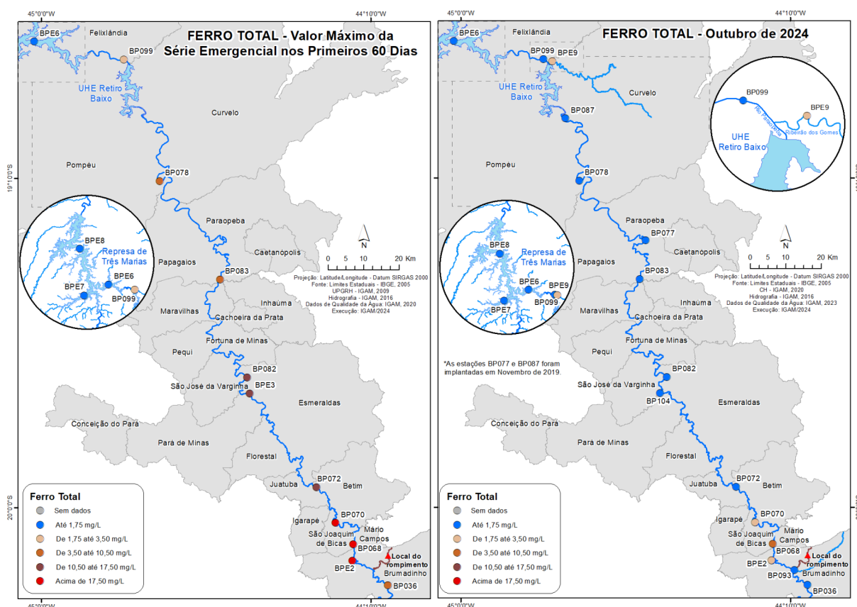
Figura 12 - Resultados dos valores máximos de ferro total para cada estação de monitoramento nos primeiros 60 dias após o rompimento da B-I e os resultados do mês de outubro de 2024
