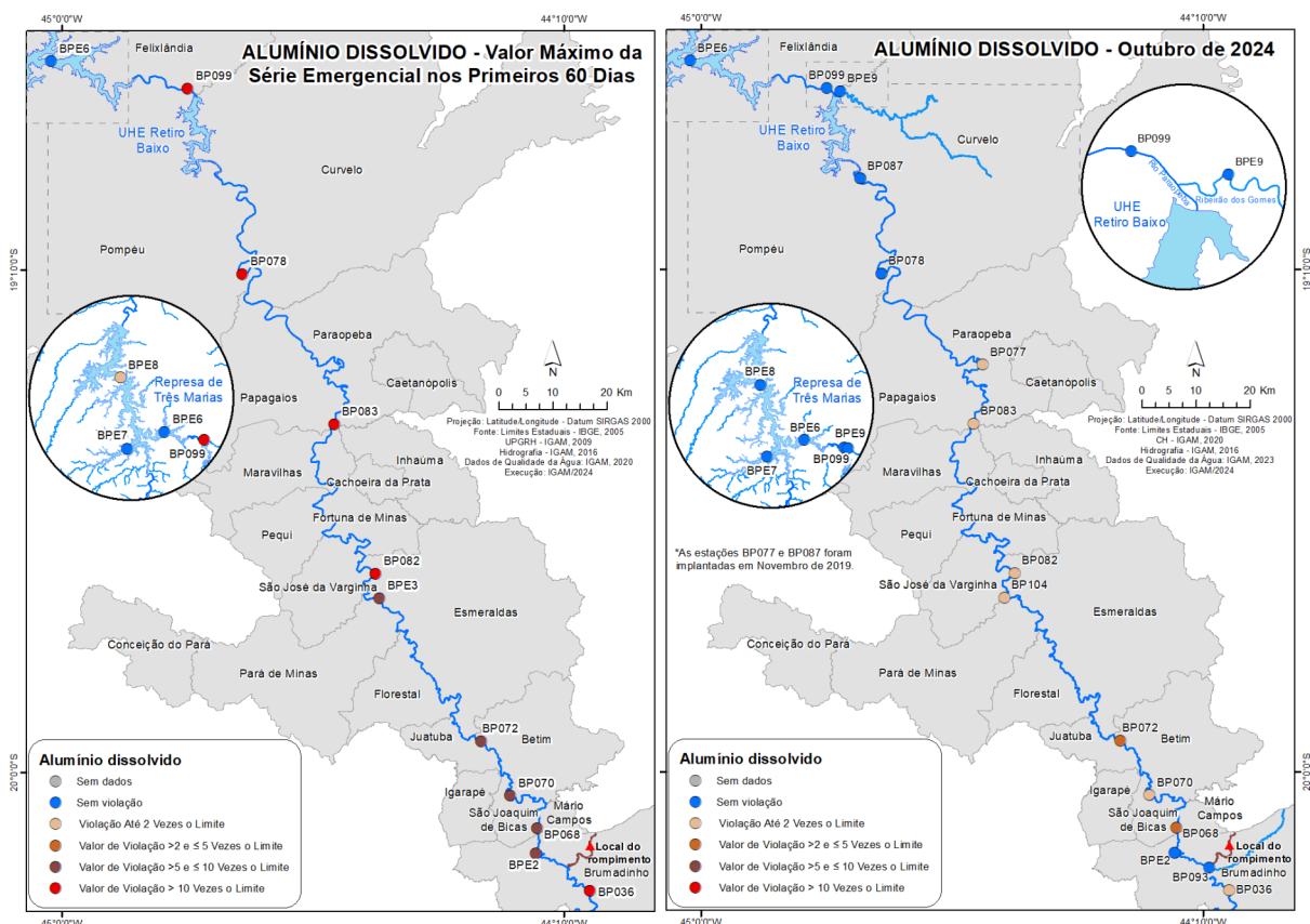
Figura 3 - Resultados dos valores máximos de alumínio dissolvido para cada estação de monitoramento nos primeiros 60 dias após o rompimento da B-I e os resultados do mês de outubro de 2024
