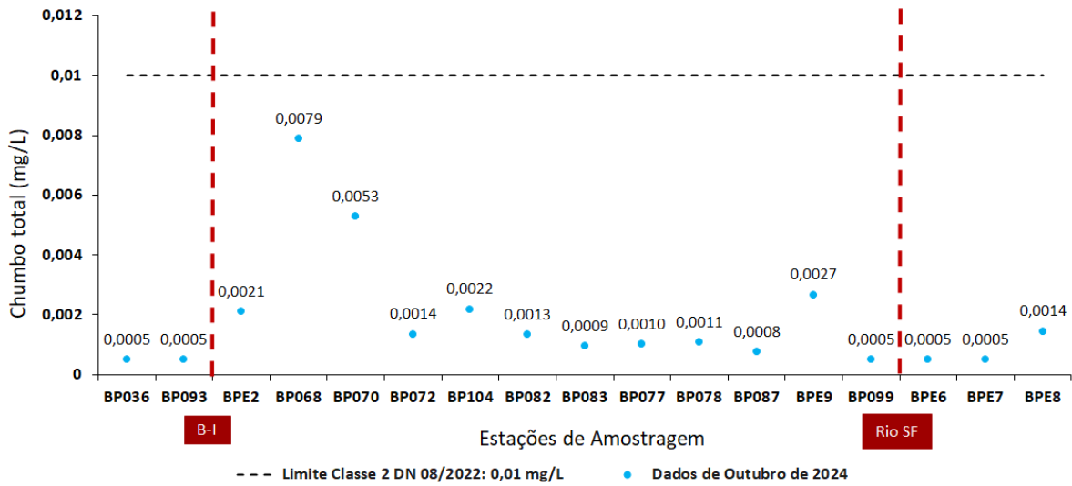
Figura 4 - Resultados de chumbo total para outubro de 2024
