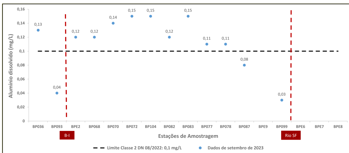
Figura 2 - Resultados de alumínio dissolvido para setembro de 2023
