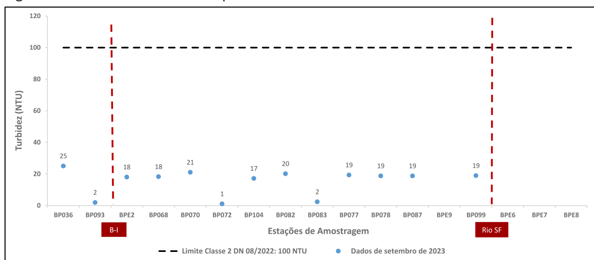
Figura 6 - Resultados de turbidez para setembro de 2023
