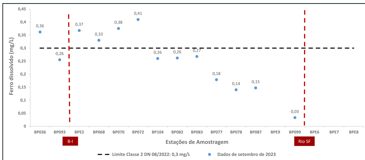
Figura 12 - Resultados de ferro dissolvido para setembro de 2023
