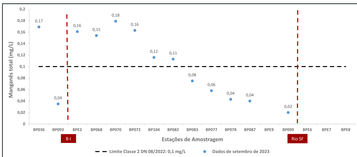
Figura 8 - Resultados de manganês total para setembro de 2023
