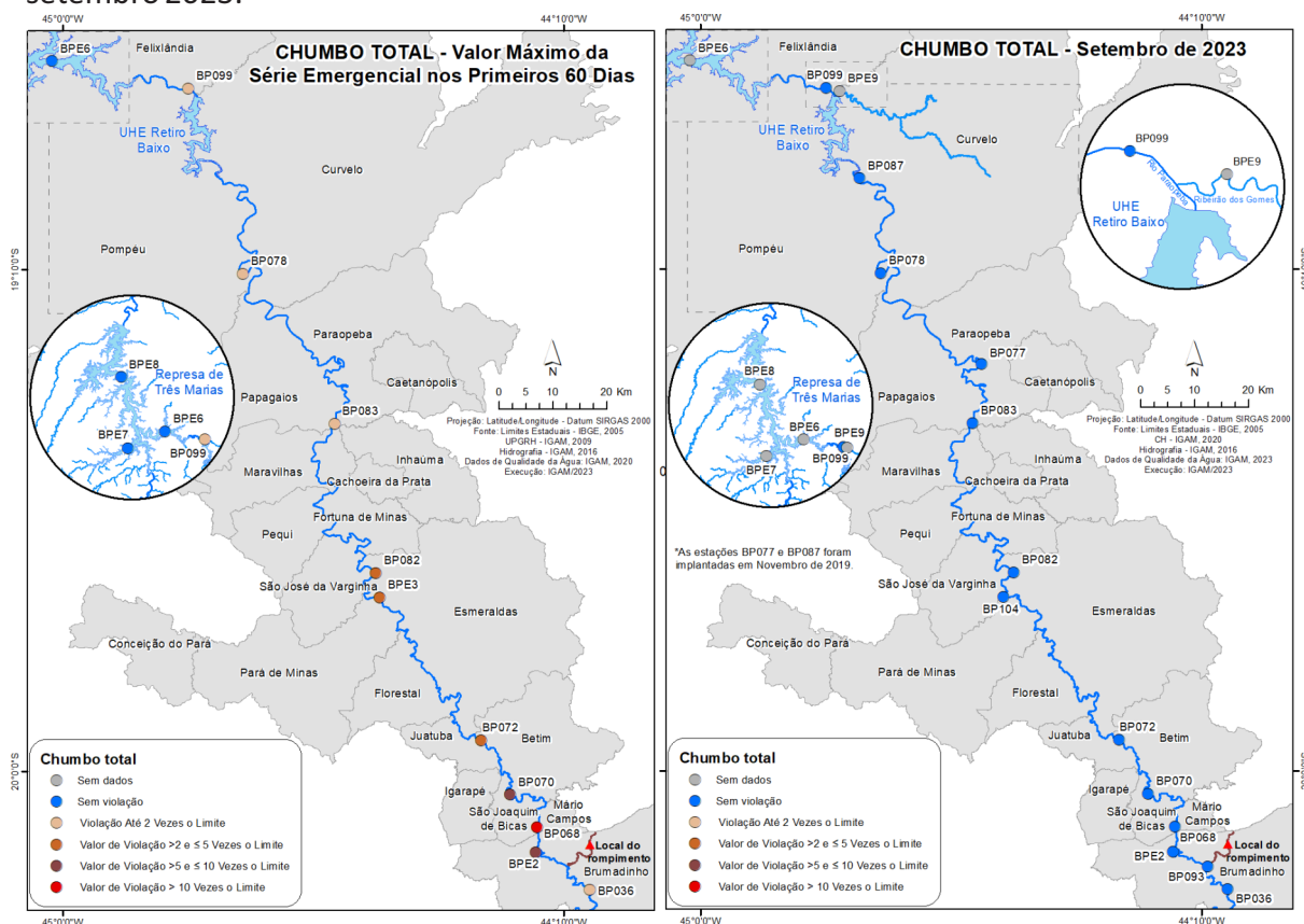
Figura 4 - Resultados dos valores máximos de chumbo total para cada estação de monitoramento nos primeiros 60 dias após o rompimento da B-I e os resultados do mês de setembro 2023.
