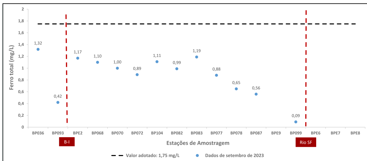
Figura 10 - Resultados de ferro total para setembro de 2023
