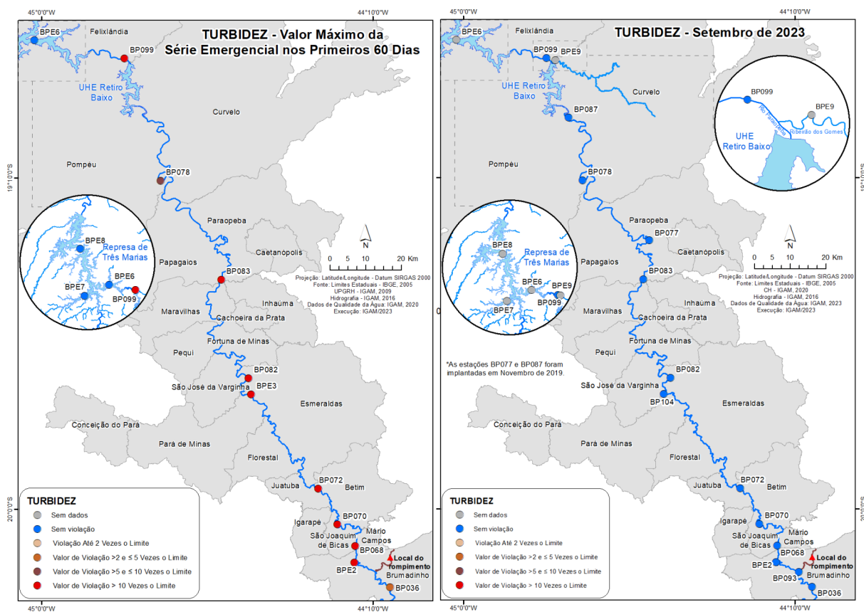
Figura 7 - Resultados dos valores máximos de turbidez para cada estação de monitoramento nos primeiros 60 dias após o rompimento da B-I e os resultados do mês de setembro 2023
