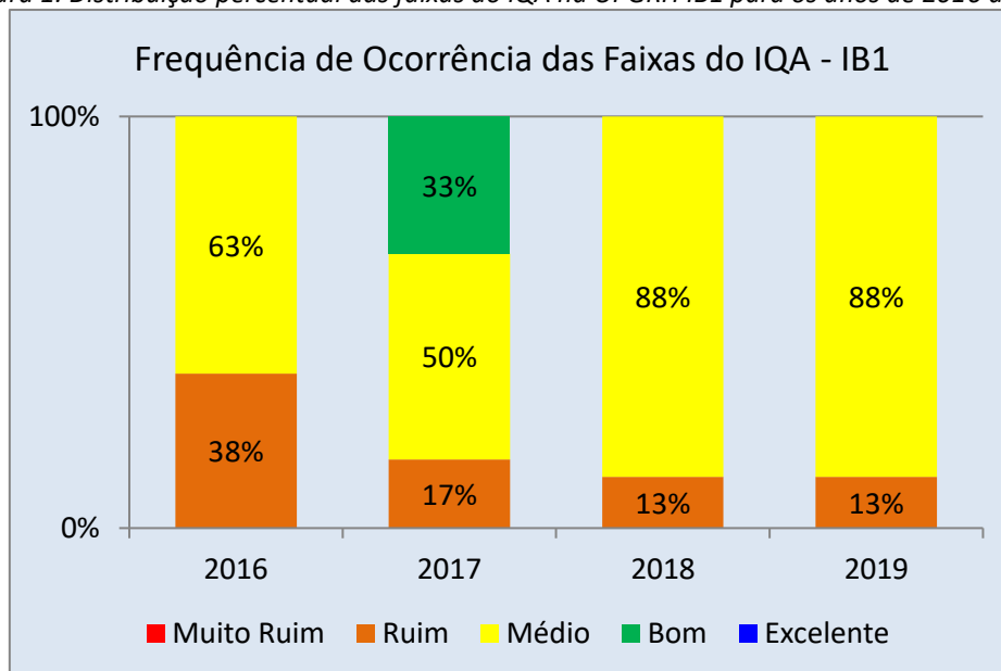
Figura 1: Distribuição percentual das faixas do IQA na UPGRH IB1 para os anos de 2016 a 2019
