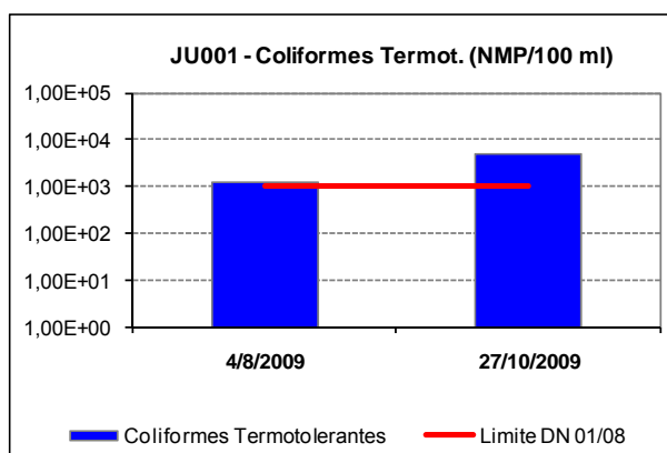
Figura 10.5: Ocorrência de coliformes termotolerantes na estação monitorada no rio Jucuruçu (Braço Norte) na cidade de Palmópolis (JU001) no ano de 2009.
