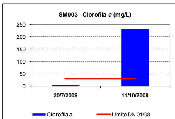
Figura 10.9: Ocorrência de clorofila-a no rio São Mateus (Braço Sul) na localidade de Barra do Ariranha (SM003) no ano de 2009.
