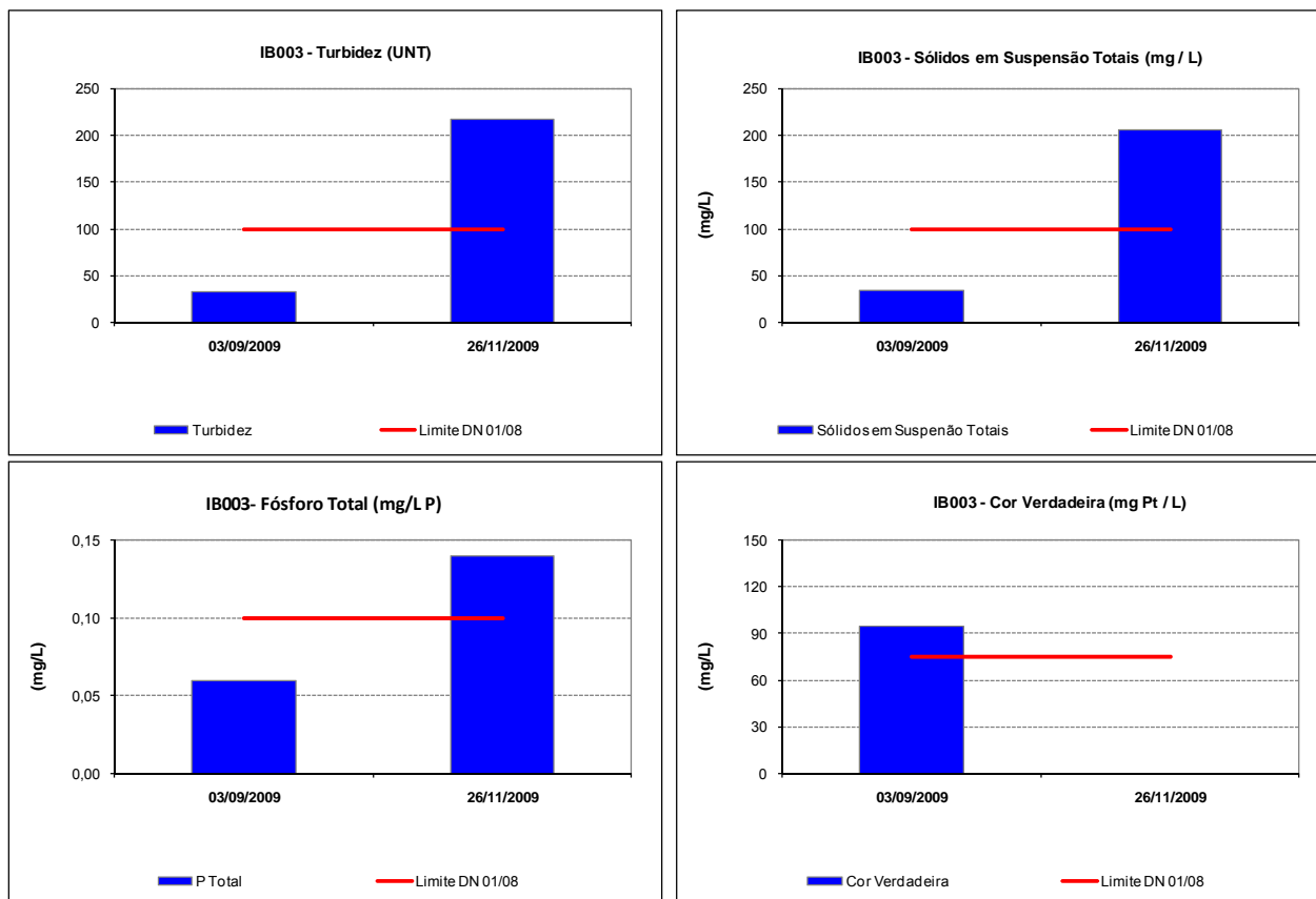
Figura 10.15: Ocorrências de turbidez, sólidos em suspensão totais, fósforo total e cor verdadeira na estação monitorada no rio São João na cidade de Caiana (IB003) no ano de 2009.
