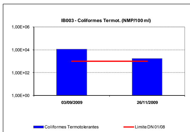
Figura 10.14: Ocorrência de coliformes termotolerantes na estação monitorada no rio São João na cidade de Caiana (IB003) no ano de 2009.
