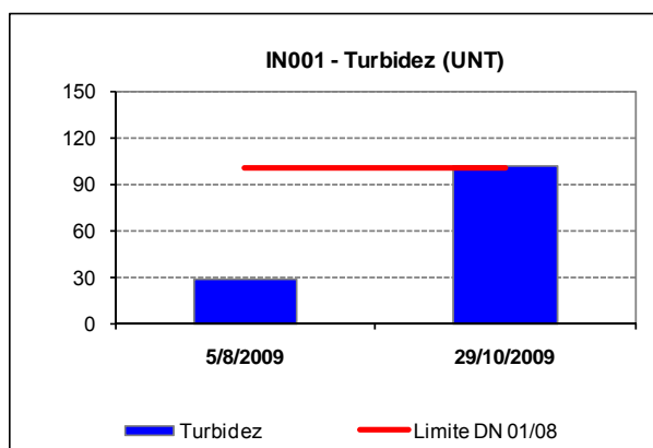
Figura 10.4: Ocorrência de turbidez na estação monitorada no rio Itanhém na cidade de Umburatiba (IN001) no ano de 2009.
