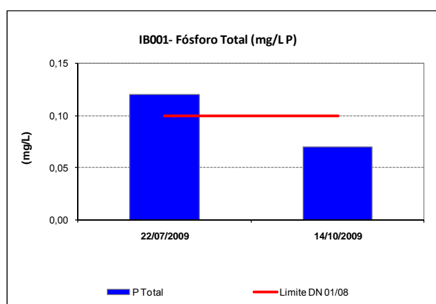
Figura 10.13: Ocorrência de fósforo total na estação monitorada no rio Caparaó na cidade de Alto Caparaó (IB001) no ano de 2009.
