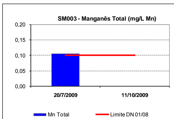
Figura 10.11: Ocorrências de manganês total no rio São Mateus (Braço Sul) na localidade de Barra do Ariranha (SM003) no ano de 2009.
