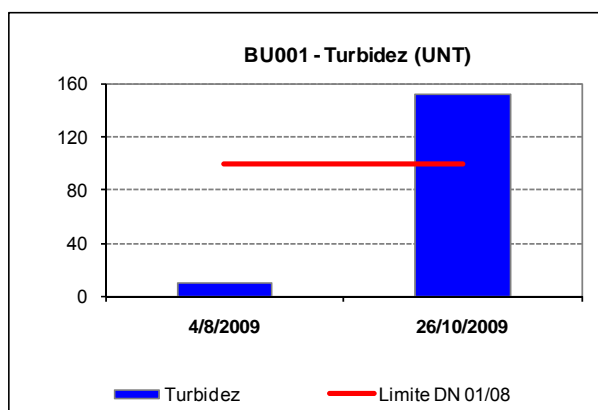
Figura 10.2: Ocorrência de turbidez na estação monitorada no rio Buranhém a jusante da cidade de Santo Antônio do Jacinto (BU001) no ano de 2009.
