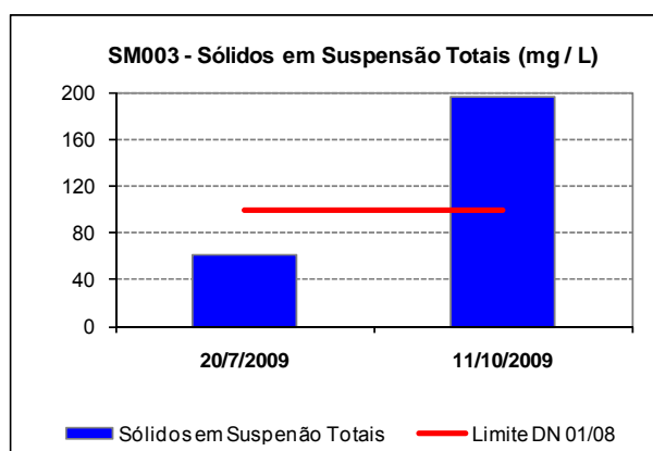
Figura 10.8: Ocorrência de sólidos em suspensão totais no rio São Mateus (Braço Sul) na localidade de Barra do Ariranha (SM003) no ano de 2009.
