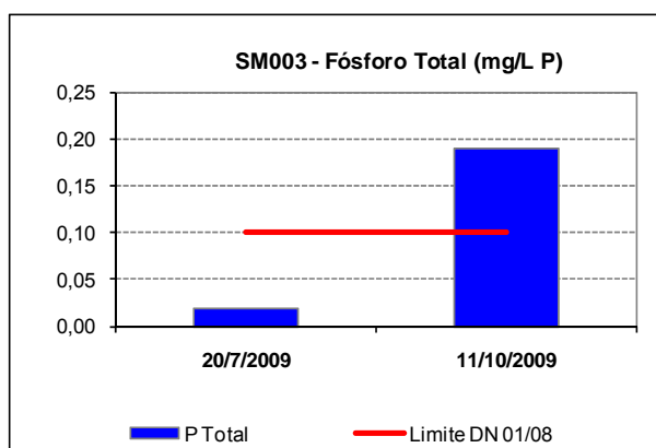
Figura 10.7: Ocorrência de fósforo total no rio São Mateus (Braço Sul) na localidade de Barra do Ariranha (SM003) no ano de 2009.
