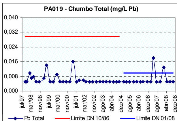
Figura 10.7: Ocorrência de chumbo total na estação de amostragem no rio Pará a montante de sua foz no rio São Francisco (PA019) no período de 1997 a 2008.
