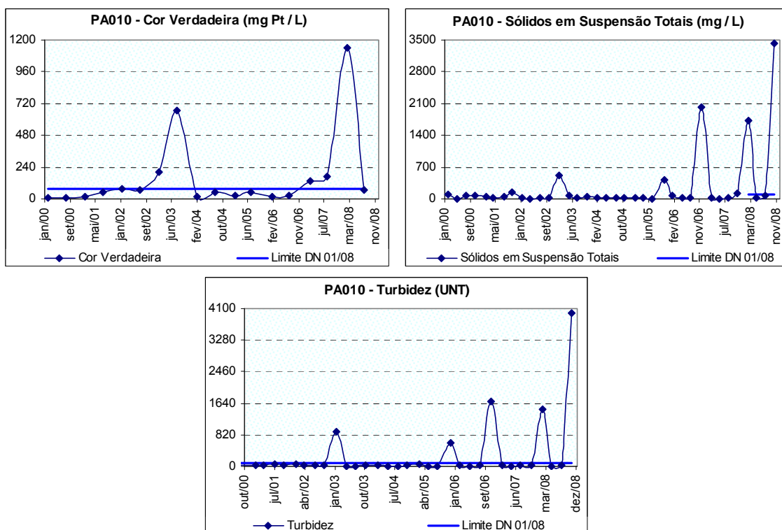
Figura 10.38: Alterações em cor verdadeira, turbidez e sólidos em suspensão totais no ribeirão Paciência a jusante de Pará de Minas (PA010) no período de 2000 a 2008.
