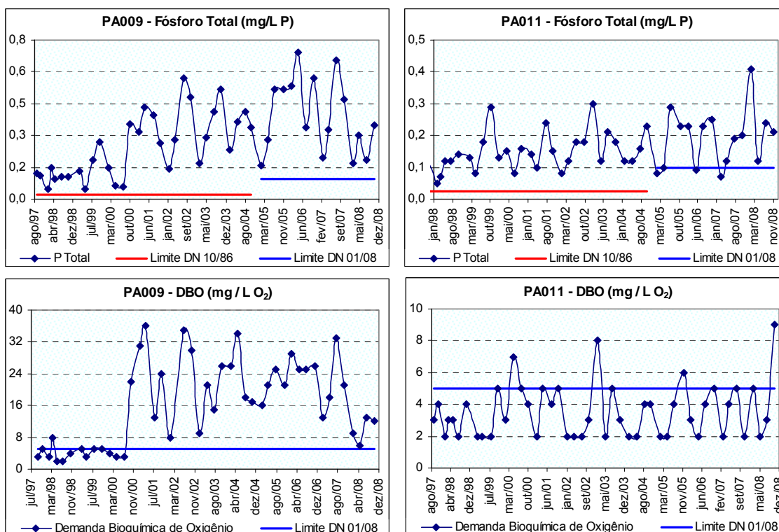
Figura 10.32: Ocorrência de fósforo total e DBO no rio São João a jusante do município de Itaúna (PA009) e próximo de sua foz no rio Pará (PA011), no período de monitoramento.
