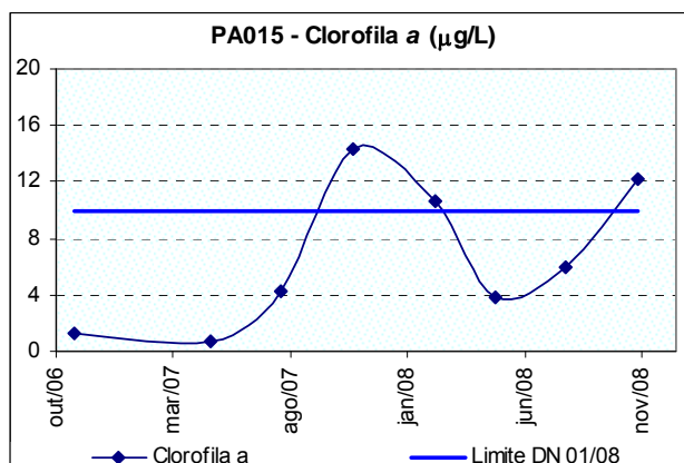
Figura 10.43: Ocorrência de clorofila-a no rio Lambari próximo de sua foz no rio Pará (PA015) no período de monitoramento.
