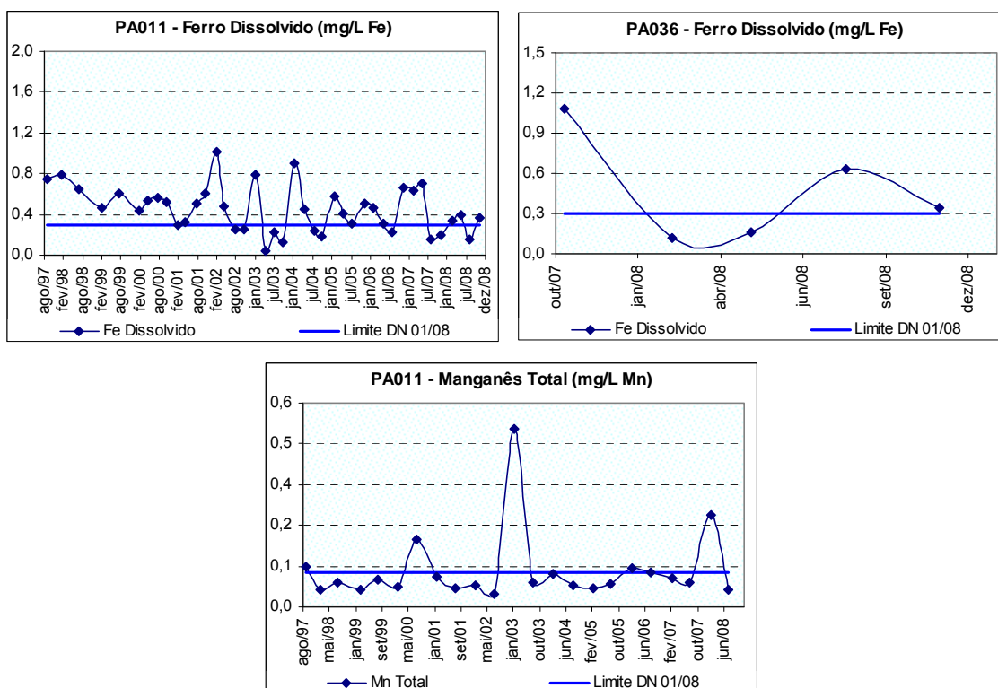
Figura 10.33: Ocorrência de ferro dissolvido no rio São João próximo à sua foz no rio Pará (PA011) e no rio São João na localidade de São João (PA036), manganês total no rio São João próximo à sua foz no rio Pará (PA011) no período de monitoramento.
