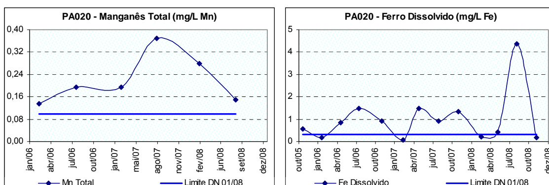
Figura 10.29: Ocorrência de manganês total e ferro dissolvido no ribeirão da Fartura ou do Gama a montante de sua foz no rio Pará no município de Nova Serrana (PA020) no período de monitoramento.
