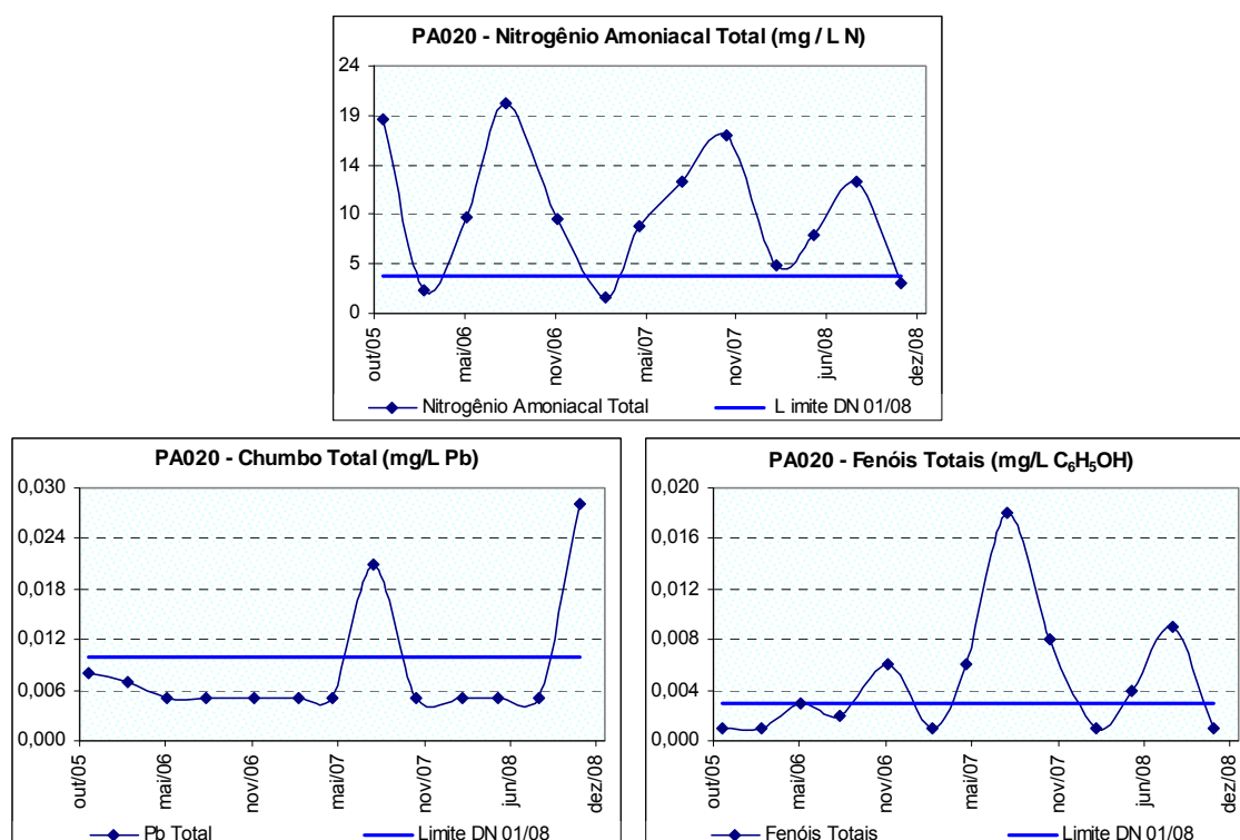
Figura 10.30: Ocorrência de nitrogênio amoniacoal total, fenóis totais e chumbo total no ribeirão da Fartura ou do Gama a montante de sua foz no rio Pará no município de Nova Serrana (PA020) no período de 2005 a 2008.
