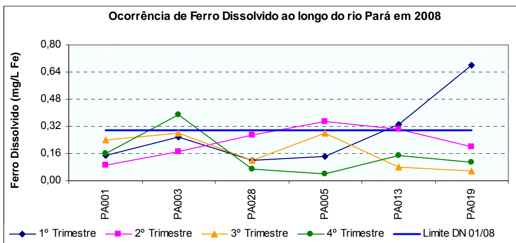
Figura 10.6: Ocorrência de ferro dissolvido ao longo do rio Pará no ano de 2008.
