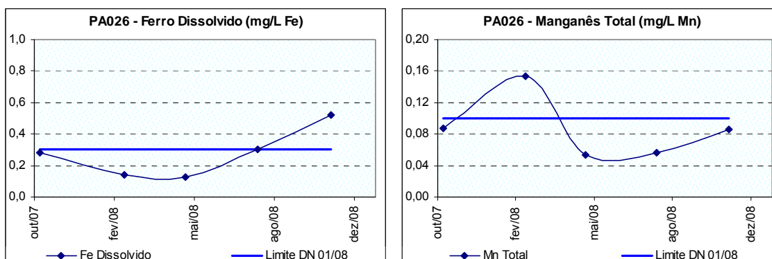
Figura 10.13: Ocorrência de ferro dissolvido e manganês total no rio do Peixe a montante do município de Piracema (PA026), no período de monitoramento.
