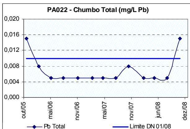
Figura 10.48: Ocorrência de chumbo total no ribeirão Diamante a jusante da cidade de Santo Antônio do Monte (PA022) no período de 2005 a 2008.
