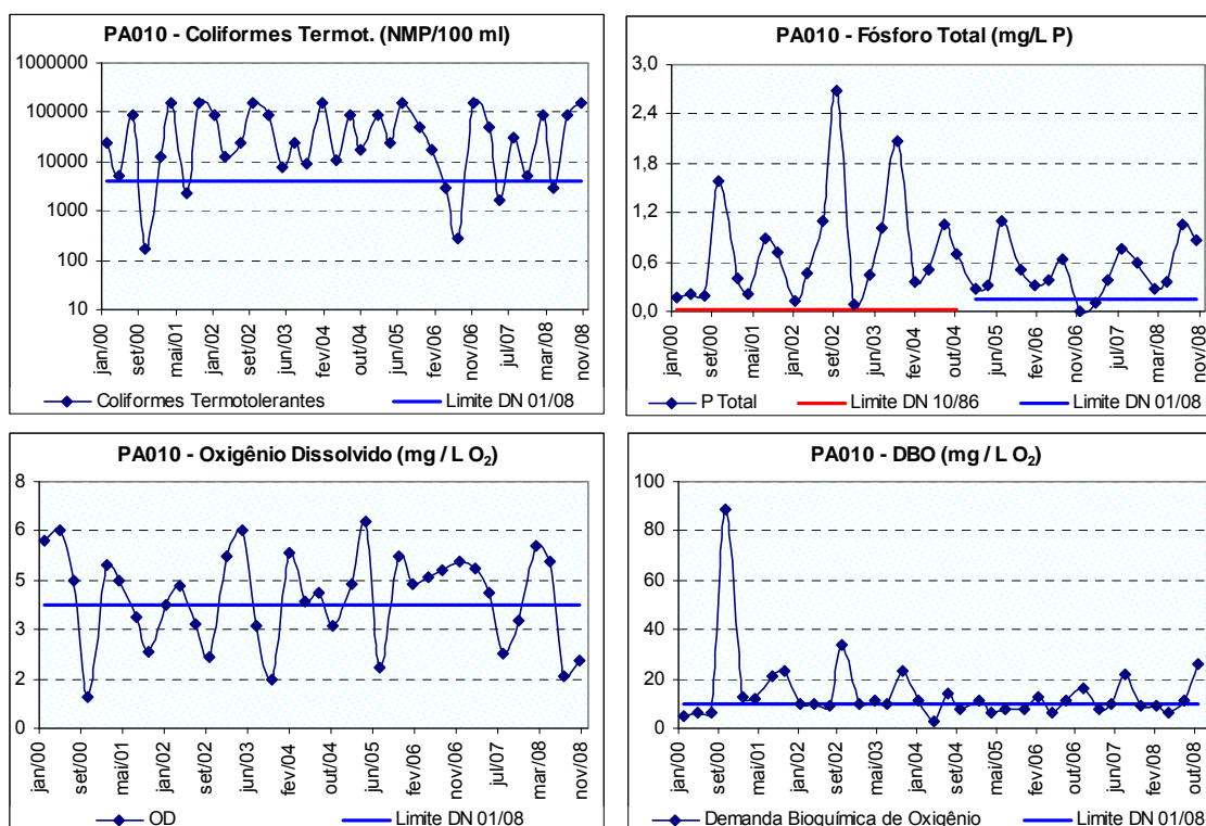
Figura 10.37: Ocorrência de coliformes termotolerantes, fósforo total, OD e DBO no ribeirão Paciência a jusante de Pará de Minas (PA010) no período de 2000 a 2008.
