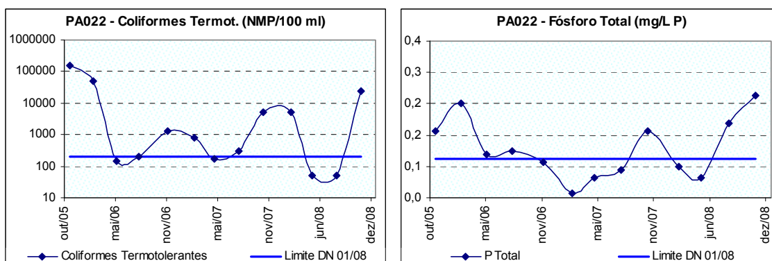
Figura 10.45: Ocorrência de coliformes termotolerantes e fósforo total no ribeirão Diamante a jusante da cidade de Santo Antônio do Monte (PA022), no período de 2005 a 2008.
