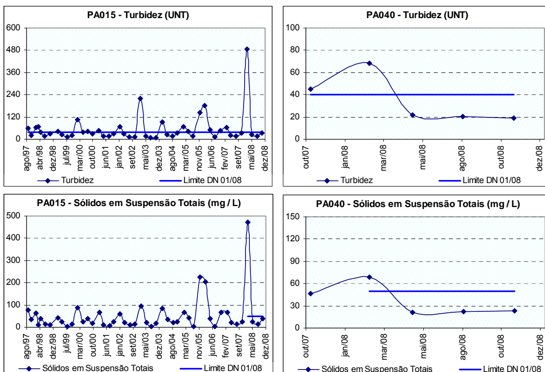
Figura 10.41: Ocorrência de turbidez e sólidos em suspensão totais no rio Lambari próximo de sua foz no rio Pará (PA015) e do rio Lambari no município de Pedra do Indaiá (PA040) no período de monitoramento.
