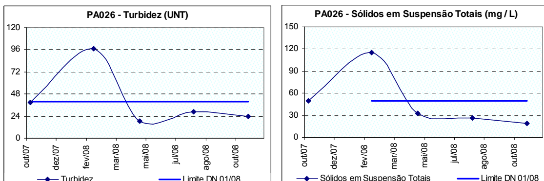
Figura 10.11: Ocorrência de turbidez e sólidos em suspensão totais no rio do Peixe a montante do município de Piracema (PA026) no período de monitoramento.
