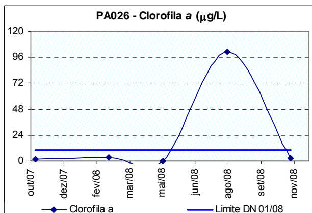
Figura 10.12: Ocorrência de clorofila-a no rio do Peixe a montante do município de Piracema (PA026) no período de monitoramento.
