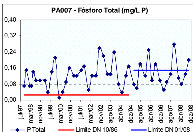
Figura 10.17: Ocorrência de fósforo total no rio Itapecerica a jusante da cidade de Divinópolis (PA007) no período de 1997 a 2008.
