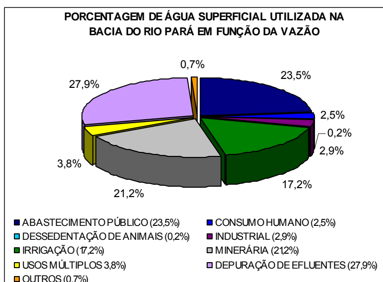
Figura 9.3: Porcentagem de água superficial utilizada na sub-bacia do rio Pará em 2008, em função da vazão outorgada.
