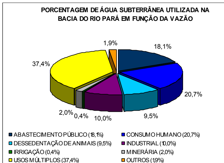
Figura 9.4: Porcentagem de água subterrânea utilizada na sub-bacia do rio Pará em 2008, em função da vazão outorgada.
