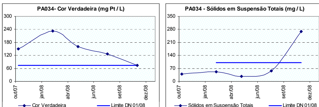
Figura 10.23: Ocorrência de cor verdadeira e sólidos em suspensão totais no córrego do Pinto ou Buriti a jusante do município de São Gonçalo do Pará (PA034) no período de monitoramento.
