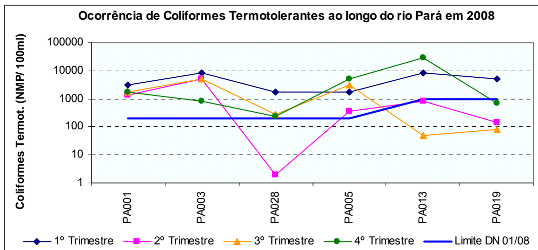
Figura 10.2: Ocorrência de coliformes termotolerantes ao longo do rio Pará, no ano de 2008.
