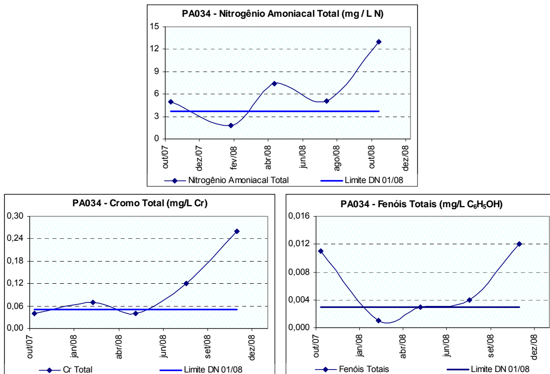
Figura 10.25: Ocorrência de nitrogênio amoniacal, cromo total e fenóis totais no córrego do Pinto ou Buriti a jusante do município de São Gonçalo do Pará (PA034), no período de monitoramento.
