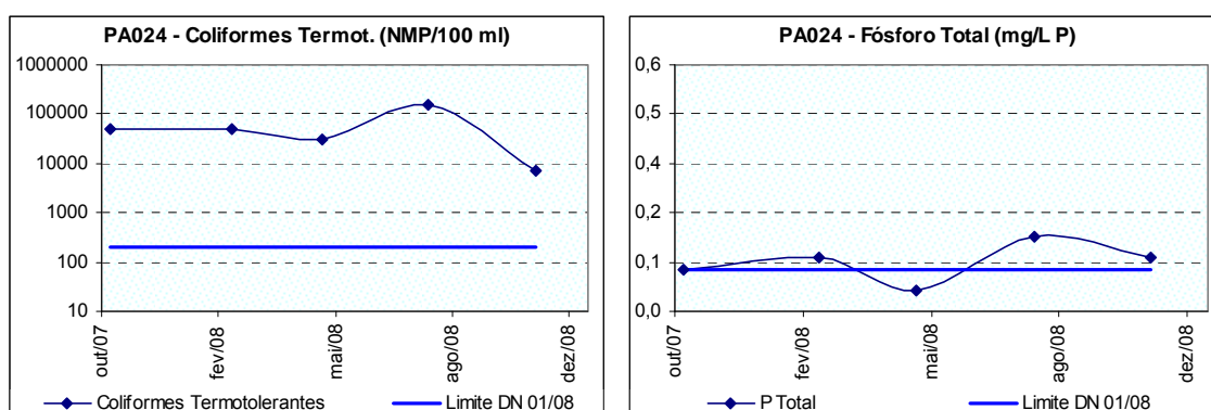
Figura 10.8: Ocorrência de coliformes termotolerantes e fósforo total na estação de amostragem localizada no ribeirão Passa Tempo na cidade de Passa Tempo (PA024) no período de monitoramento.
