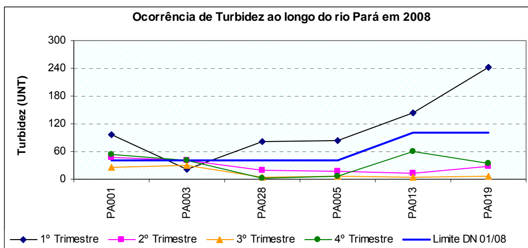
Figura 10.3: Ocorrência de turbidez ao longo do rio Pará, no ano de 2008.
