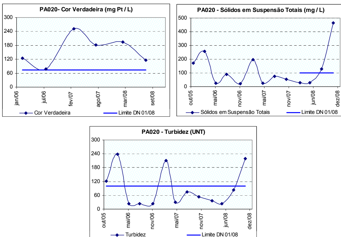
Figura 10.27: Ocorrência de cor verdadeira, sólidos em suspensão totais e turbidez no ribeirão da Fartura ou do Gama a montante de sua foz no rio Pará no município de Nova Serrana (PA020), no período de 2005 a 2008.
