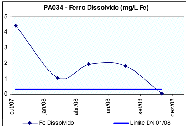
Figura 10.24: Ocorrência de ferro dissolvido no córrego do Pinto ou Buriti a jusante do município de São Gonçalo do Pará (PA034) no período de monitoramento.
