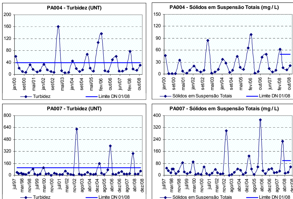
Figura 10.18: Ocorrência de turbidez e sólidos em suspensão totais no rio Itapeçerica a montante de Divinópolis (PA004) e a jusante de Divinópolis (PA007) no período de monitoramento.
