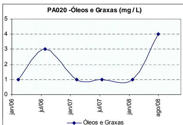
Figura 10.28: Ocorrência de óleos e graxas no ribeirão da Fartura ou do Gama a montante de sua foz no rio Pará no município de Nova Serrana (PA020) no período de 2006 a 2008.
