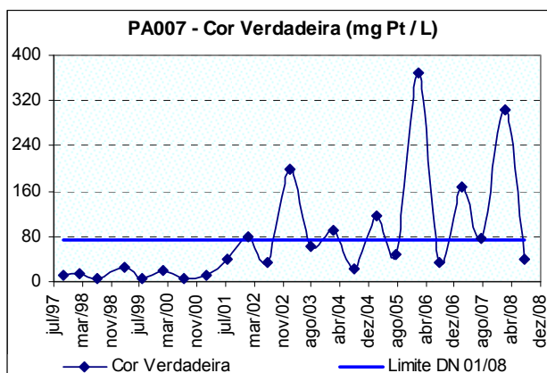
Figura 10.19: Ocorrência de cor verdadeira no rio Itapecerica a jusante da cidade de Divinópolis (PA007) no período de 1997 a 2008.
