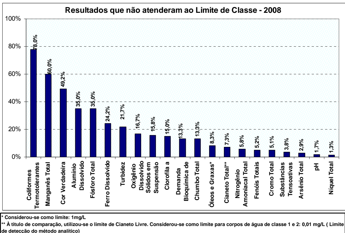
Figura 8.31: Frequência da ocorrência de parâmetros fora dos limites estabelecidos na legislação em 2008 – UPRGH SF3.
