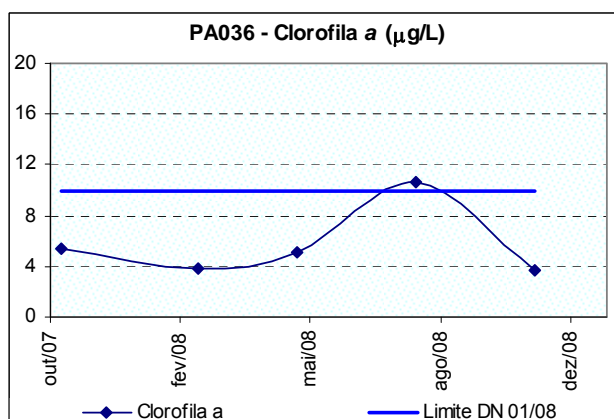
Figura 10.35: Ocorrência de clorofila-a no rio São João na localidade de São João (PA036) no período de monitoramento.
