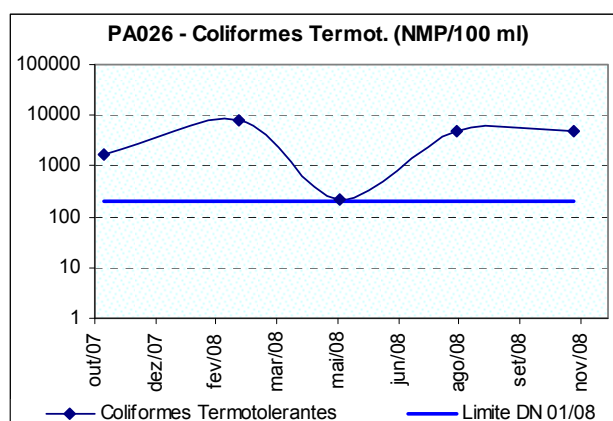
Figura 10.10: Ocorrência de coliformes termotolerantes na estação de amostragem localizada no rio do Peixe a montante do município de Piracema (PA026) no período de monitoramento.
