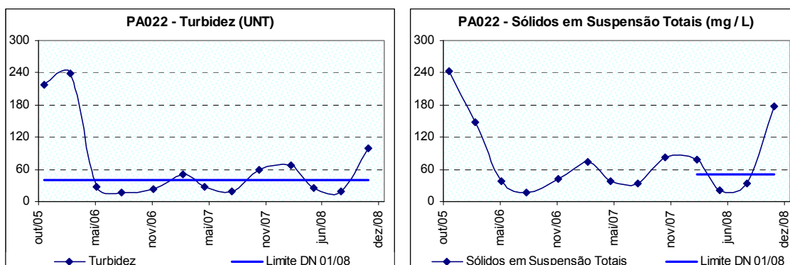
Figura 10.46: Alterações de turbidez e sólidos em suspensão totais no ribeirão Diamante a jusante da cidade de Santo Antônio do Monte (PA022) no período de 2005 a 2008.
