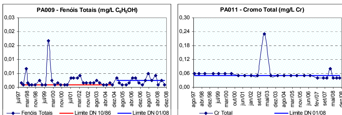
Figura 10.36: Ocorrência de fenóis totais no rio São João a jusante do município de Itaúna (PA009) e próximo à sua foz no rio Pará (PA011) e cromo total a jusante do município de Itaúna (PA009), no período de 1997 a 2008.
