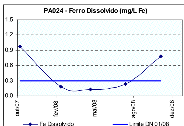
Figura 10.9: Ocorrência de ferro dissolvido na estação de amostragem localizada no ribeirão Passa Tempo na cidade de Passa Tempo (PA024) no período de monitoramento.
