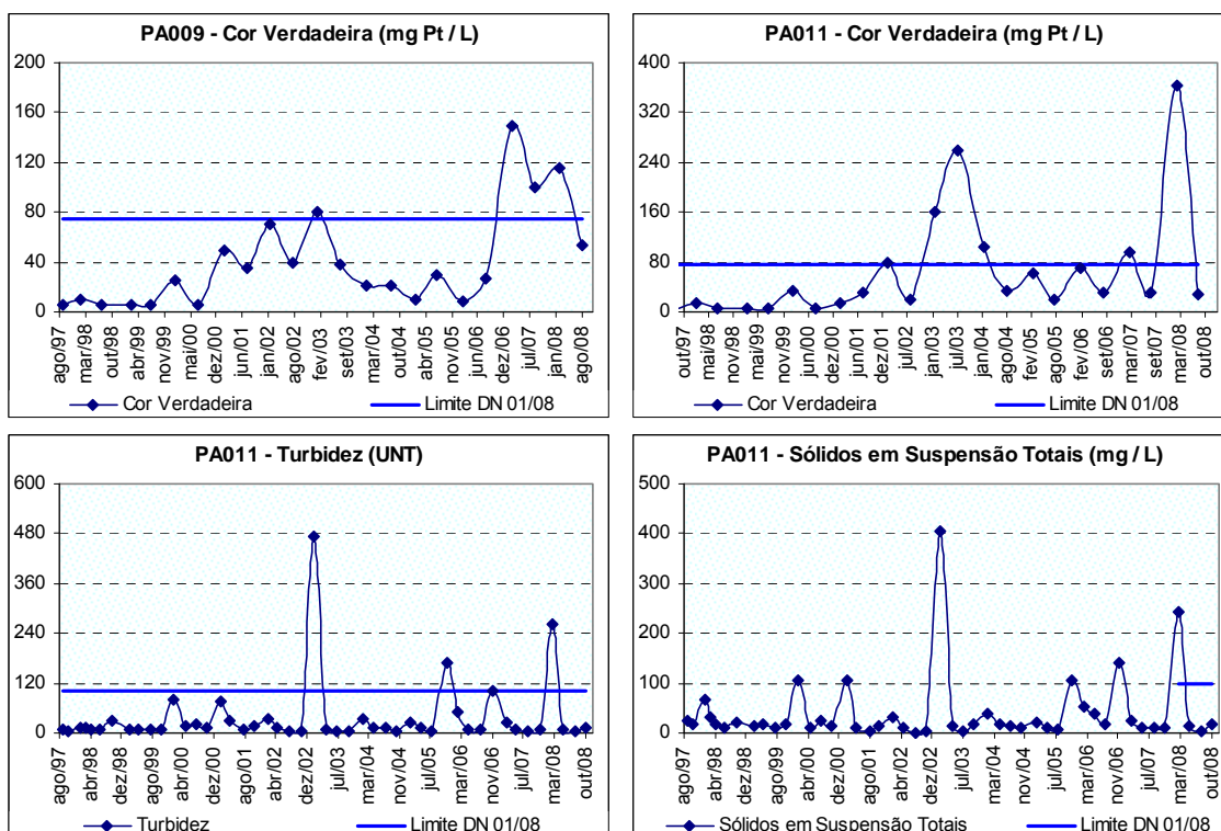
Figura 10.34: Ocorrência de cor verdadeira no rio São João a jusante do município de Itaúna (PA009) e cor verdadeira, turbidez e sólidos em suspensão totais próximo à sua foz no rio Pará (PA011) no período de 1997 a 2008.
