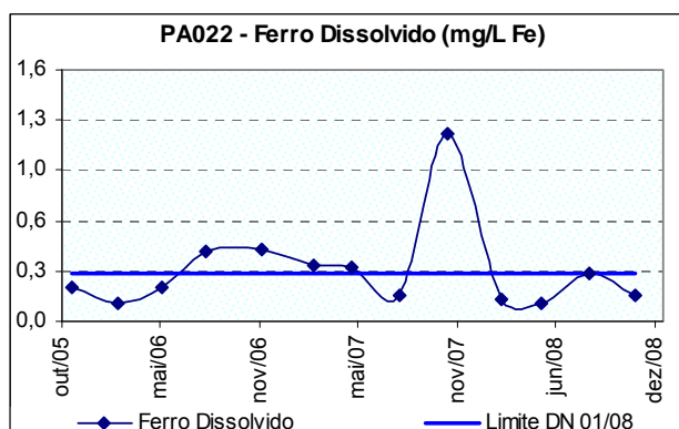
Figura 10.47: Ocorrência de ferro dissolvido no ribeirão Diamante a jusante da cidade de Santo Antônio do Monte (PA022) no período de 2005 a 2008.
