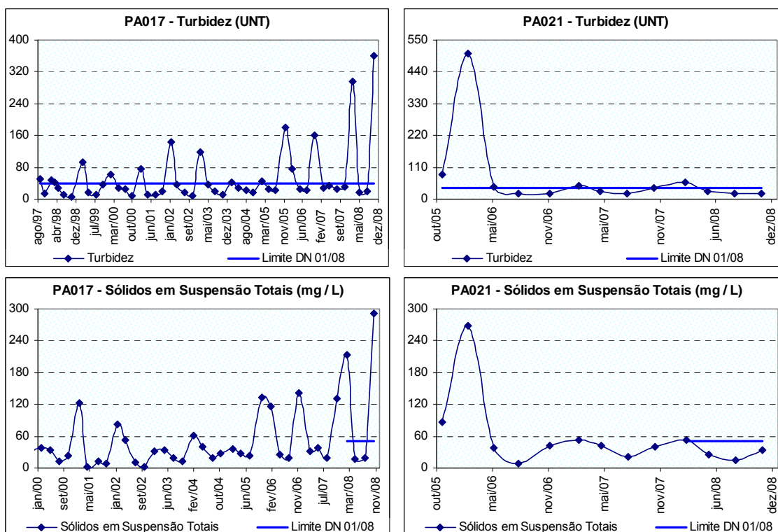
Figura 10.55: Ocorrência de turbidez e sólidos em suspensão totais no rio Picão a jusante da cidade de Bom Despacho (PA021) e no rio do Picão próximo de sua foz no rio Pará (PA017) no período de monitoramento.
