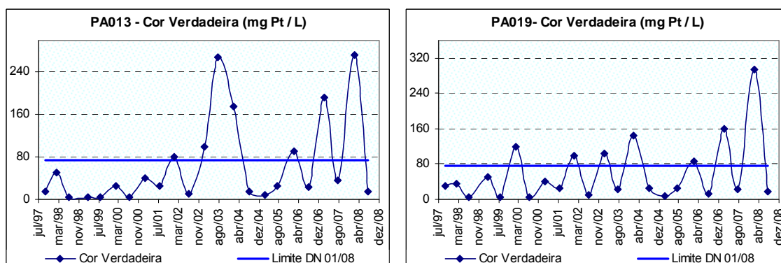
Figura 10.4: Ocorrência de cor verdadeira no rio Pará na localidade de Velho da Taipa próximo ao município de Pitangui (PA013) e a montante de sua foz no rio São Francisco (PA019) no período de 1997 a 2008.
