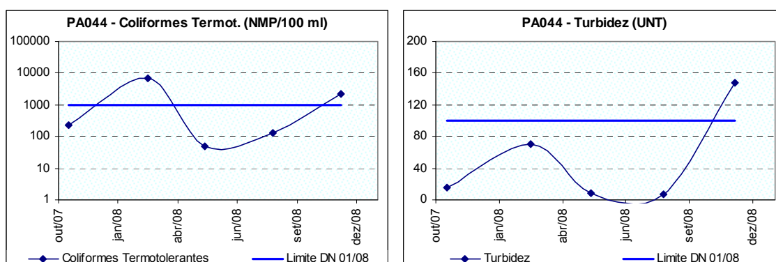
Figura 10.51: Ocorrência de coliformes termotolerantes e turbidez no Córrego Salobro a jusante do município de Pompéu (PA044) no período de monitoramento.
