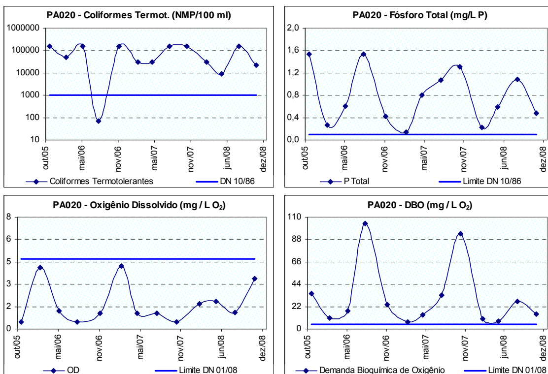
Figura 10.26: Ocorrência de coliformes termotolerantes, fósforo total, OD e DBO no ribeirão da Fartura ou do Gama a montante de sua foz no rio Pará, município de Nova Serrana (PA020) no período de 2005 a 2008.
