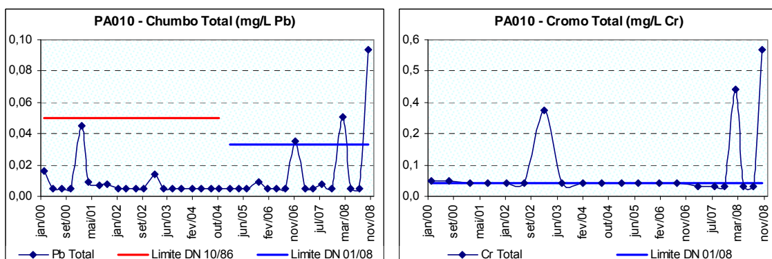
Figura 10.39: Alterações em chumbo total, cromo total no ribeirão Paciência a jusante de Pará de Minas (PA010) no período de 2000 a 2008.
