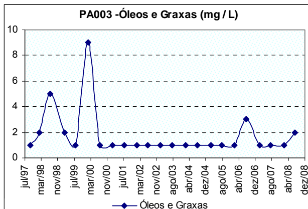
Figura 10.5: Ocorrência de óleos e graxas no rio Pará na localidade de Pará dos Vilelas a jusante da foz do ribeirão Campo Grande (PA003) no período de 1997 a 2008.
