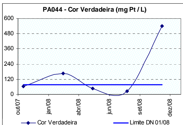
Figura 10.52: Ocorrência de cor verdadeira no Córrego Salobro a jusante do município de Pompéu (PA044) no período de monitoramento.
