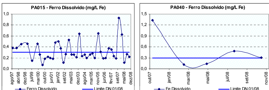
Figura 10.42: Ocorrência de ferro dissolvido no rio Lambari próximo de sua foz no rio Pará (PA015) e no rio Lambari no município de Pedra do Indaiá (PA040) no período de monitoramento.
