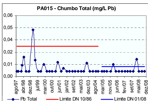
Figura 10.44: Ocorrência de chumbo total no rio Lambari próximo de sua foz no rio Pará (PA015), no período de monitoramento.
