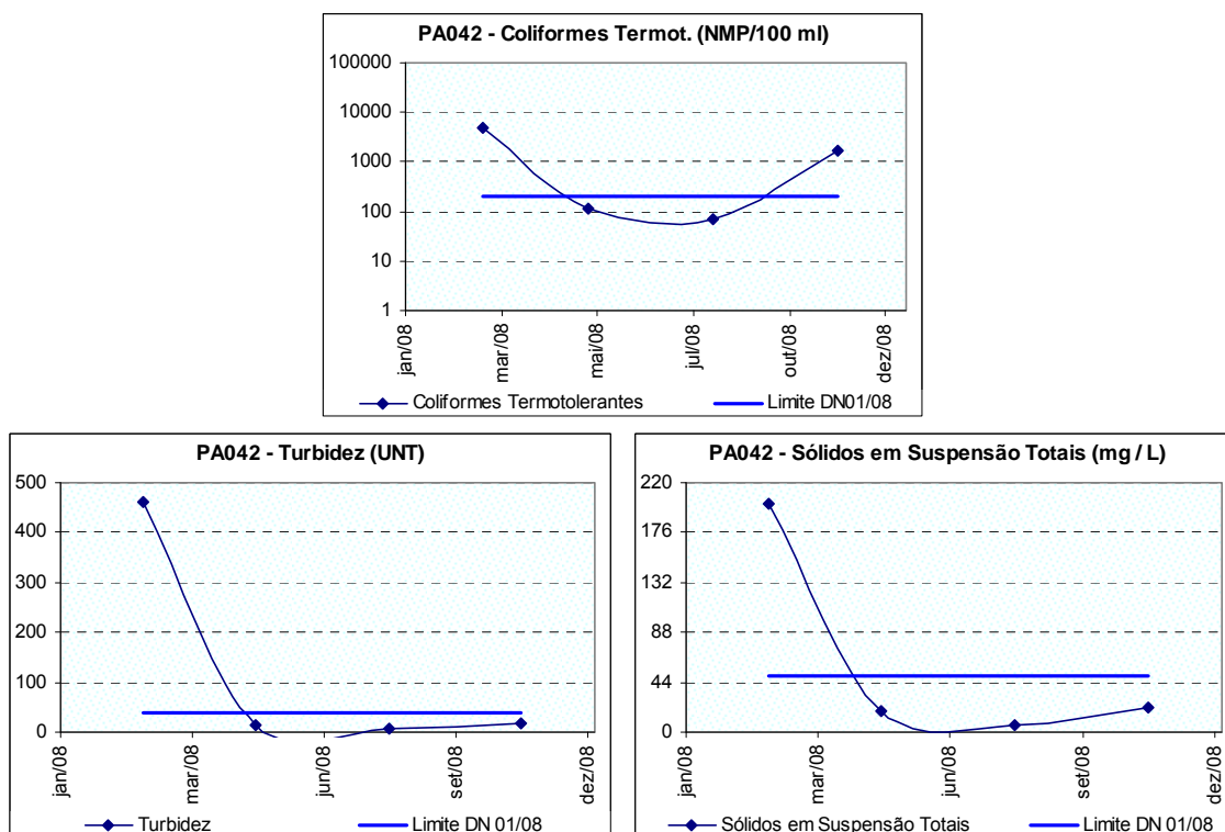
Figura 10.49: Ocorrência de coliformes termotolerantes, turbidez e sólidos em suspensão totais no rio do Peixe na localidade de rio do Peixe (PA042) no período de monitoramento.
