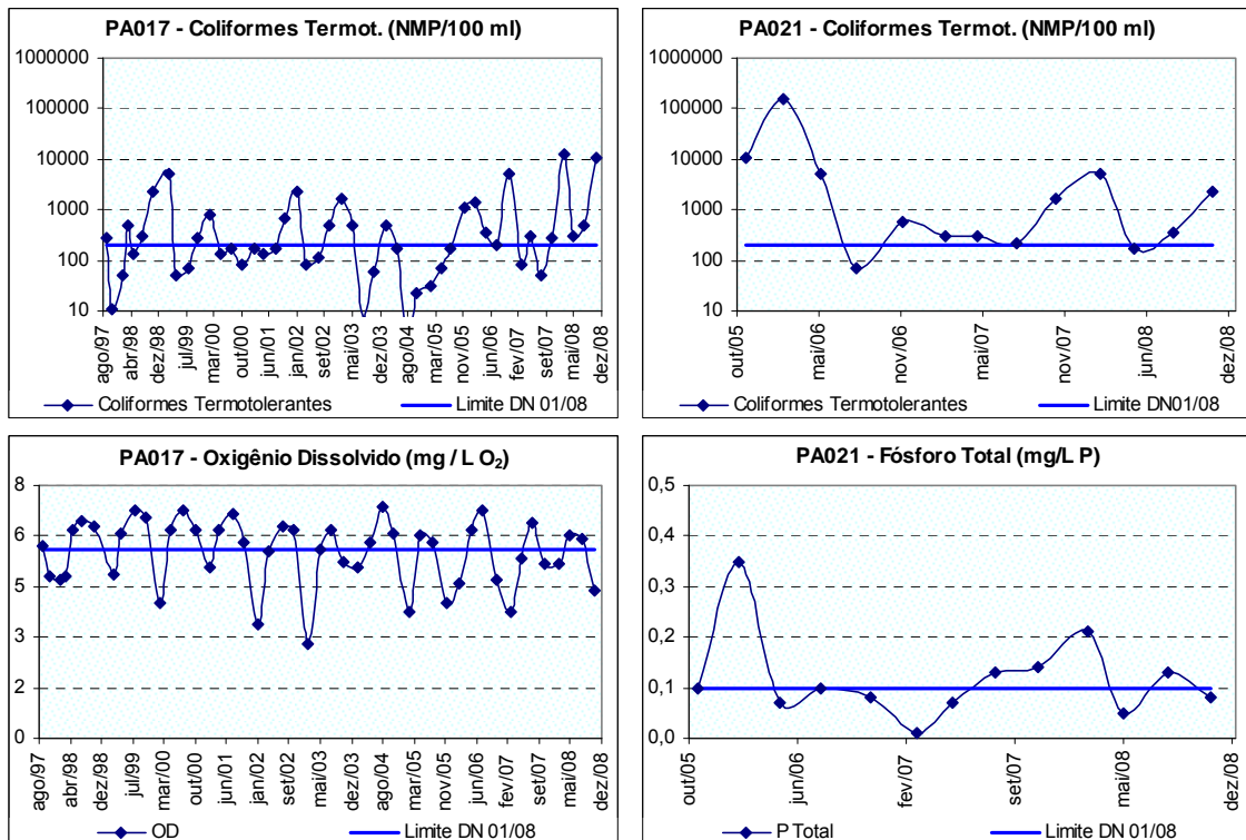
Figura 10.53: Ocorrências de coliformes termotolerantes e OD no rio do Picão próximo de sua foz no rio Pará (PA017) e coliformes termotolerantes e fósforo total a jusante da cidade de Bom Despacho (PA021) no período de monitoramento.
