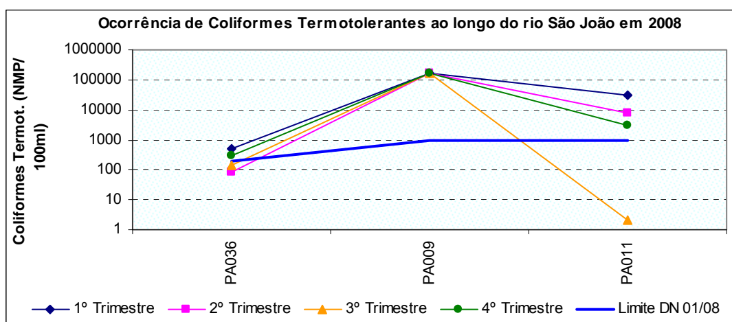
Figura 10.31: Ocorrência de coliformes termotolerantes ao longo do rio São João, no ano de 2008.
