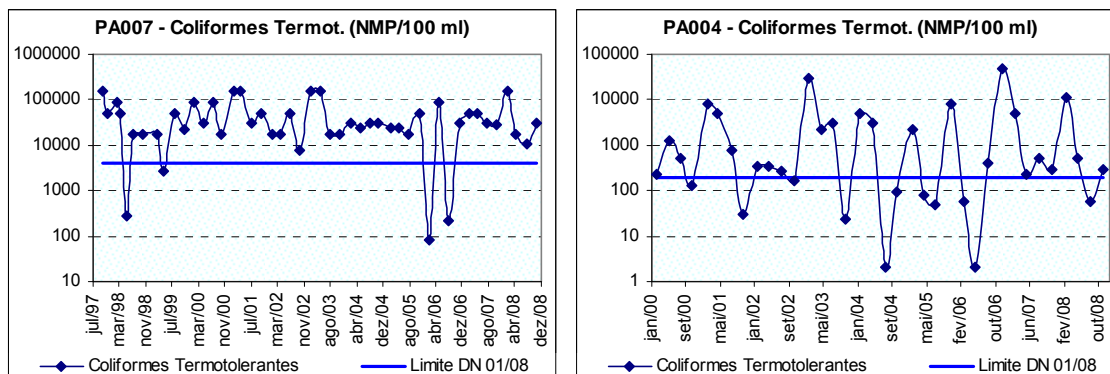
Figura 10.16: Ocorrência de coliformes termotolerantes no rio Itapecerica a jusante da cidade de Divinópolis (PA007) e no rio Itapecerica a montante de Divinópolis (PA004) no período de monitoramento.
