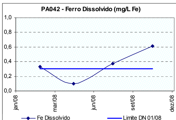
Figura 10.50: Ocorrência de ferro dissolvido no rio do Peixe na localidade de rio do Peixe (PA042) no período de monitoramento.
