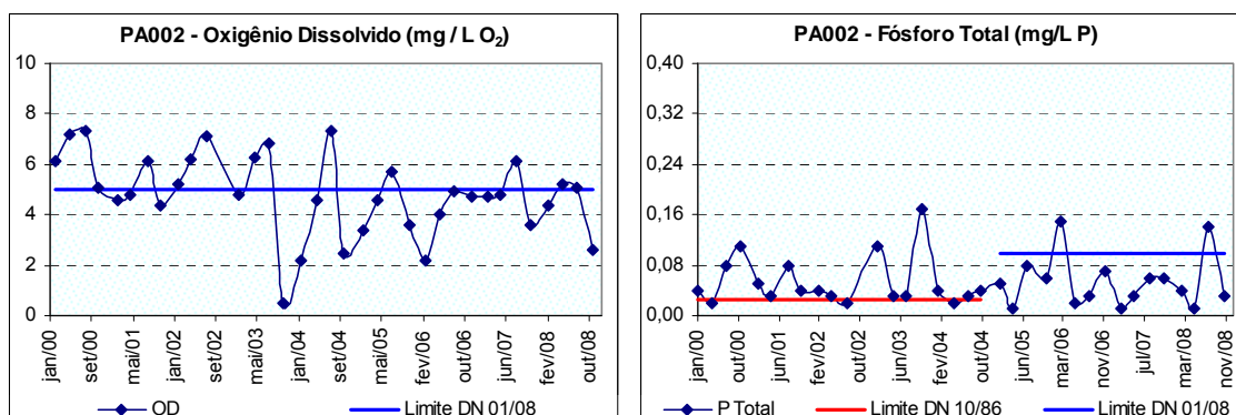
Figura 10.14: Ocorrência de oxigênio dissolvido e fósforo total na estação de amostragem no ribeirão Paiol a jusante da cidade de Carmópolis de Minas (PA002) no período de 2000 a 2008.
