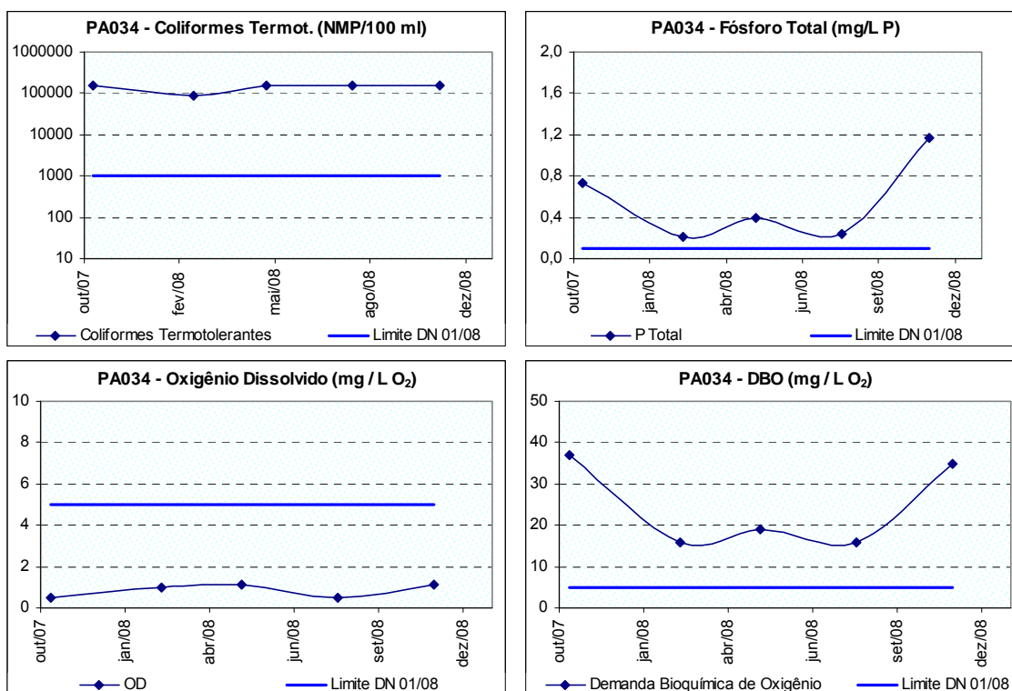
Figura 10.22: Ocorrências de coliformes termotolerantes, fósforo total, OD e DBO no córrego do Pinto ou Buriti a jusante do município de São Gonçalo do Pará (PA034) no período de monitoramento.
