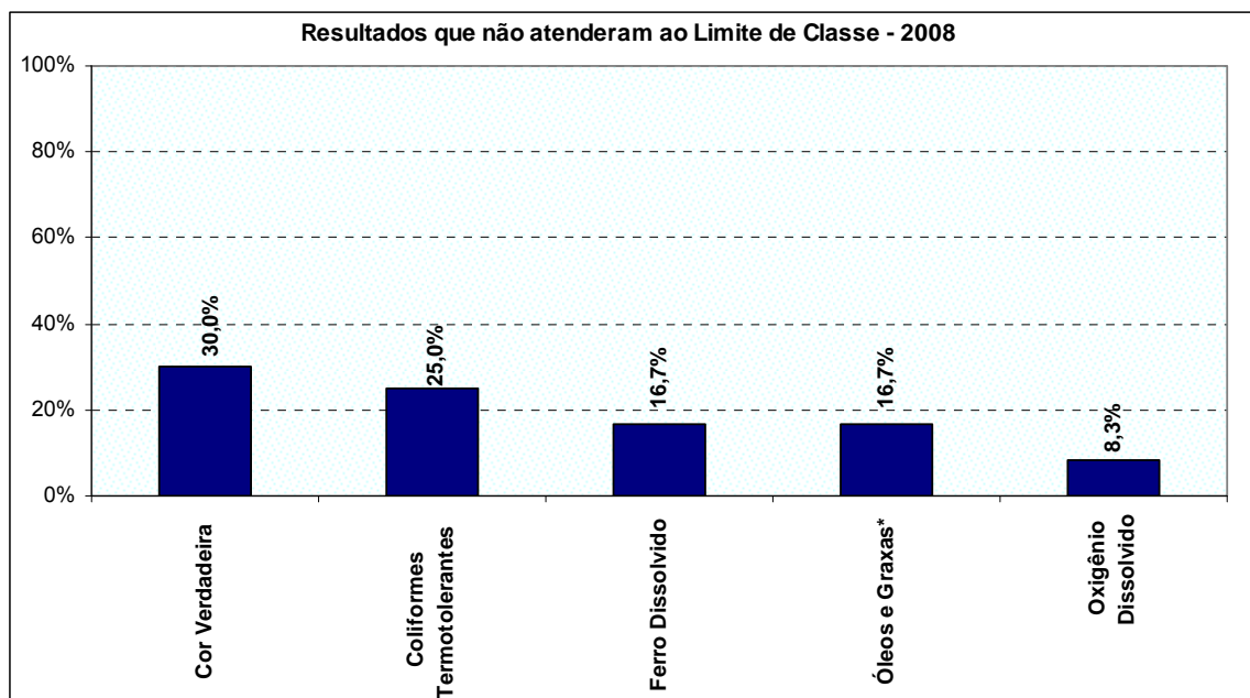
Figura 8.39: Frequência da ocorrência de parâmetros fora dos limites estabelecidos na legislação em 2008 – UPRH PA1.
