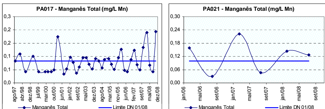
Figura 10.54: Ocorrência de manganês total no rio Picão próximo de sua foz no rio Pará (PA017) e a jusante da cidade de Bom Despacho (PA021) no período de monitoramento.
