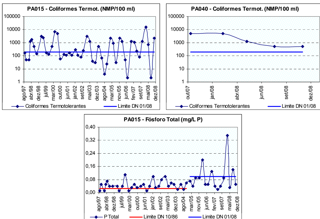
Figura 10.40: Ocorrência de coliformes termotolerantes e fósforo total no rio Lambari próximo de sua foz no rio Pará (PA015) e coliformes termotolerantes no rio Lambari no município de Pedra do Indaiá (PA040), no período de monitoramento.
