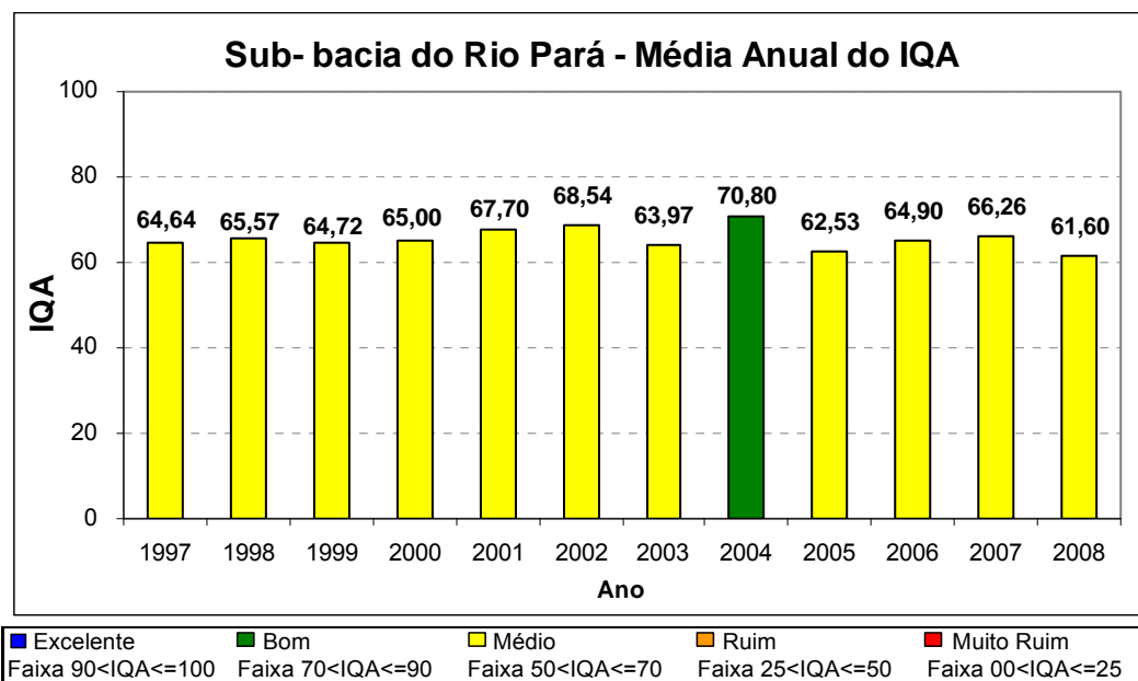
Figura 10.1: Evolução temporal da média anual do IQA na sub-bacia do rio Pará.
