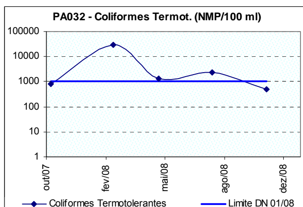
Figura 10.21: Ocorrência de coliformes termotolerantes no ribeirão Boa Vista a jusante do município de Carmo da Mata (PA032) no período de monitoramento.
