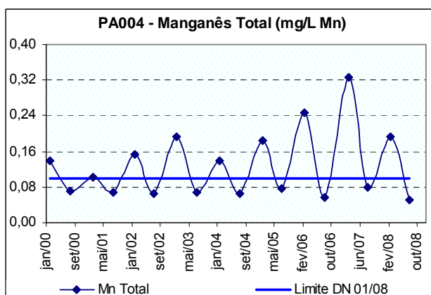
Figura 10.20: Ocorrência de manganês total no rio Itapecerica a montante da cidade de Divinópolis (PA004), no período de 2000 a 2008.
