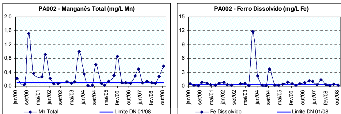
Figura 10.15: Ocorrência de manganês total e ferro dissolvido na estação de amostragem no ribeirão Paiol a jusante da cidade de Carmópolis de Minas (PA002) no período de 2000 a 2008.
