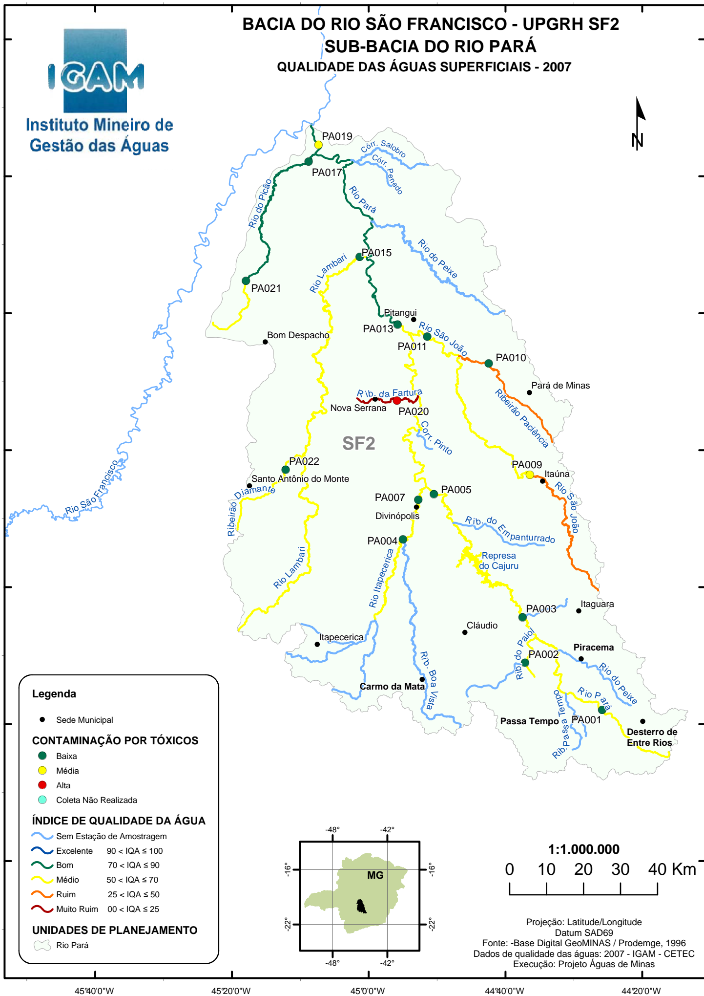
Mapa 9.7: Qualidade das águas superficiais da sub-bacia do rio Pará em 2007 – UPGRH SF2.
