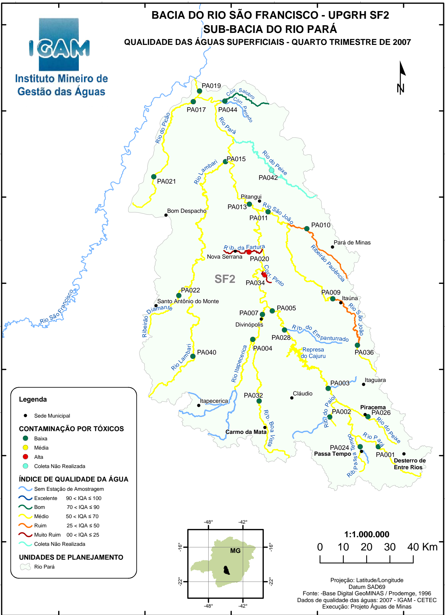
Mapa 9.6: Qualidade das águas superficiais da sub-bacia do rio Pará no quarto trimestre de 2007 - UPGRH SF2.
