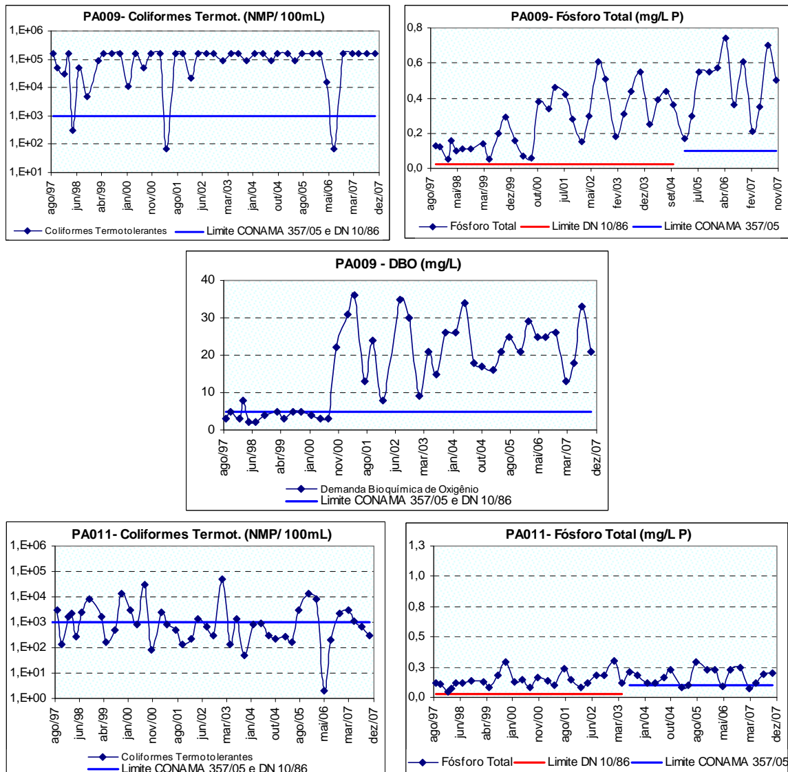
Figura 10.20: Ocorrência de coliformes termotolerantes , fósforo total e DBO no rio São João a jusante do município de Itaúna (PA009) e próximo á sua foz no rio Pará (PA011), no período de 1997 a 2007.
