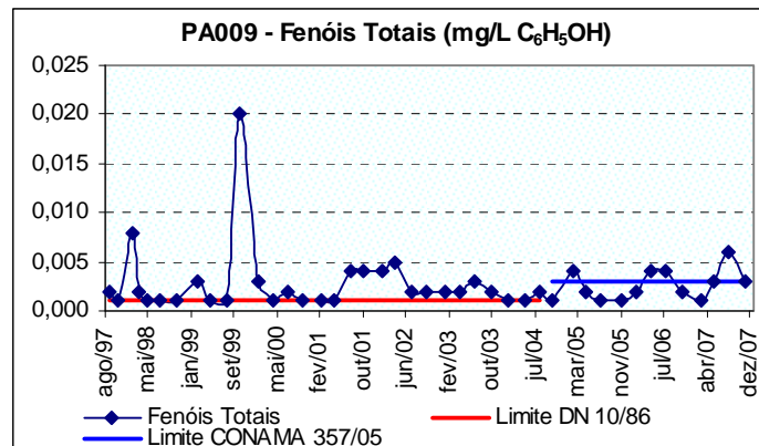
Figura 10.25: Ocorrência de fenóis totais no rio São João a jusante do município de Itaúna (PA009), no período de 1997 a 2007.
