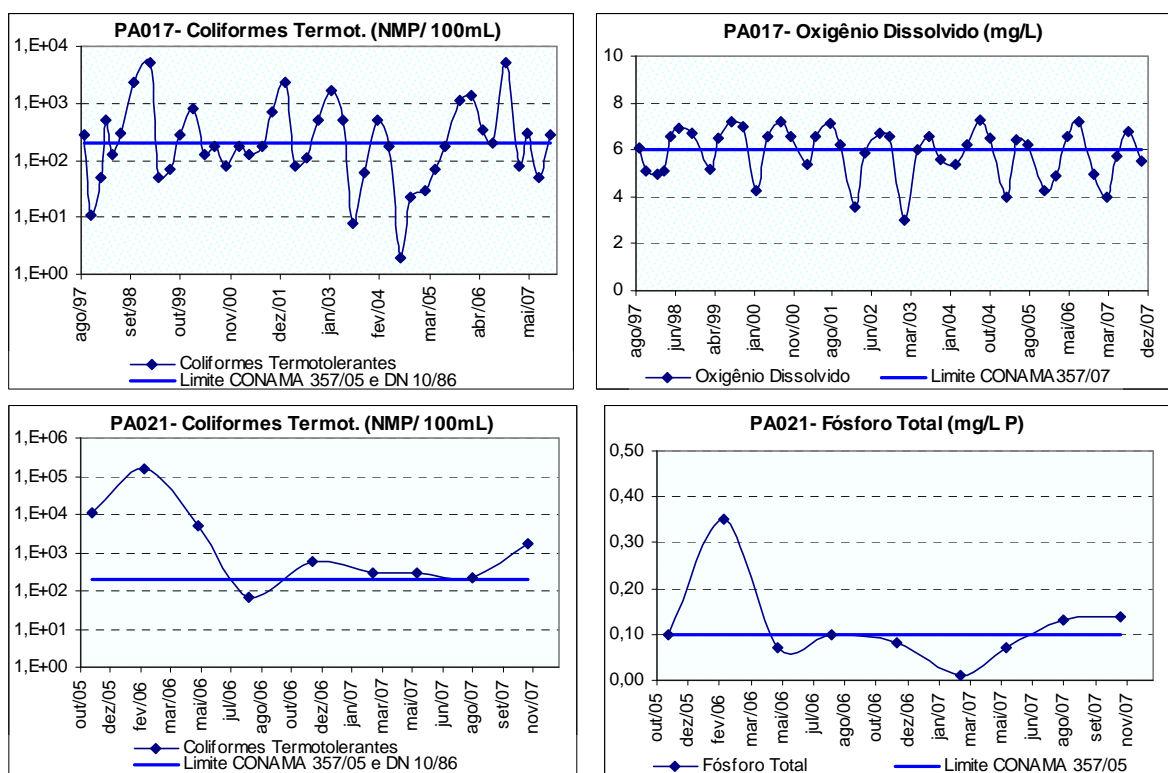
Figura 10.34: Ocorrências de coliformes termotolerantes, OD no rio do Picão próximo de sua foz no rio Pará (PA017) e coliformes termotolerantes e fósforo total a jusante da cidade de Bom Despacho (PA021), no período de monitoramento.
