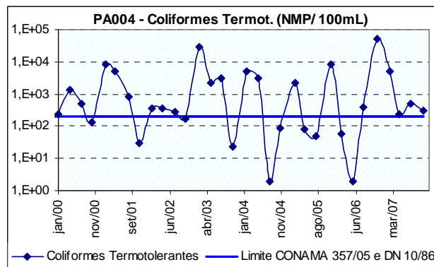
Figura 10.10: Ocorrência de coliformes termotolerantes no rio Itapecerica a montante de Divinópolis (PA004), no período de 2000 a 2007.
