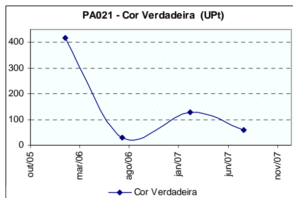
Figura 10.36: Ocorrência de cor verdadeira no rio Picão a jusante da cidade de Bom Despacho (PA021), no período de monitoramento.
