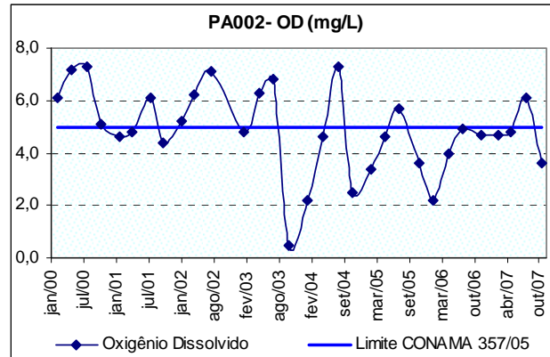
Figura 10.8: Ocorrência de oxigênio dissolvido na estação de amostragem no ribeirão Paiol a jusante da cidade de Carmópolis de Minas (PA002), no período de 2000 a 2007.
