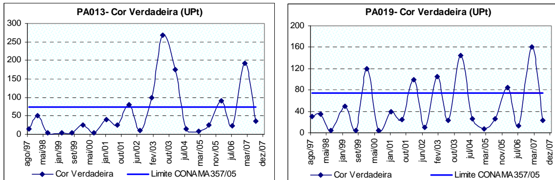
Figura 10.4 : Ocorrência de cor verdadeira no rio Pará na localidade de Velho da Taipa próximo ao município de Pitangui (PA013) e a montante de sua foz no rio São Francisco (PA019), no período de 1997 a 2007.
