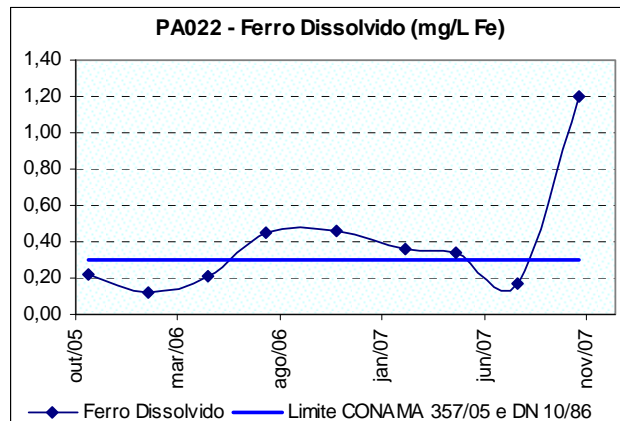
Figura 10.33: Ocorrência de ferro dissolvido no ribeirão Diamante a jusante da cidade de Santo Antônio do Monte (PA022), no período de 2005 a 2007.
