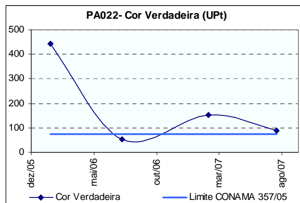
Figura 10.32: Alterações de cor verdadeira no ribeirão Diamante a jusante da cidade de Santo Antônio do Monte (PA022), no período de 2005 a 2007.
