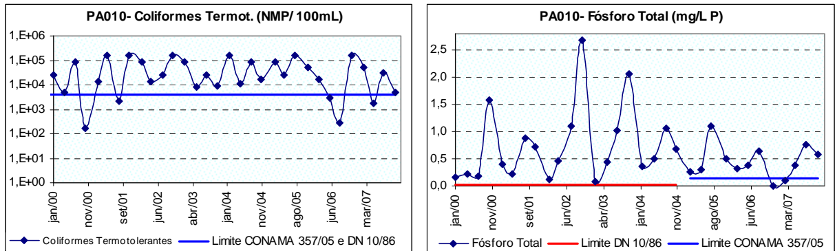
Figura 10.26: Ocorrência de coliformes termotolerantes e fósforo total no ribeirão Paciência a jusante de Pará de Minas (PA010), no período de 2000 a 2007.
