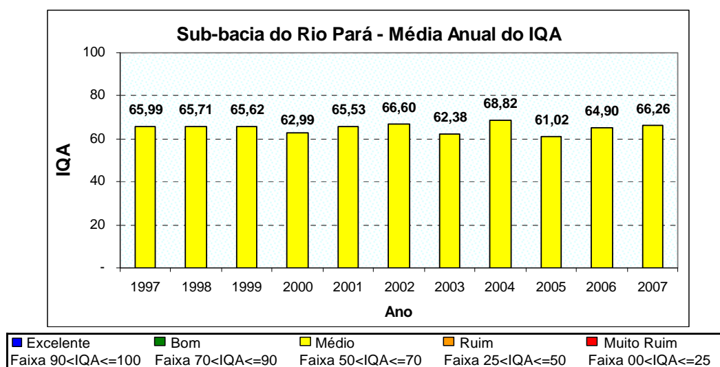
Figura 10.1: Evolução temporal da média anual do IQA na sub-bacia do Rio Pará.
