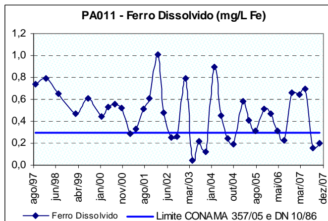
Figura 10.22: Ocorrência de ferro dissolvido no rio São João próximo à sua foz no rio Pará (PA011), no período de 1997 a 2007.
