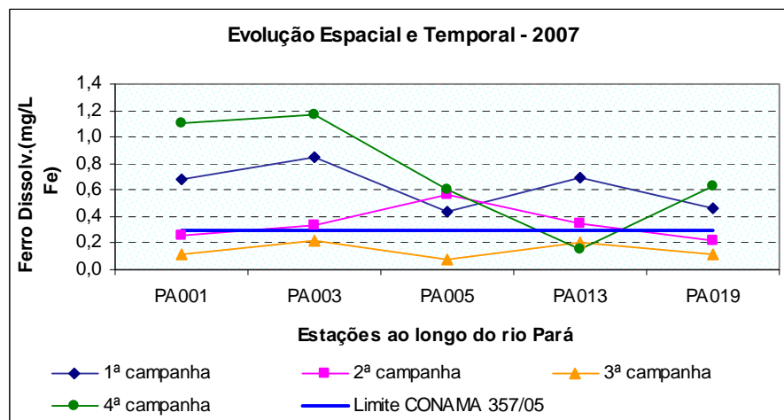
Figura 10.5: Ocorrência de ferro dissolvido ao longo do rio Pará, no ano de 2007.
