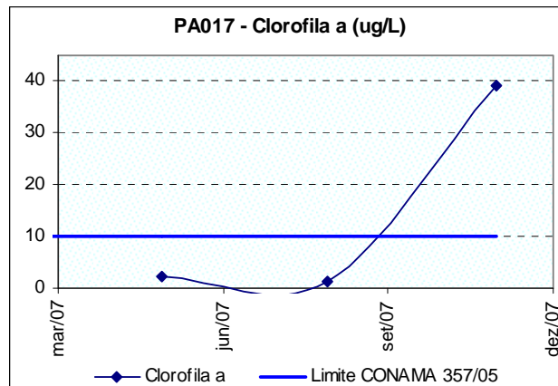
Figura 10.37: Ocorrência de clorofila-a no rio do Picão próximo de sua foz no rio Pará (PA017) no período de monitoramento.
