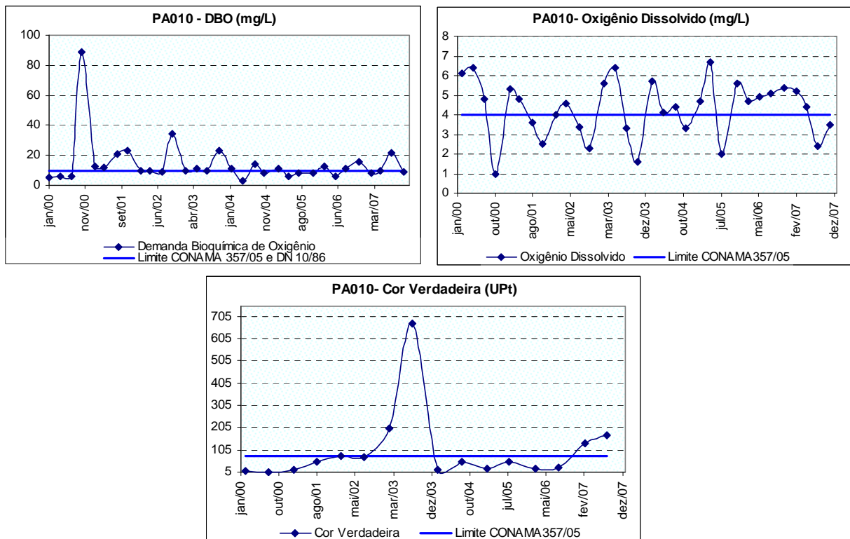
Figura 10.27: Alterações em DBO, oxigênio dissolvido e cor verdadeira no ribeirão Paciência a jusante de Pará de Minas (PA010), no período de 2000 a 2007.
