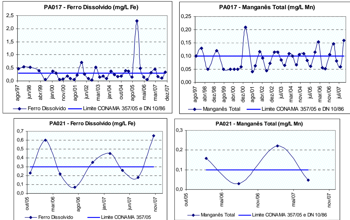
Figura 10.35: Ocorrência de manganês total e ferro dissolvido no rio Picão próximo de sua foz no rio Pará (PA017) e a jusante da cidade de Bom Despacho (PA021), no período de monitoramento.
