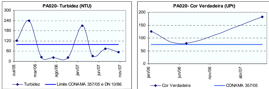
Figura 10.17: Ocorrência de turbidez e cor verdadeira no ribeirão da Fartura a montante de sua foz no rio Pará no município de Nova Serrana (PA020), no período de 2005 a 2007.
