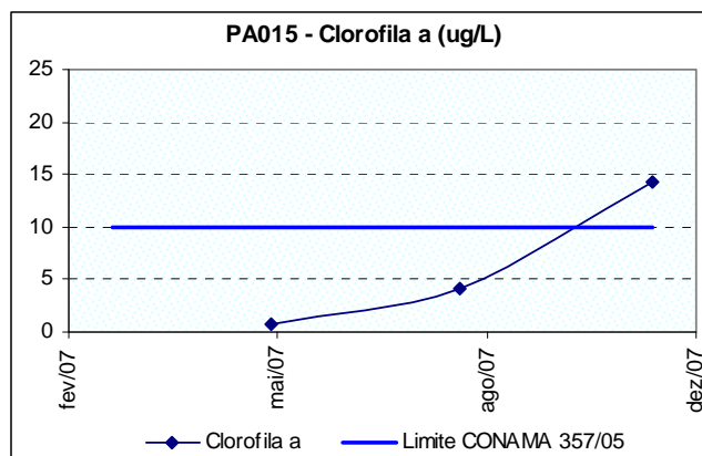
Figura 10.30: Ocorrência de clorofila-a no rio Lambari próximo de sua foz no rio Pará (PA015), no período de monitoramento.
