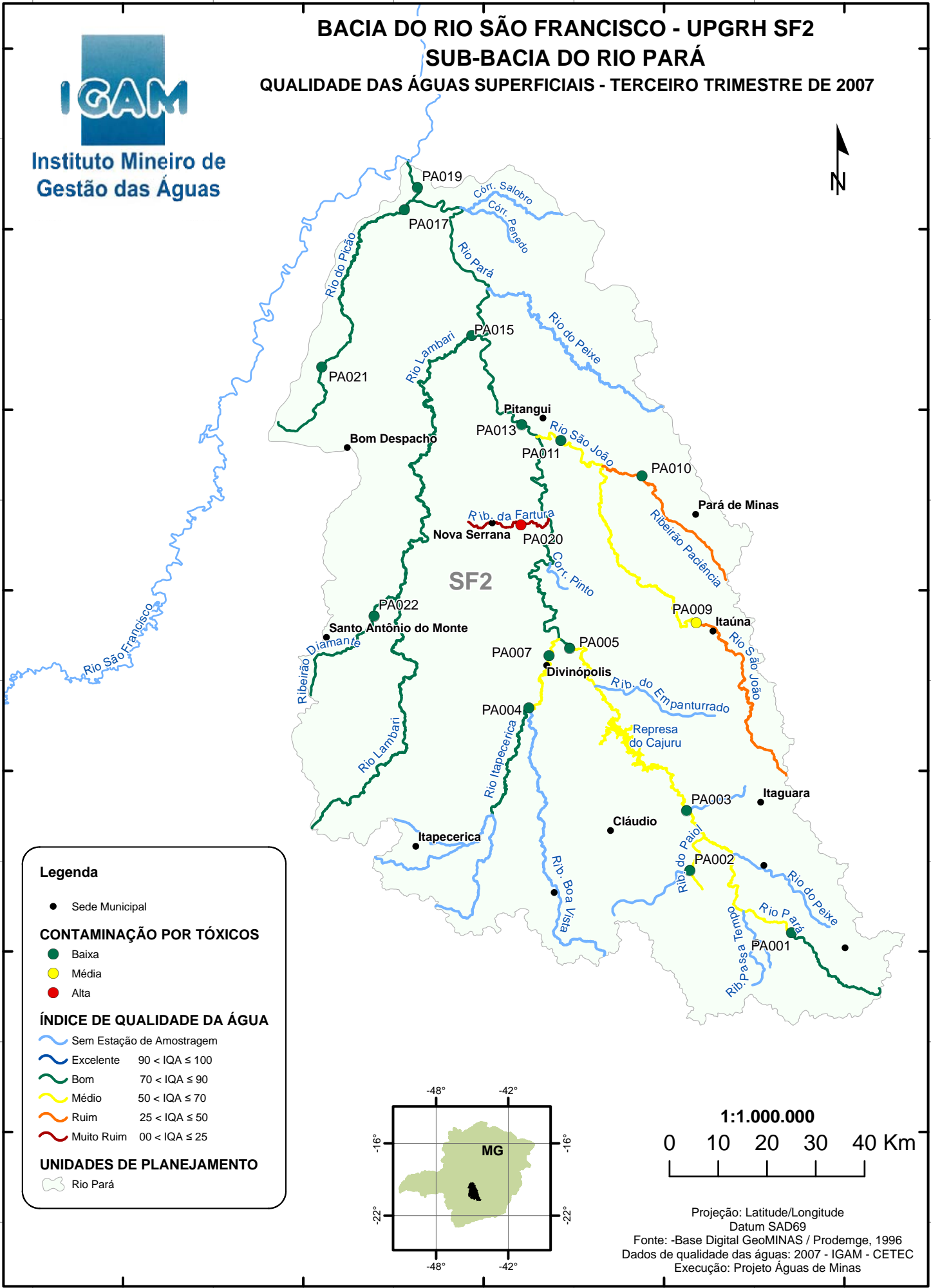
Mapa 9.5: Qualidade das águas superficiais da sub-bacia do rio Pará no terceiro trimestre de 2007- UPRGH SF2.
