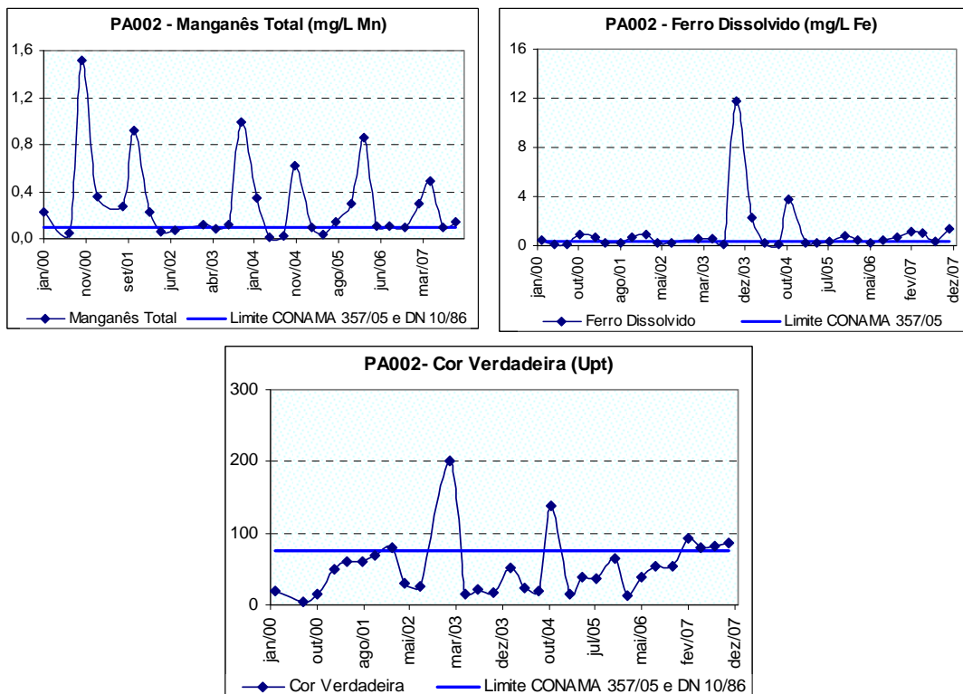
Figura 10.9: Ocorrência de manganês total, ferro dissolvido e cor verdadeira na estação de amostragem no ribeirão Paiol a jusante da cidade de Carmópolis de Minas (PA002), no período de 2000 a 2007.
