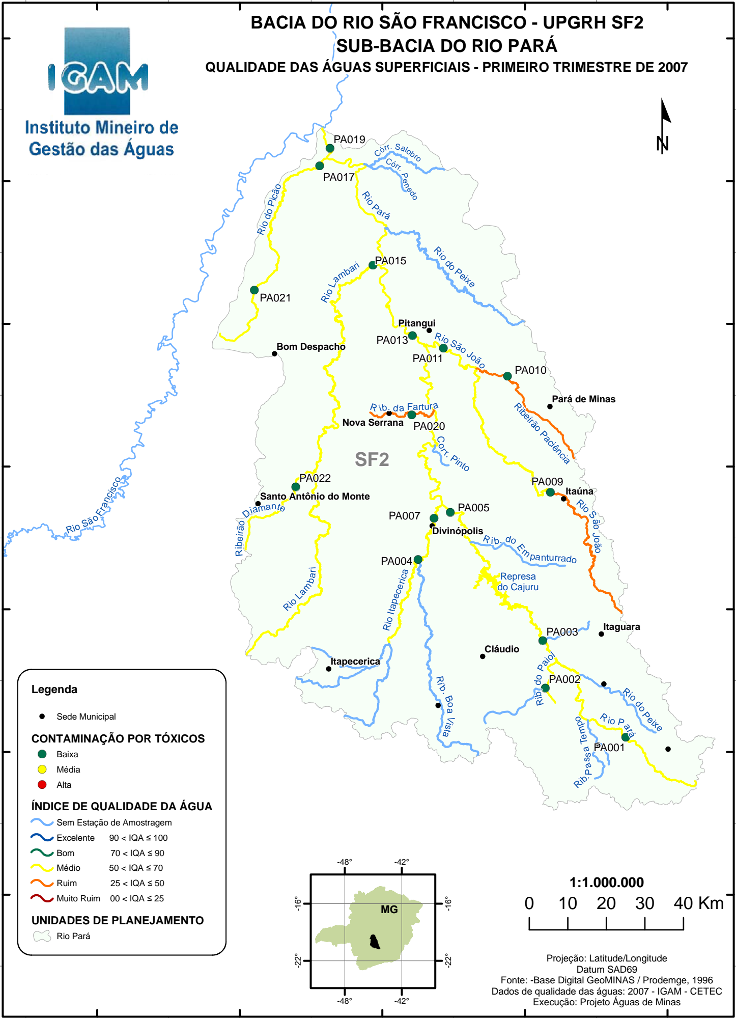
Mapa 9.3: Qualidade das águas superficiais da sub-bacia do rio Pará no primeiro trimestre de 2007 - UPGRH SF2.
