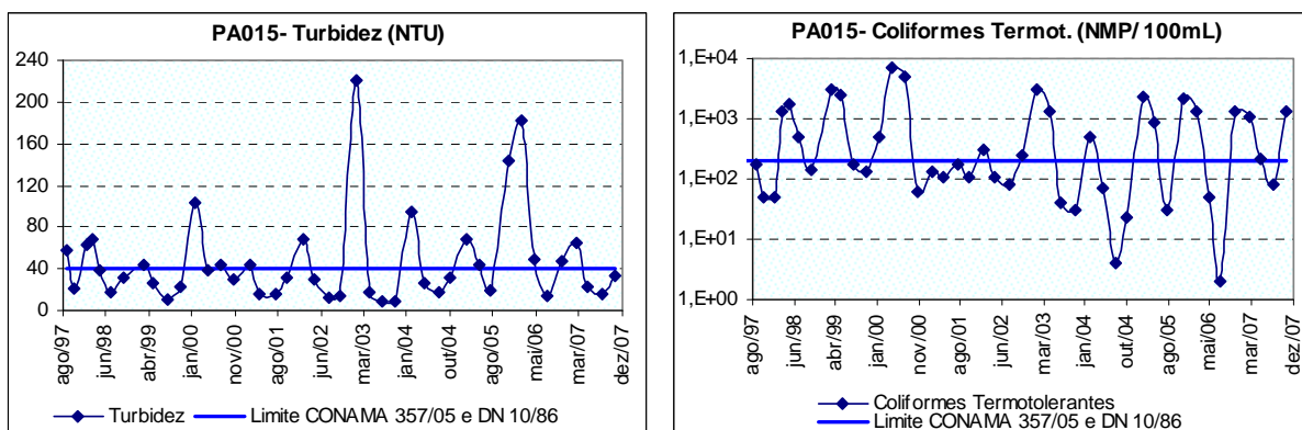
Figura 10.28: Ocorrência de turbidez e coliformes termotolerantes no rio Lambari próximo de sua foz no rio Pará (PA015), no período de 2000 a 2007.
