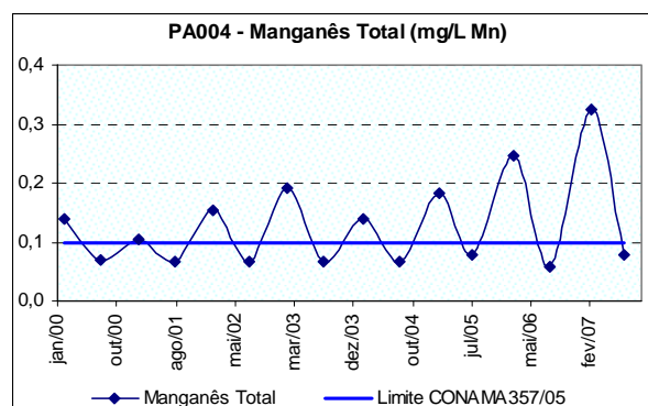
Figura 10.13: Ocorrência de manganês total no rio Itapecerica a montante da cidade de Divinópolis (PA004), no período de 2000 a 2007.
