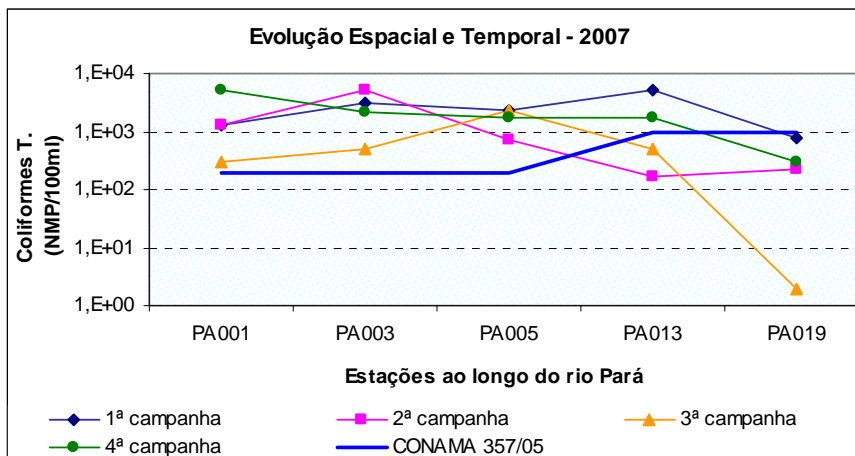
Figura 10.2: Ocorrência de coliformes termotolerantes ao longo do rio Pará, no ano de 2007.
