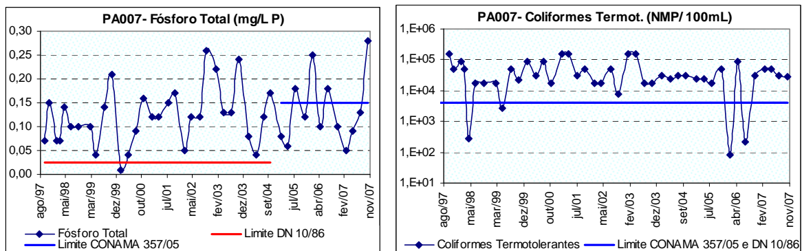
Figura 10.11: Ocorrência de fósforo total e coliformes termotolerantes no rio Itapecerica a jusante da cidade de Divinópolis (PA007), no período de 1997 a 2007.
