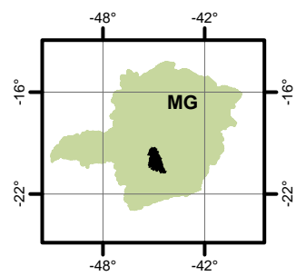
Mapa 9.7: Qualidade das águas superficiais da sub-bacia do rio Pará em 2007 – UPGRH SF2.
