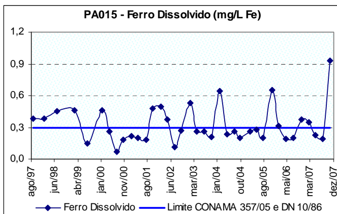
Figura 10.29: Ocorrência de ferro dissolvido no rio Lambari próximo de sua foz no rio Pará (PA015), no período de 1997 a 2007.
