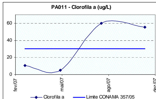
Figura 10.24: Ocorrência de clorofila-a no rio São João próximo à sua foz no rio Pará (PA011), no período de monitoramento.
