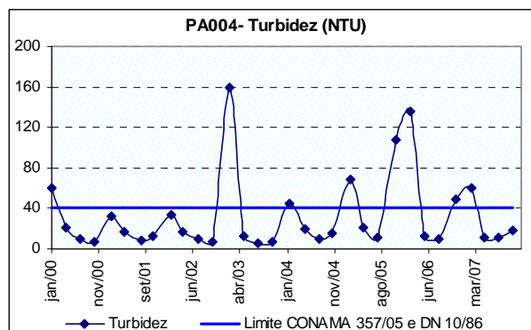
Figura 10.12: Ocorrência de turbidez no rio Itapecerica a montante de Divinópolis (PA004), no período de 2000 a 2007.
