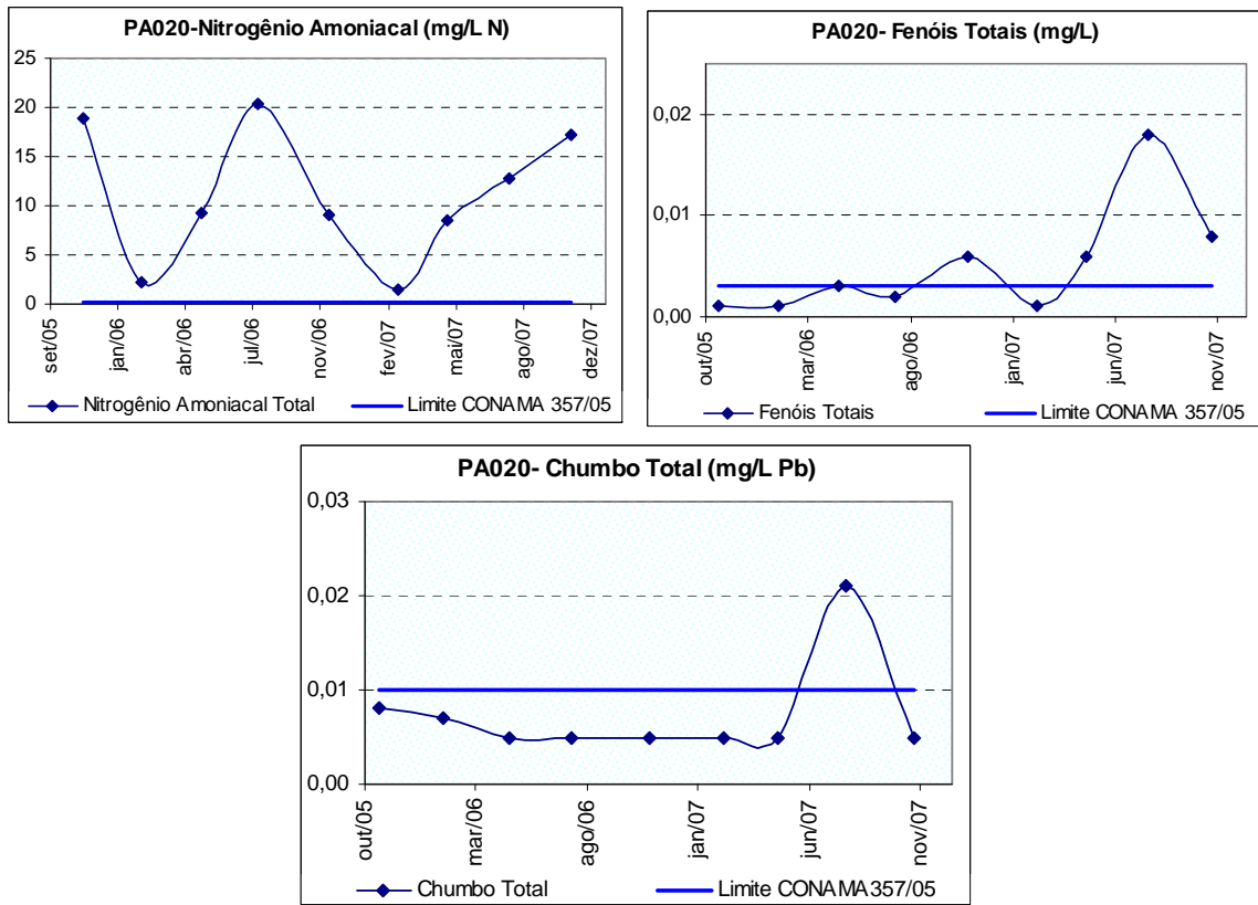
Figura 10.19: Ocorrência de nitrogênio amoniacoal, fenóis totais e chumbo total no ribeirão da Fartura a montante de sua foz no rio Pará no município de Nova Serrana (PA020), no período de 2005 a 2007.
