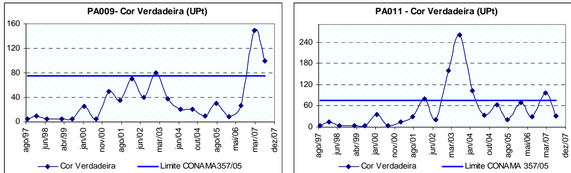
Figura 10.23: Ocorrência de cor verdadeira no rio São João a jusante do município de Itaúna (PA009) e próximo à sua foz no rio Pará (PA011), no período de 1997 a 2007.
