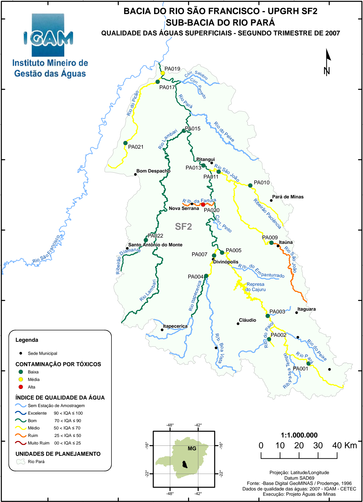
Mapa 9.4: Qualidade das águas superficiais da sub-bacia do rio Pará no segundo trimestre de 2007 - UPRGH SF2.
