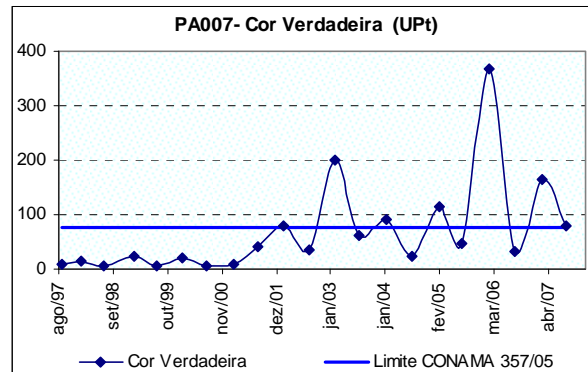
Figura 10.14: Ocorrência de cor verdadeira no rio Itapecerica a jusante da cidade de Divinópolis (PA007), no período de 2000 a 2007.
