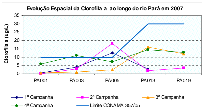
Figura 10.6: Ocorrência de clorofila-a ao longo do rio Pará, no ano de 2007.
