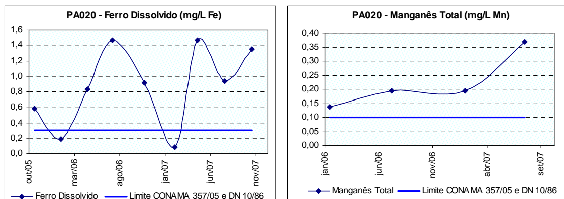
Figura 10.18: Ocorrência de ferro dissolvido e manganês total no ribeirão da Fartura a montante de sua foz no rio Pará no município de Nova Serrana (PA020), no período de monitoramento.
