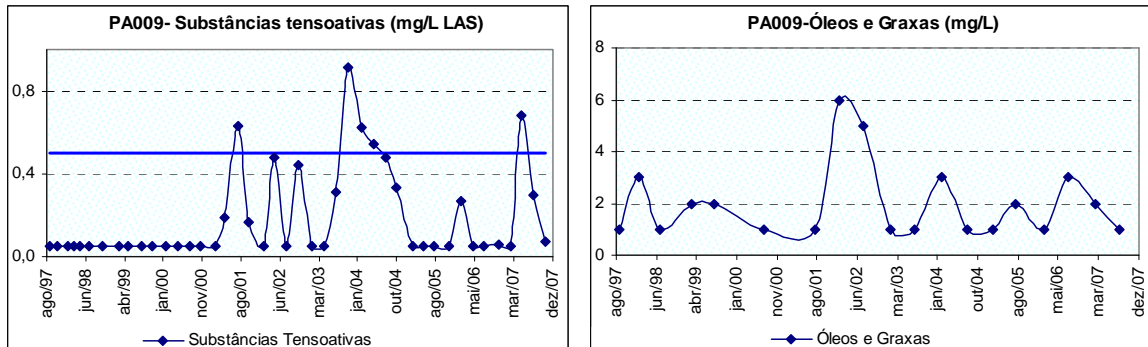
Figura 10.21: Alterações em substâncias tensoativas e óleos e no rio São João a jusante do município de Itaúna (PA009), no período de 1997 a 2007.
