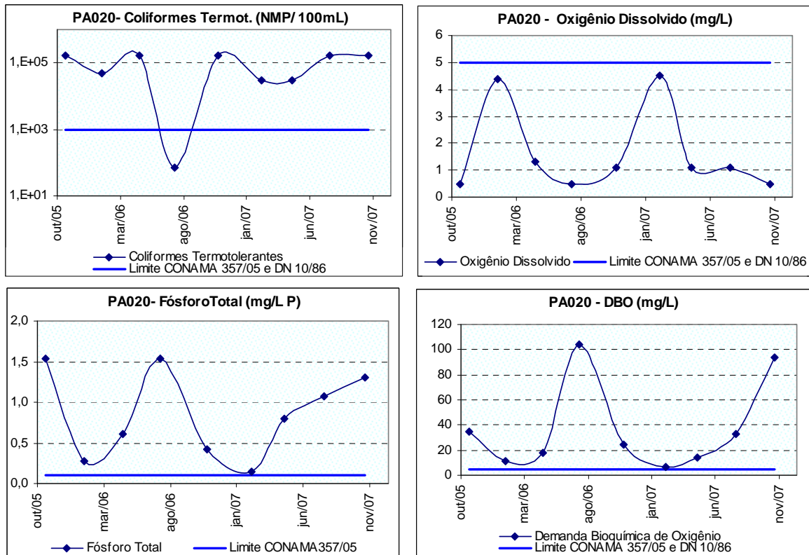
Figura 10.15: Ocorrência de coliformes termotolerantes, OD, fósforo total e DBO no ribeirão da Fartura a montante de sua foz no rio Pará, município de Nova Serrana (PA020) no período de 2005 a 2007.
