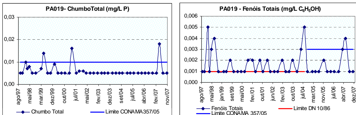
Figura 10.7: Ocorrência de chumbo total e fenóis totais na estação de amostragem no rio Pará a montante de sua foz no rio São Francisco (PA019), no período de amostragem.
