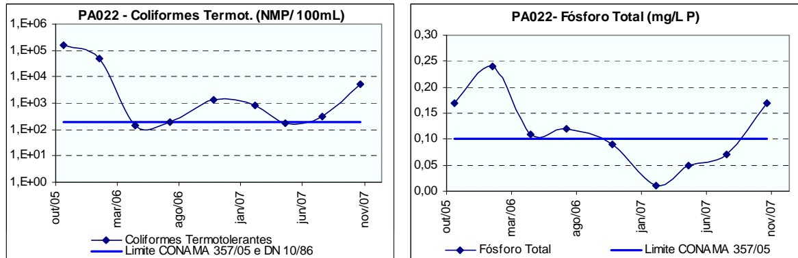
Figura 10.31: Ocorrência de coliformes termotolerantes e fósforo total no ribeirão Diamante a jusante da cidade de Santo Antônio do Monte (PA022), no período de 2005 a 2007.
