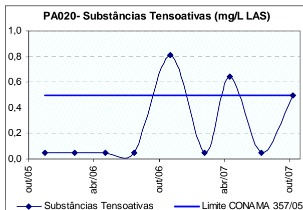
Figura 10.16: Ocorrência de substâncias tensoativas no ribeirão da Fartura a montante de sua foz no rio Pará, município de Nova Serrana (PA020) no período de 2005 a 2007.
