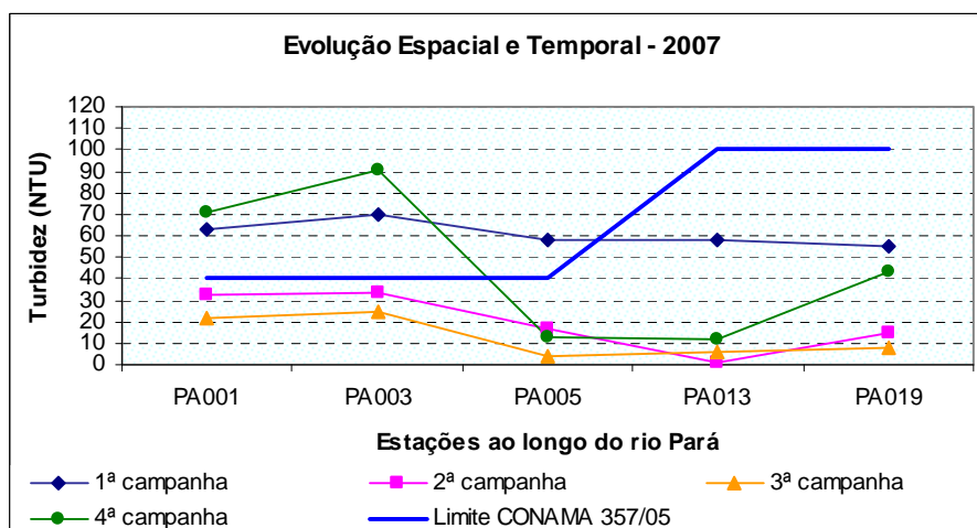
Figura 10.3: Ocorrência de turbidez ao longo do rio Pará, no ano de 2007.
