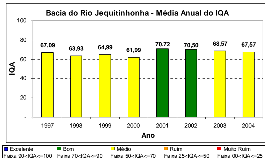
Figura 8.1: Evolução Temporal da Média Anual do IQA na Bacia do Rio Jequitinhonha.
