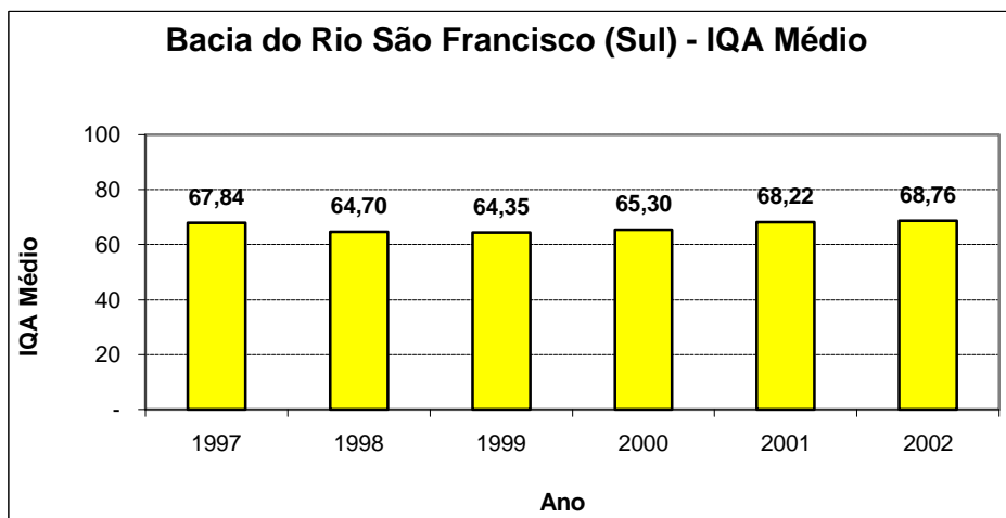
Figura 9.1: Evolução Temporal do IQA Médio na Sub-Bacia do Rio São Francisco - Sul
