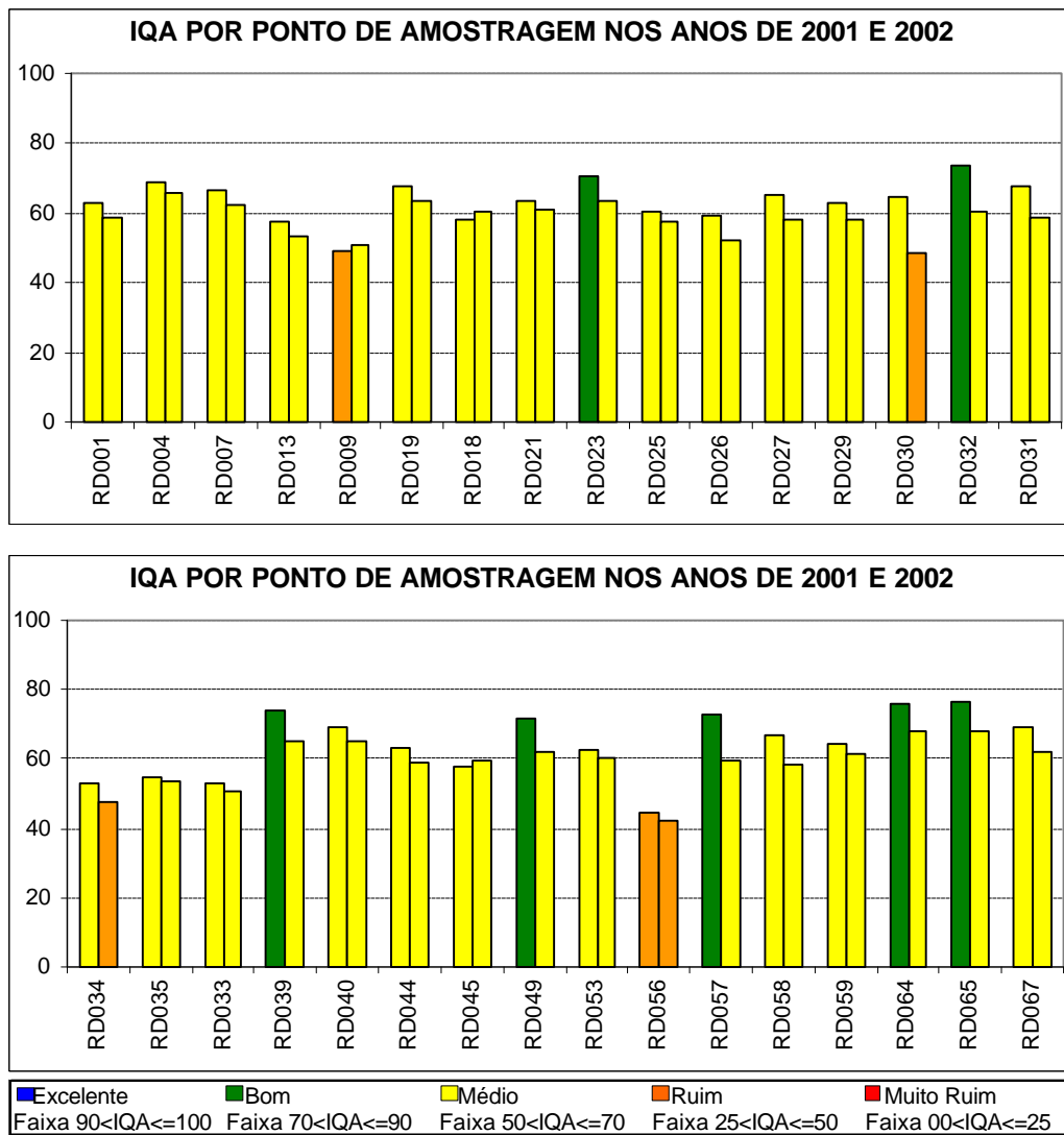
Figura 8.8: IQA médio dos anos 2001 e 2002, respectivamente, por estação de amostragem – UPGRHs DO1 a DO5
